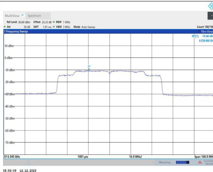
11AX80MIMO_Ant1_6545
