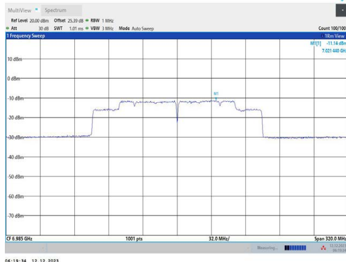
11AX160MIMO_Ant1_6985
