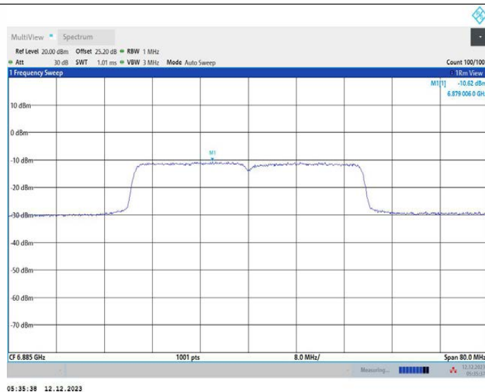
11AX40MIMO_Ant1_6885
