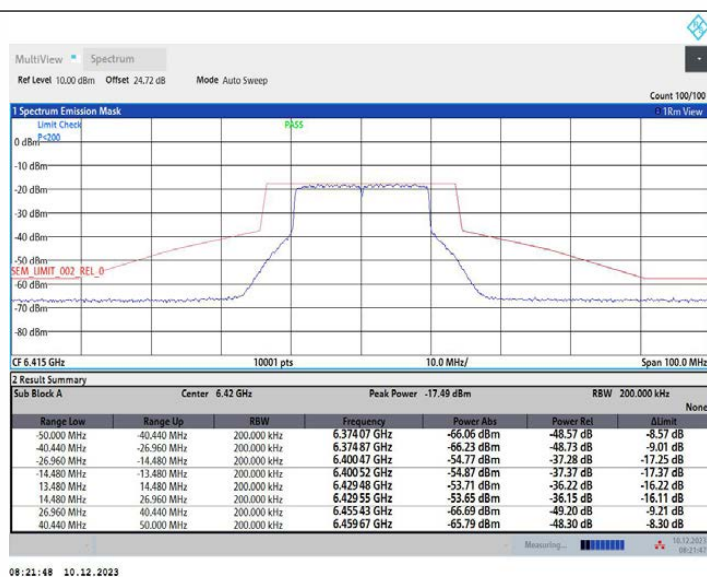
11AX20MIMO_Ant1_6415
