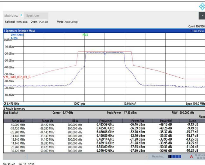
11AX20MIMO_Ant1_6475
