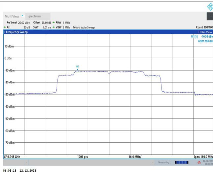
11AX80MIMO_Ant1_6945
