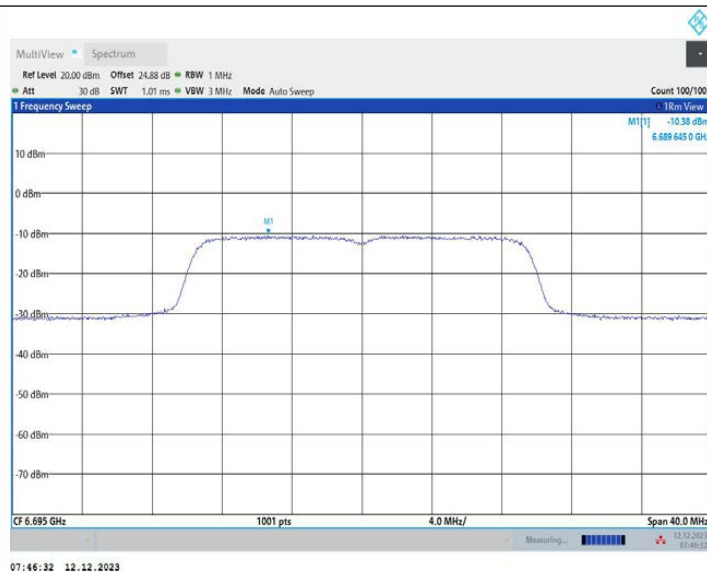
11AX20MIMO_Ant1_6695
