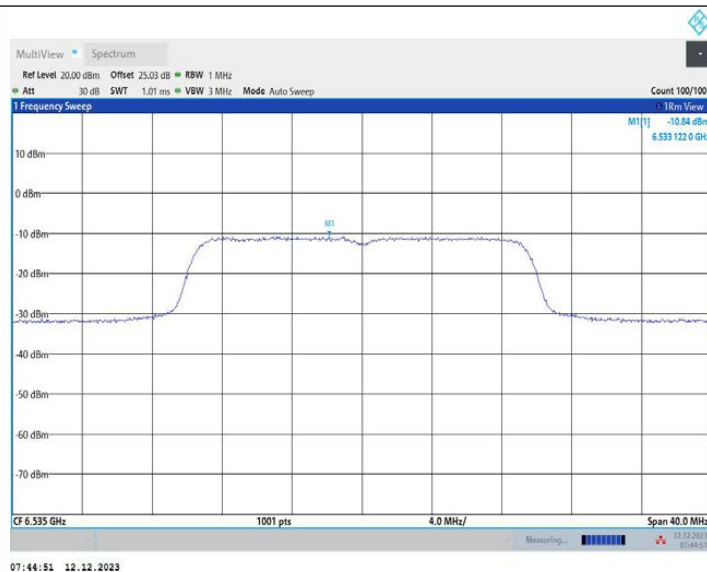
11AX20MIMO_Ant1_6535
