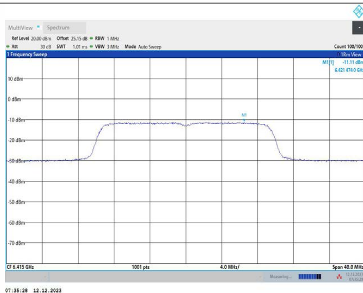
11AX20MIMO_Ant1_6415
