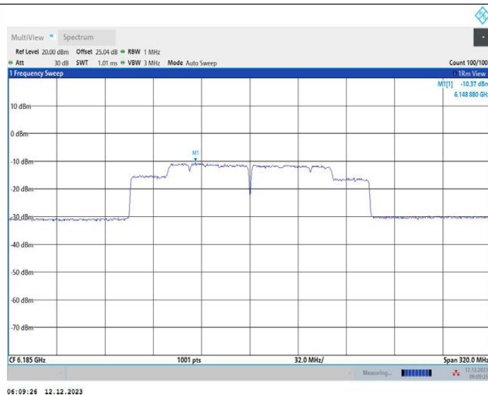
11AX160MIMO_Ant1_6185
