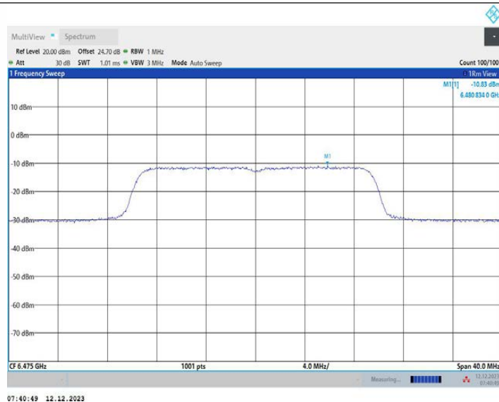
11AX20MIMO_Ant1_6475
