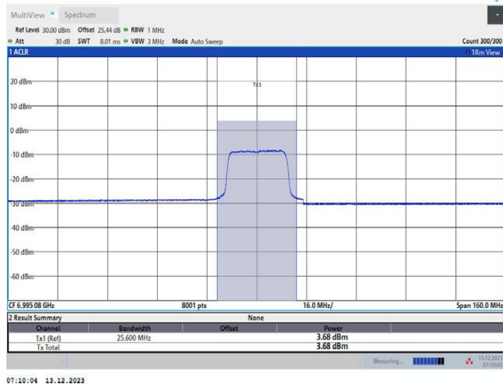
11AX80MIMO_Ant1_7025_484Tone_RU65
