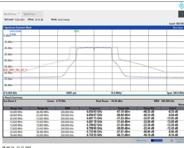
11AX20MIMO_Ant1_6695
