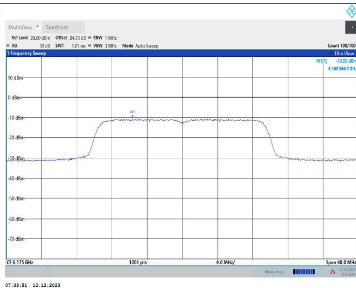
11AX20MIMO_Ant1_6175
