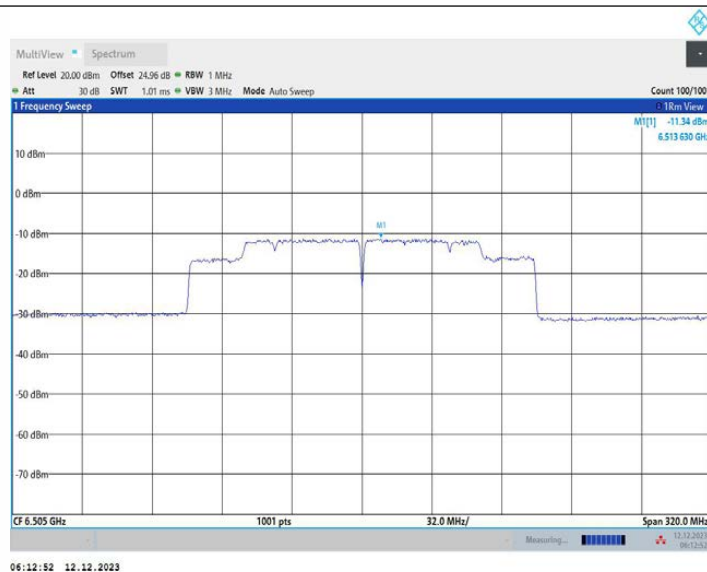
11AX160MIMO_Ant1_6505
