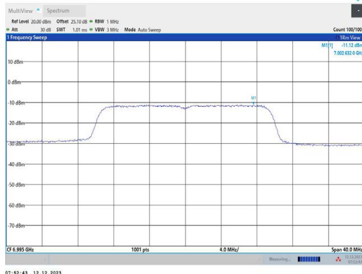
11AX20MIMO_Ant1_6995
