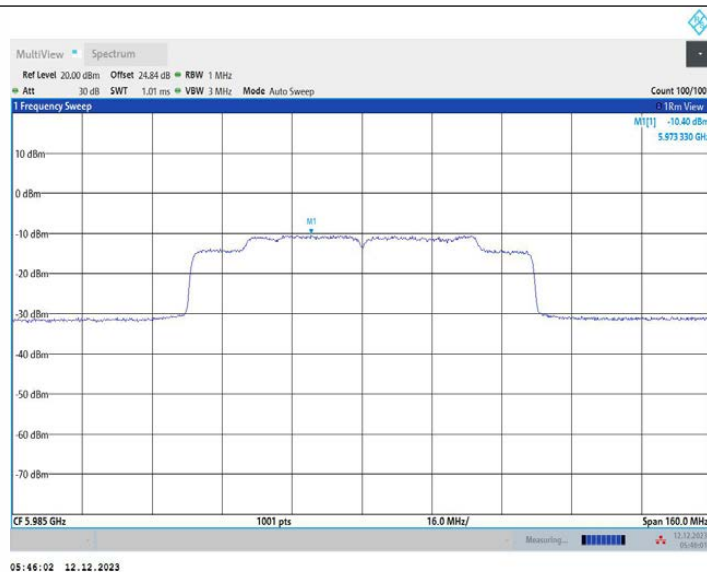
11AX80MIMO_Ant1_5985
