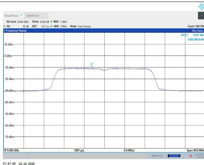
11AX20MIMO_Ant1_6855
