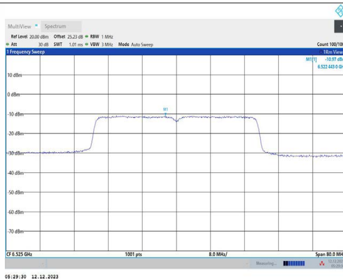
11AX40MIMO_Ant1_6525
