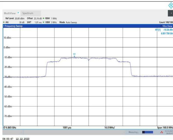
11AX80MIMO_Ant1_6865
