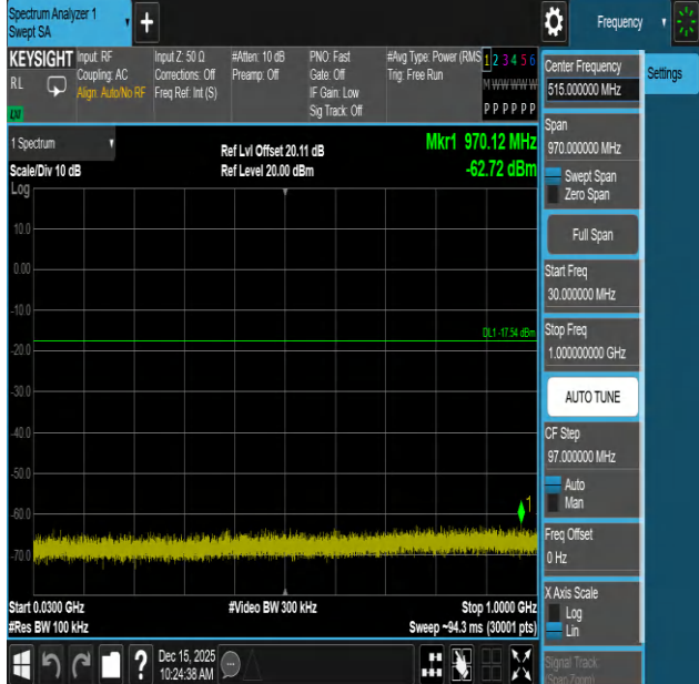
BLE 2M-2402-30~1000-PASS
