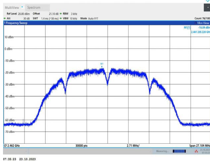
11B_Ant2_2462
