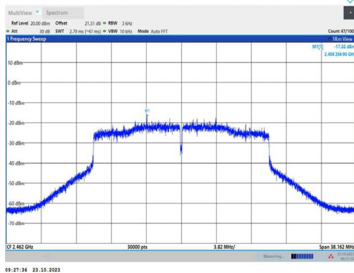
11AX20MIMO_Ant2_2462
