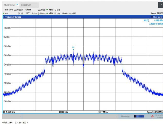
11G_Ant2_2462
