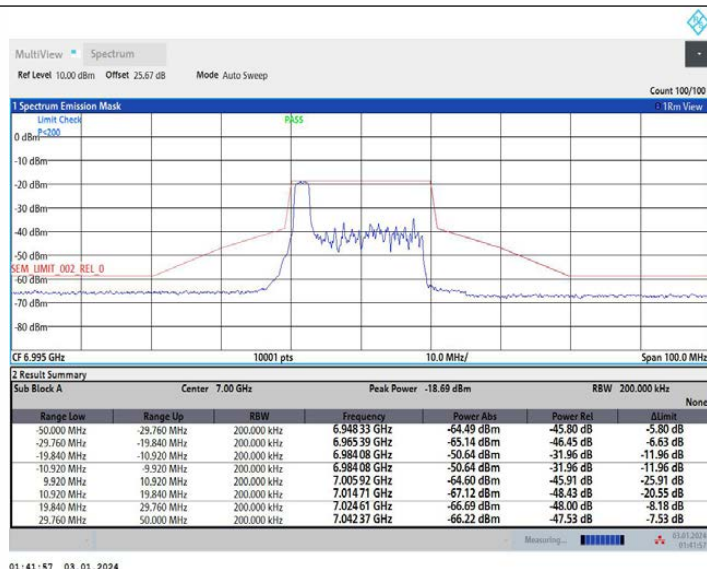
11AX20MIMO_Ant1_6995_52Tone_RU37
