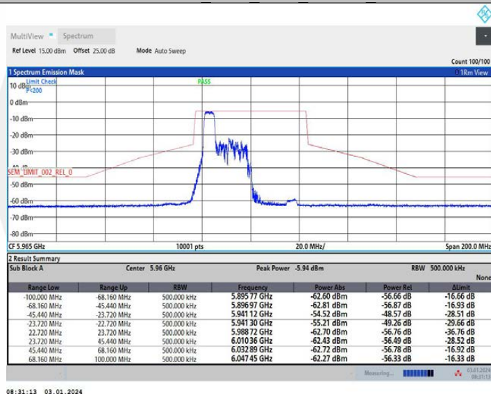
11AX40MIMO Ant1 5965 106Tone RU53
