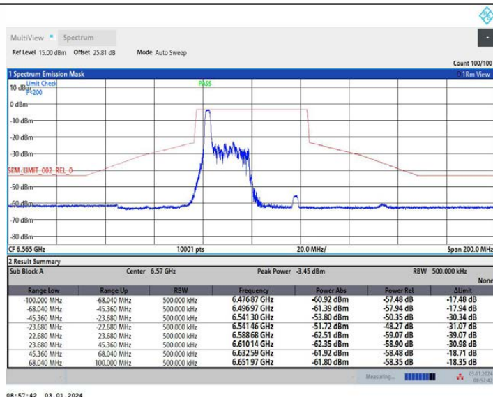
11AX40MIMO Ant1 6565 52Tone RU37
