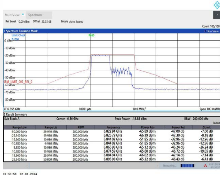
11AX20MIMO_Ant1_6875_26Tone_RU0
