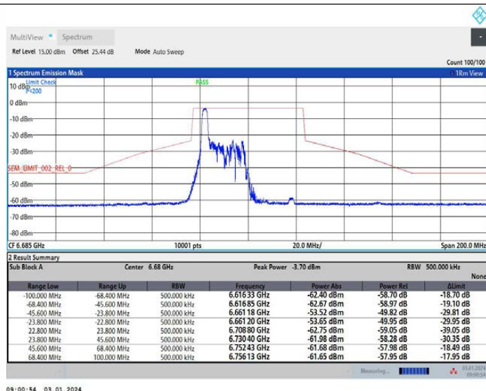
11AX40MIMO Ant1 6685 52Tone RU37
