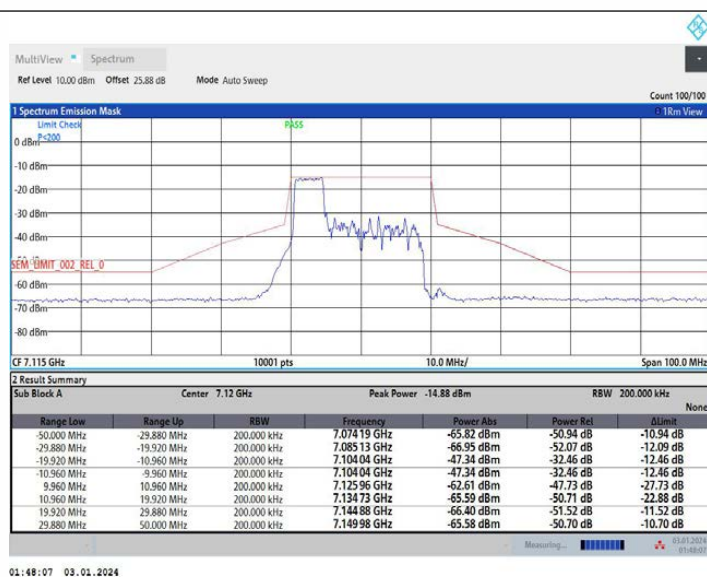
11AX20MIMO_Ant2_7115_106Tone_RU53
