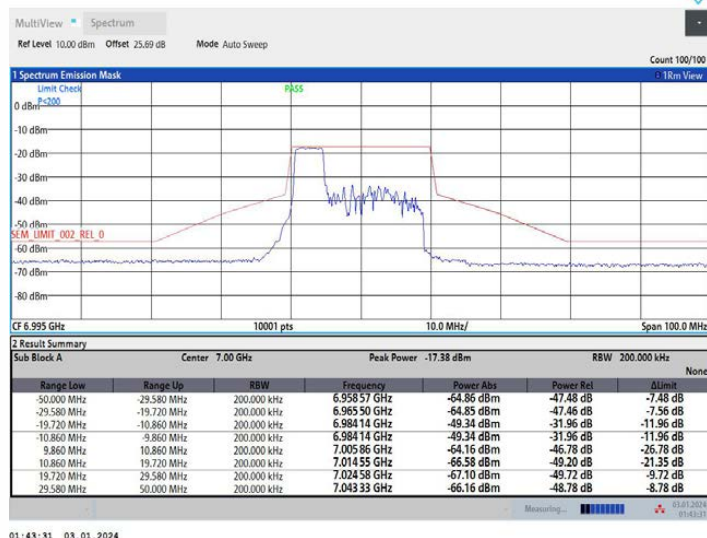
11AX20MIMO_Ant2_6995_106Tone_RU53
