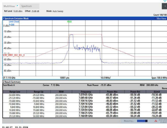
11AX20MIMO_Ant2_7115_52Tone_RU37
