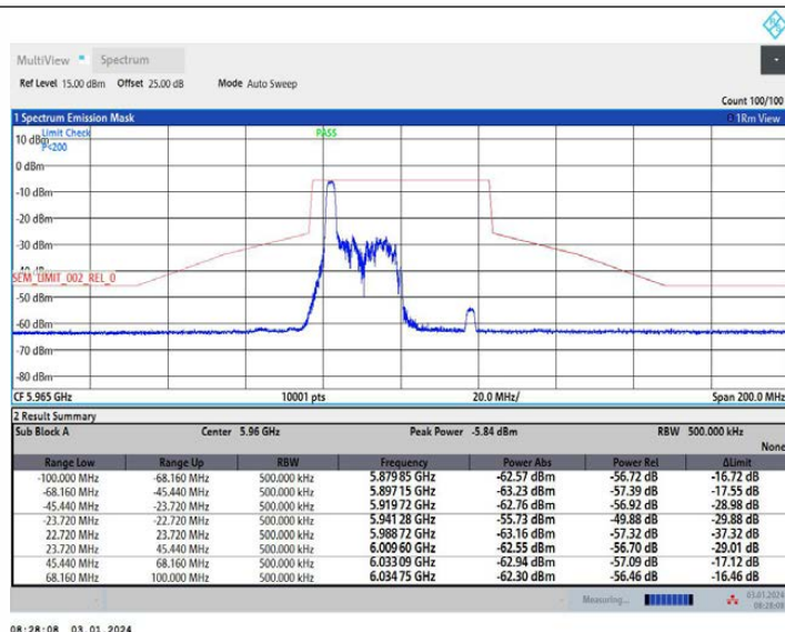
11AX40MIMO Ant1 5965 52Tone RU37
