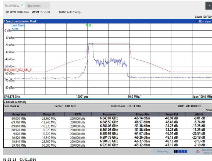
11AX20MIMO_Ant2_6875_52Tone_RU37
