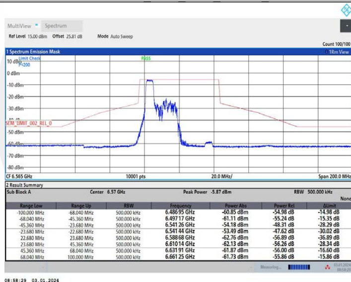
11AX40MIMO Ant1 6565 106Tone RU53
