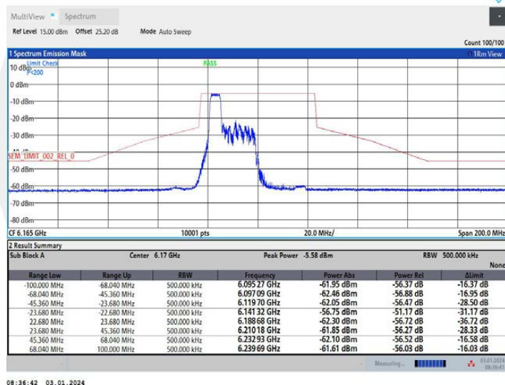
11AX40MIMO Ant1 6165 106Tone RU53
