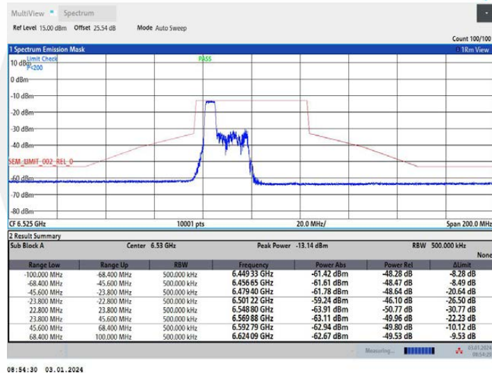
11AX40MIMO Ant1 6525 106Tone RU53
