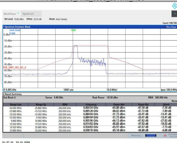
11AX20MIMO_Ant2_6895_52Tone_RU37
