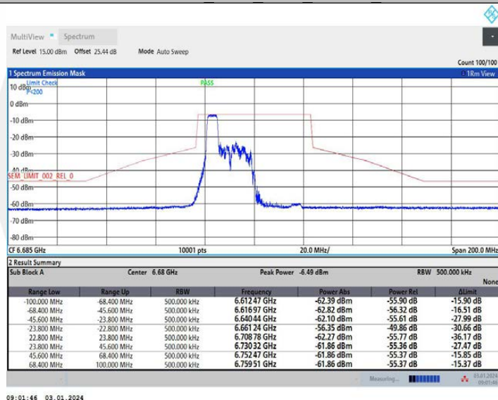
11AX40MIMO Ant1 6685 106Tone RU53
