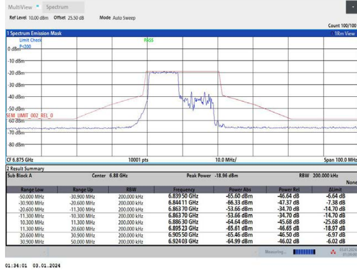
11AX20MIMO_Ant2_6875_26Tone_RU0
