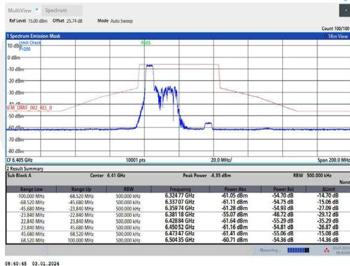
11AX40MIMO Ant1 6405 106Tone RU53
