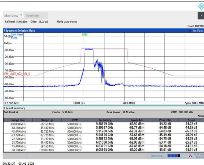
11AX40MIMO Ant1 5965 242Tone RU61
