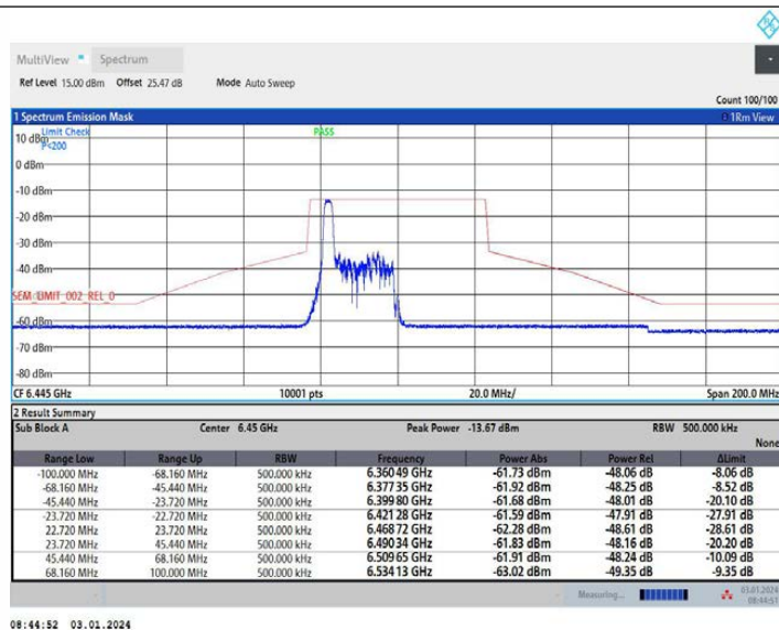
11AX40MIMO Ant1 6445 52Tone RU37
