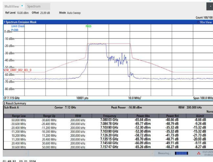
11AX20MIMO_Ant2_7115_26Tone_RU0
