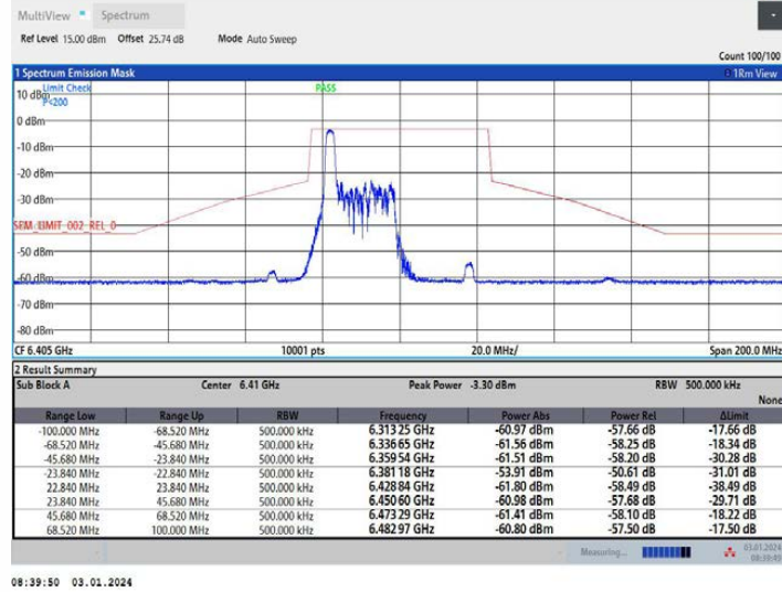
11AX40MIMO Ant1 6405 52Tone RU37
