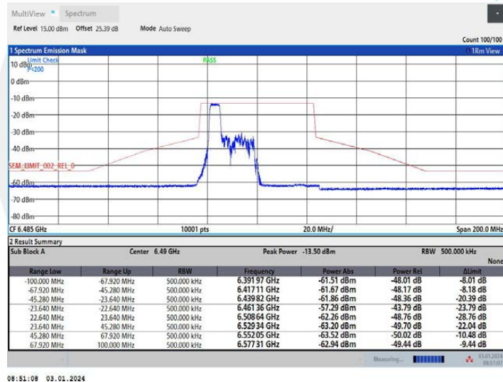
11AX40MIMO Ant1 6485 106Tone RU53
