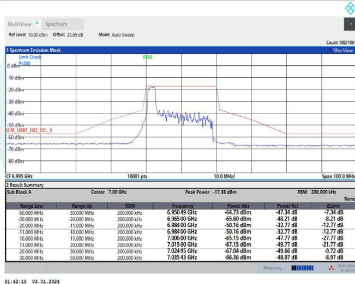
11AX20MIMO_Ant2_6995_52Tone_RU37
