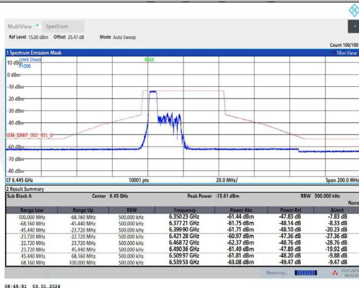
11AX40MIMO Ant1 6445 106Tone RU53
