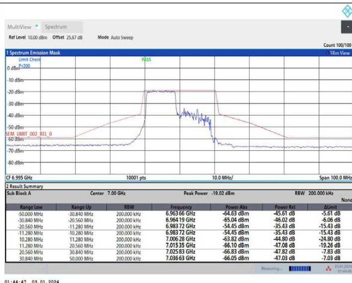
11AX20MIMO_Ant2_6995_26Tone_RU0
