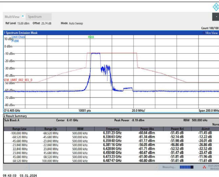
11AX40MIMO Ant1 6405 242Tone RU61
