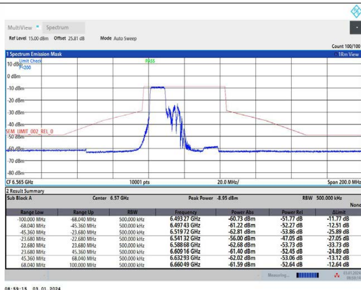
11AX40MIMO Ant1 6565 242Tone RU61
