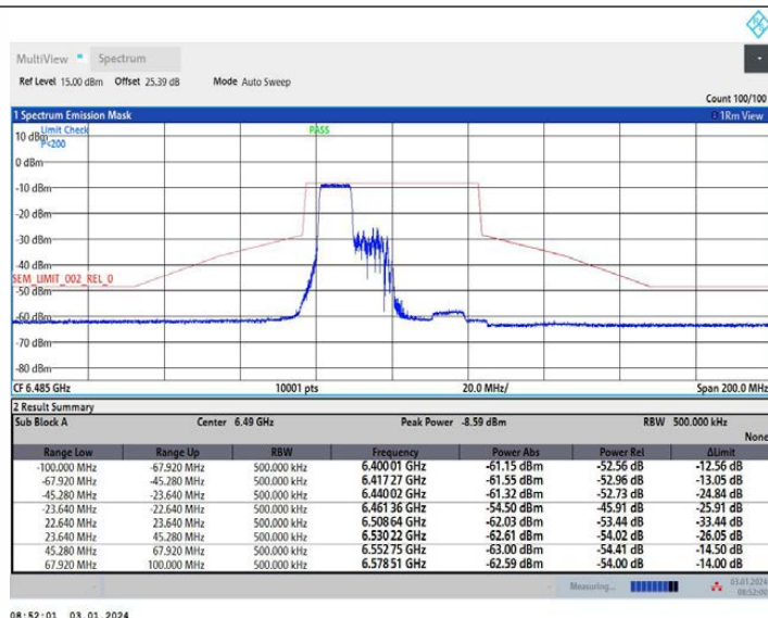
11AX40MIMO Ant1 6485 242Tone RU61
