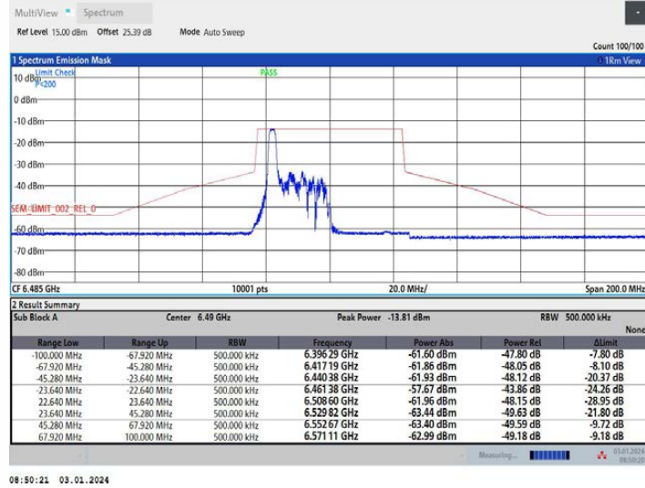
11AX40MIMO Ant1 6485 52Tone RU37
