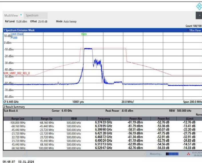
11AX40MIMO Ant2 6445 242Tone RU61
