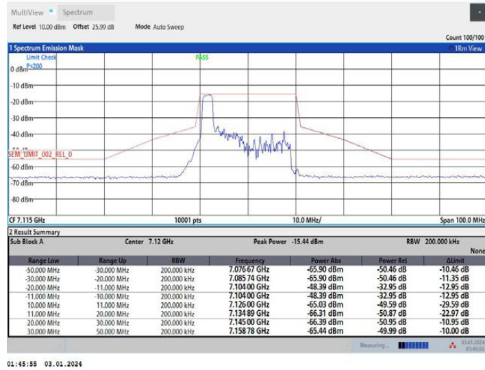
11AX20MIMO_Ant1_7115_52Tone_RU37
