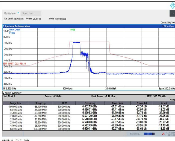
11AX40MIMO Ant1 6525 242Tone RU61
