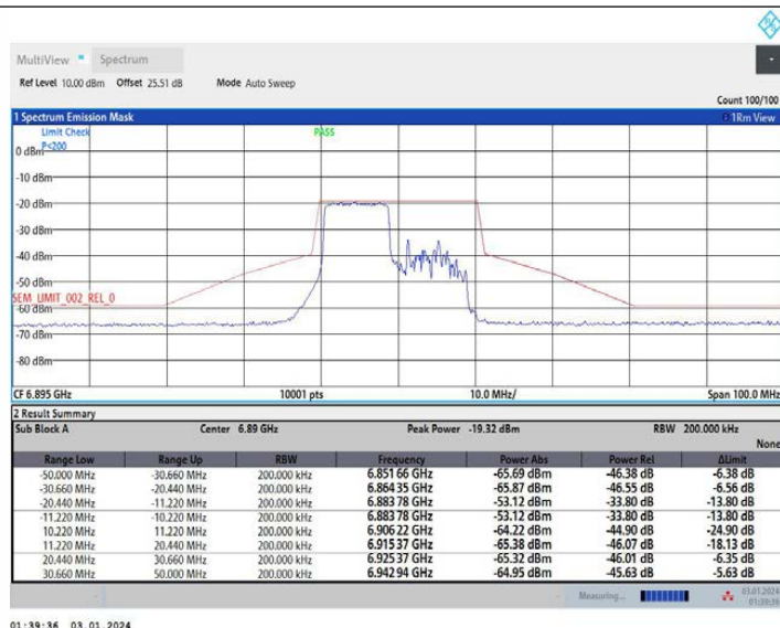
11AX20MIMO_Ant2_6895_26Tone_RU0
