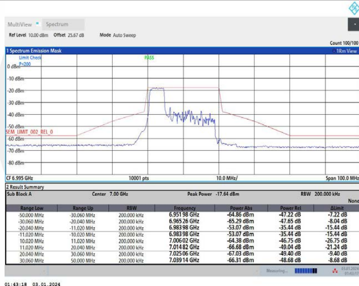
11AX20MIMO_Ant1_6995_106Tone_RU53
