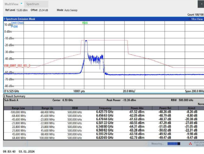
11AX40MIMO Ant1 6525 52Tone RU37
