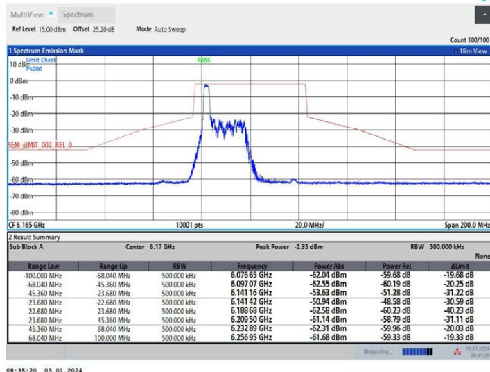
11AX40MIMO Ant1 6165 52Tone RU37
