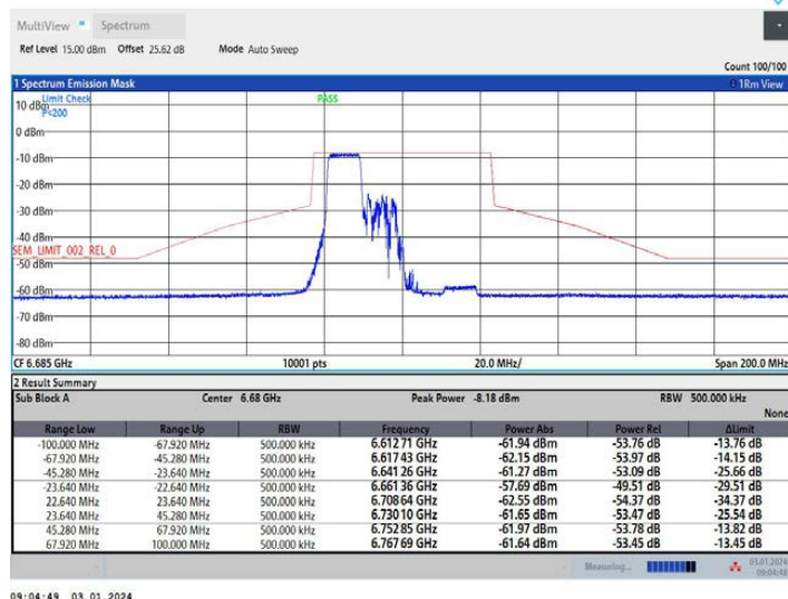
11AX40MIMO Ant2 6685 242Tone RU61
