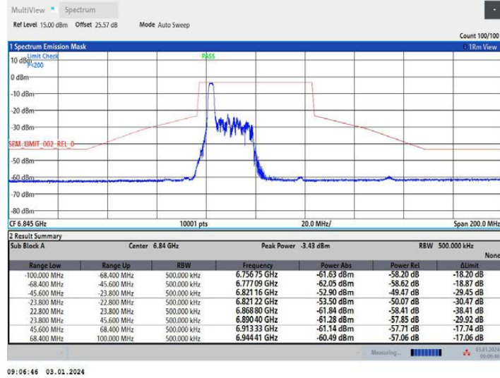
11AX40MIMO Ant1 6845 52Tone RU37
