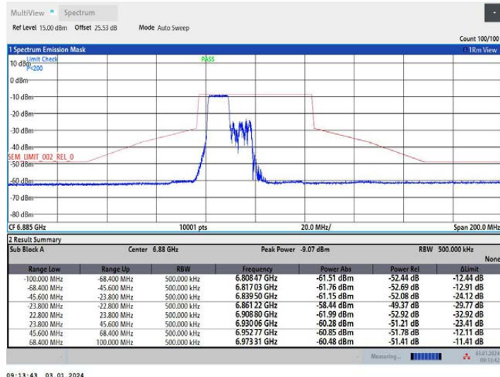
11AX40MIMO Ant1 6885 242Tone RU61
