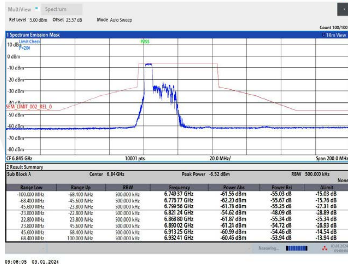
11AX40MIMO Ant1 6845 106Tone RU53
