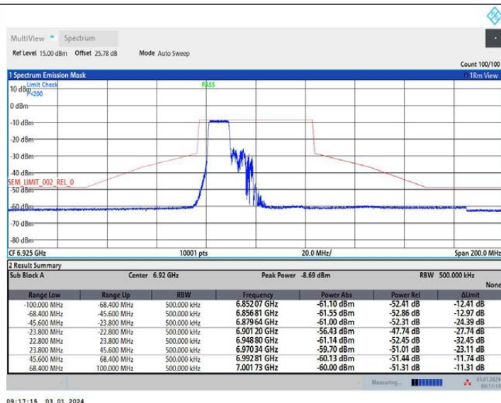
11AX40MIMO Ant1 6925 242Tone RU61
