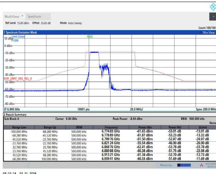
11AX40MIMO Ant2 6845 242Tone RU1
