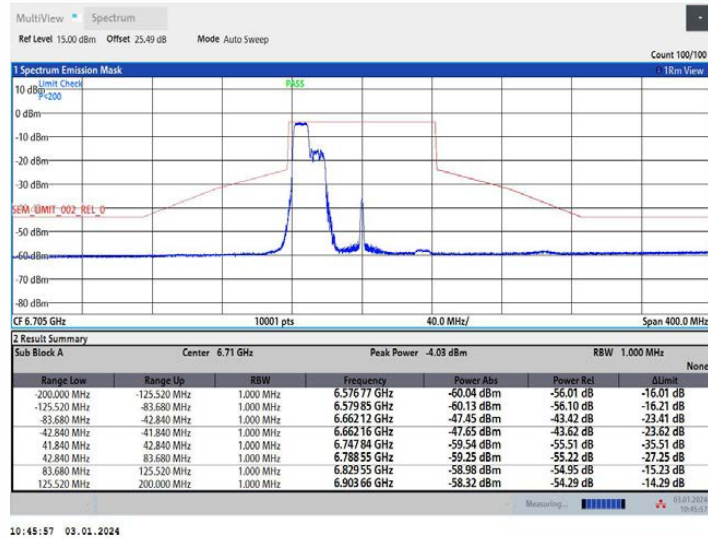
11AX80MIMO Ant1 6705 242Tone RU61
