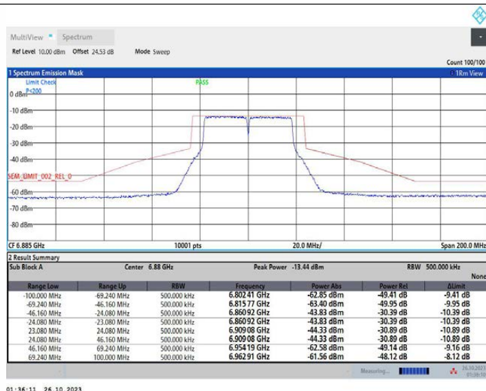
11N40MIMO_Ant2_6885
