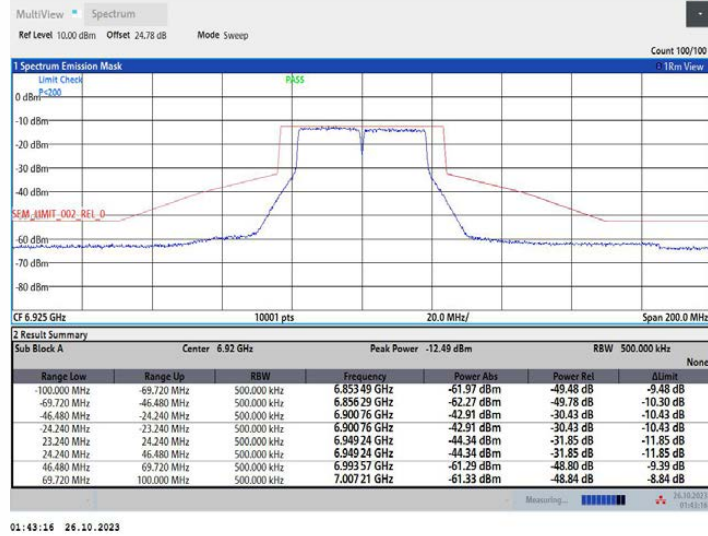
11N40MIMO_Ant2_6925
