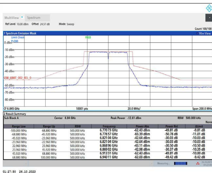
11N40MIMO_Ant2_6845
