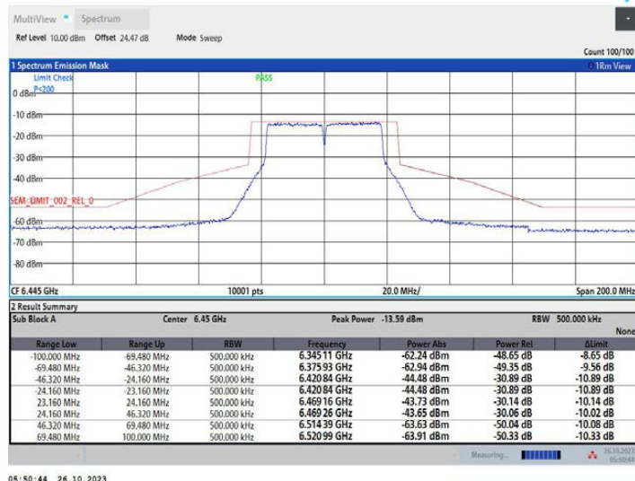
11AC40MIMO_Ant2_6445
