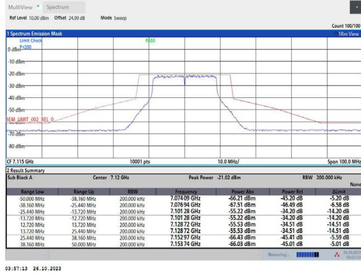
11AC20MIMO_Ant2_7115
