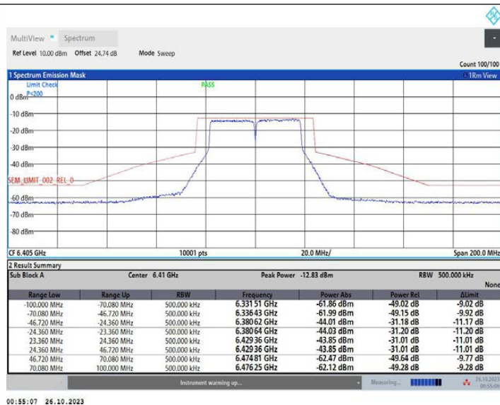
11N40MIMO_Ant2_6405
