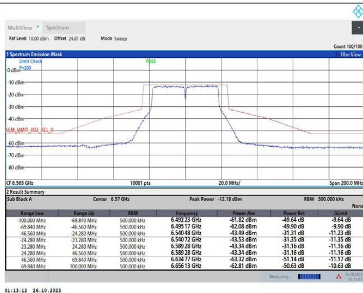
11N40MIMO_Ant2_6565
