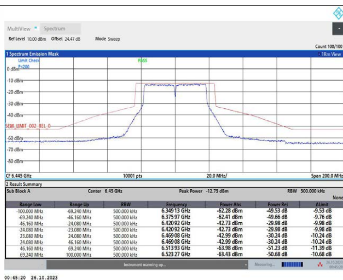
11N40MIMO_Ant2_6445
