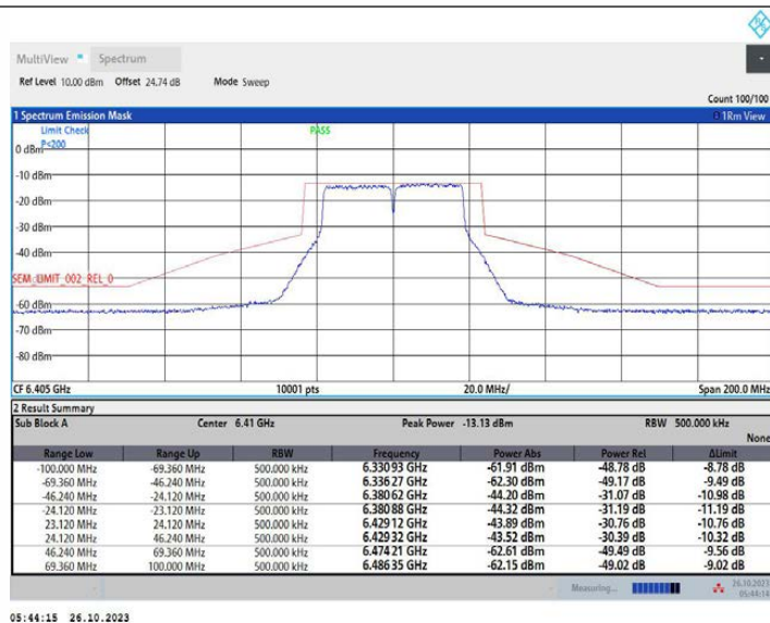
11AC40MIMO_Ant2_6405
