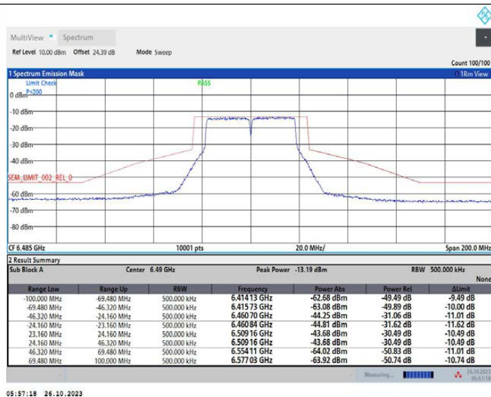
11AC40MIMO_Ant2_6485
