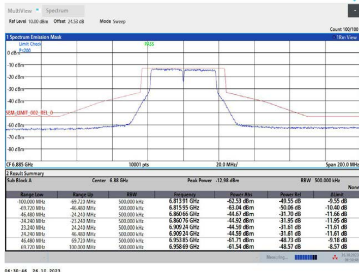
11AC40MIMO_Ant2_6885
