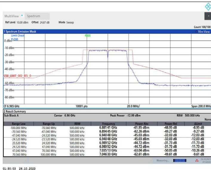
11N40MIMO_Ant2_6965
