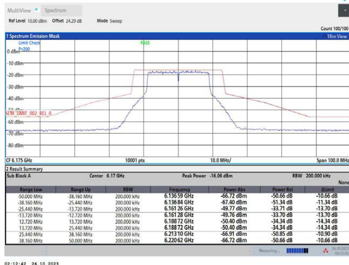
11AC20MIMO_Ant2_6175
