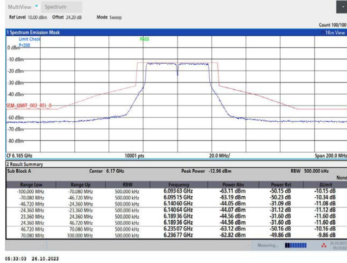
11AC40MIMO_Ant2_6165
