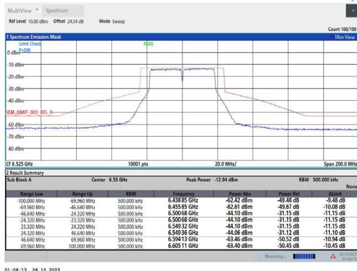
11N40MIMO_Ant2_6525
