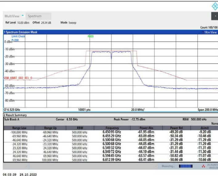
11AC40MIMO_Ant2_6525
