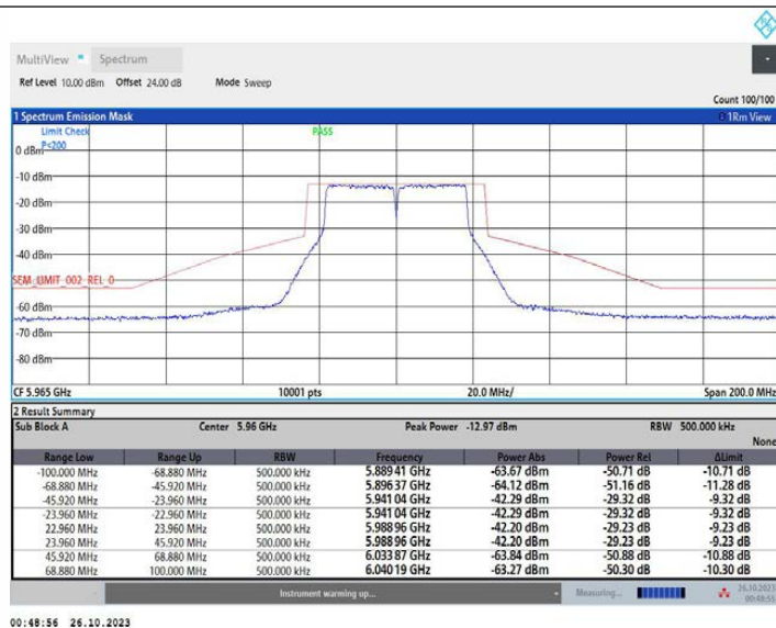
11N40MIMO_Ant2_5965
