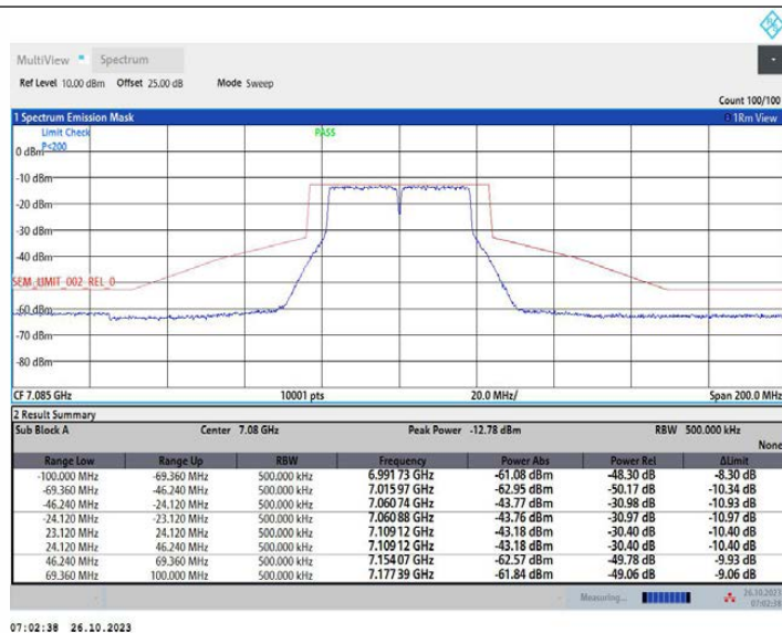
11AC40MIMO_Ant2_7085
