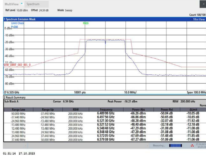
11AX20MIMO_Ant2_6535
