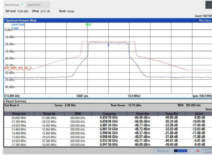
11AX20MIMO_Ant2_6895
