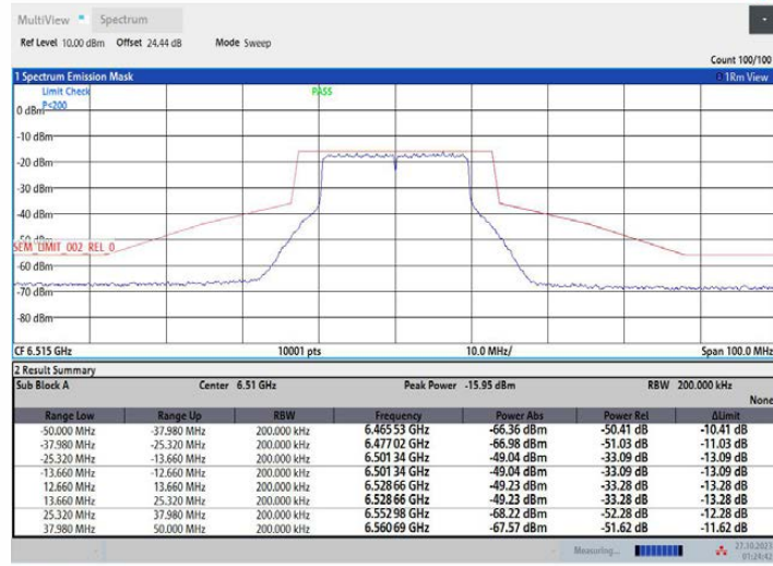
11AX20MIMO_Ant2_6515
