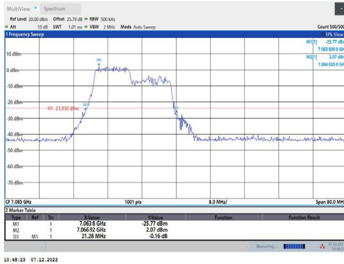
11AX40MIMO_Ant2_7085_242Tone_RU61
