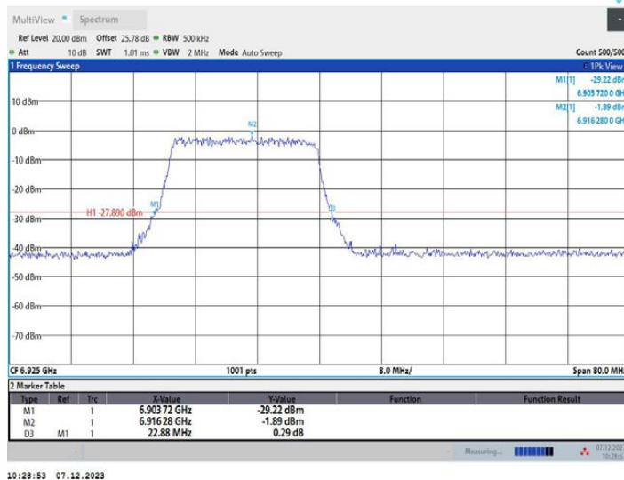
11AX40MIMO_Ant2_6925_26Tone_RU0
