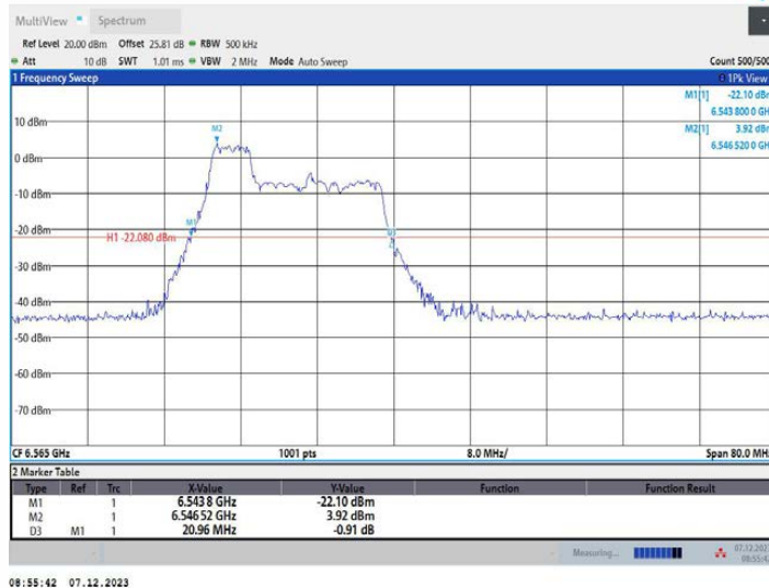
11AX40MIMO_Ant1_6565_106Tone_RU53
