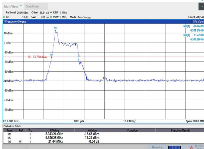
11AX80MIMO_Ant2_6385_52Tone_RU37
