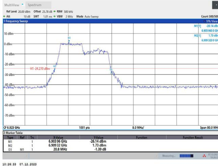
11AX40MIMO_Ant1_6925_242Tone_RU61
