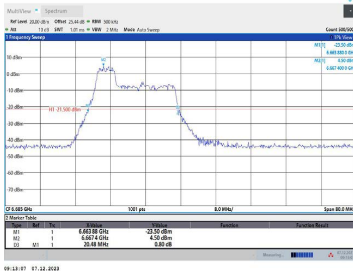
11AX40MIMO_Ant1_6685_106Tone_RU53
