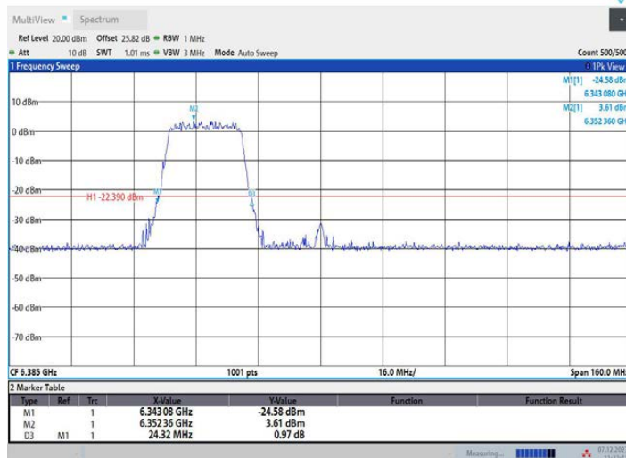
11AX80MIMO_Ant1_6385_484Tone_RU65
