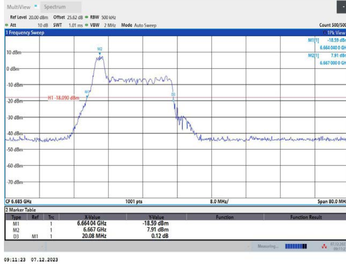
11AX40MIMO_Ant2_6685_52Tone_RU37
