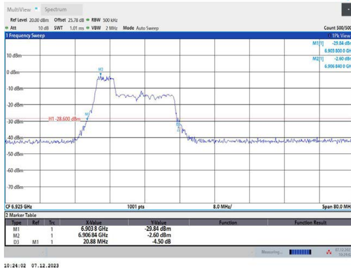
11AX40MIMO_Ant1_6925_106Tone_RU53
