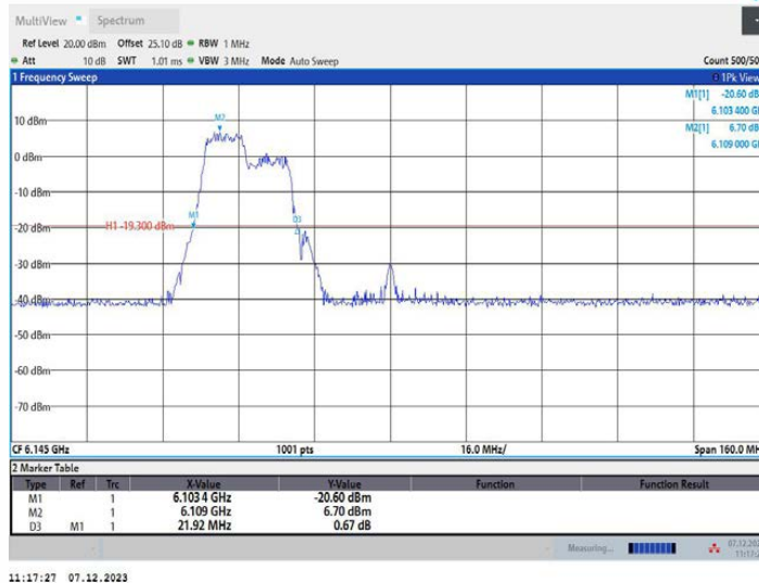
11AX80MIMO_Ant2_6145_242Tone_RU61
