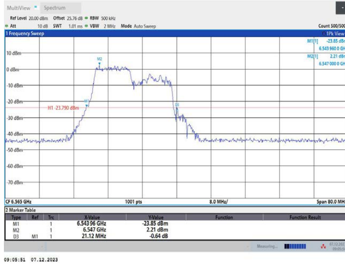
11AX40MIMO_Ant2_6565_242Tone_RU61
