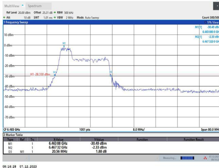
11AX40MIMO_Ant2_6485_106Tone_RU53
