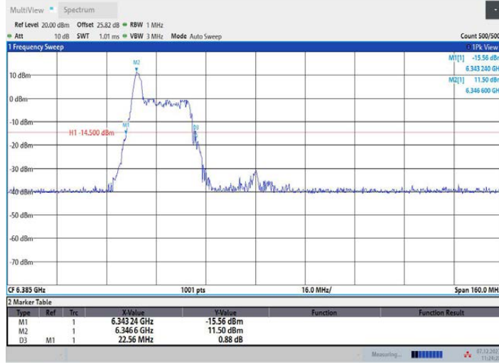
11AX80MIMO_Ant1_6385_52Tone_RU37
