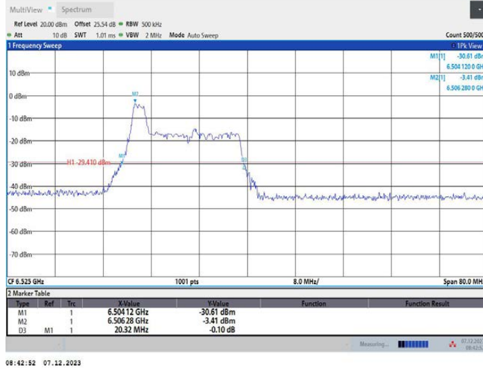
11AX40MIMO_Ant1_6525_52Tone_RU37
