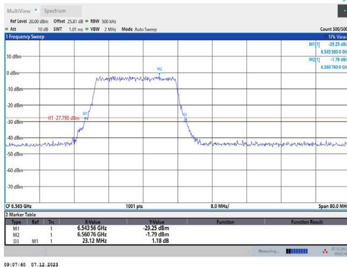
11AX40MIMO_Ant2_6565_26Tone_RU0
