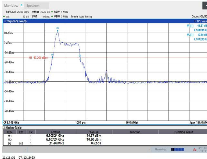
11AX80MIMO_Ant2_6145_52Tone_RU37
