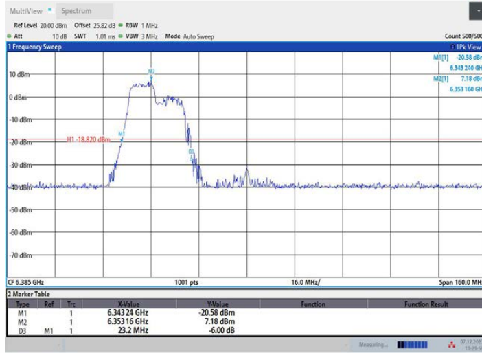
11AX80MIMO_Ant1_6385_242Tone_RU61
