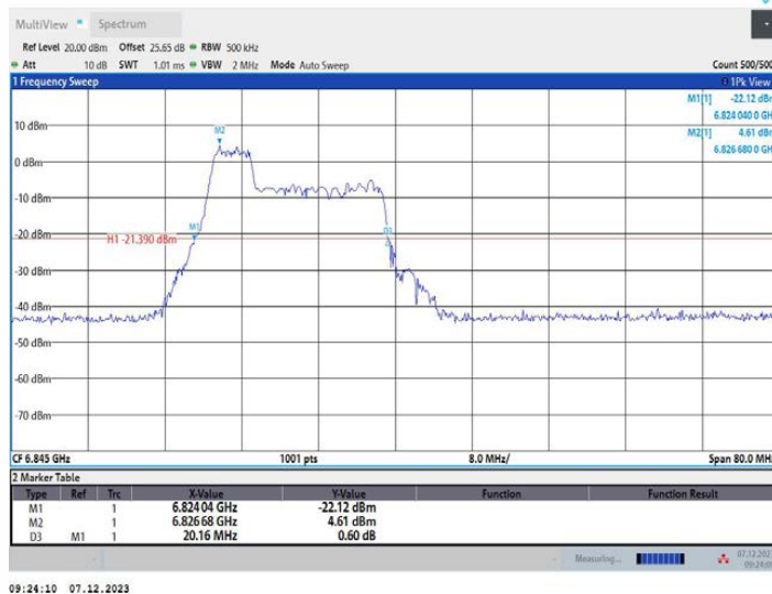
11AX40MIMO_Ant2_6845_106Tone_RU53
