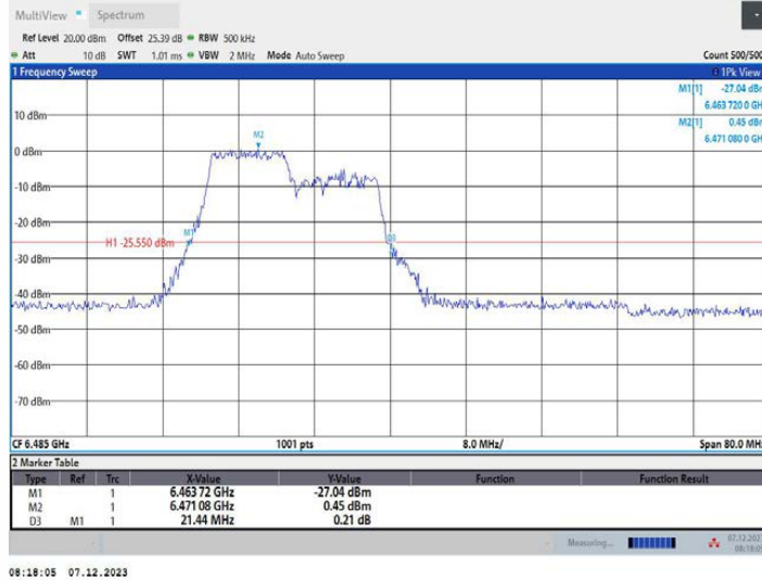
11AX40MIMO_Ant1_6485_242Tone_RU61
