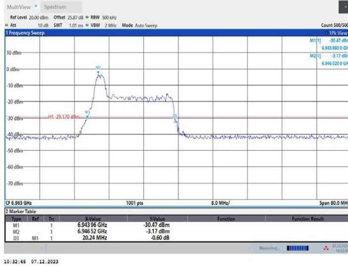
11AX40MIMO_Ant2_6965_52Tone_RU37
