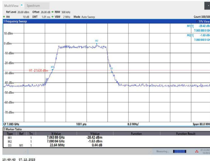
11AX40MIMO_Ant2_7085_26Tone_RU0
