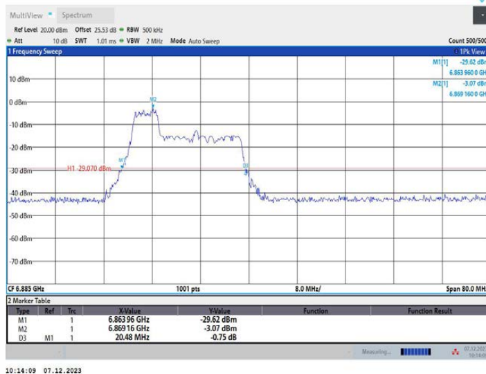
11AX40MIMO_Ant1_6885_106Tone_RU53
