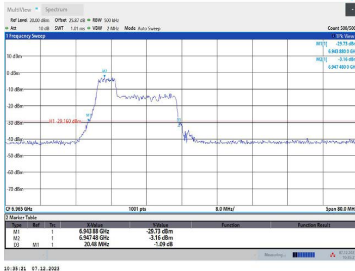
11AX40MIMO_Ant2_6965_106Tone_RU53
