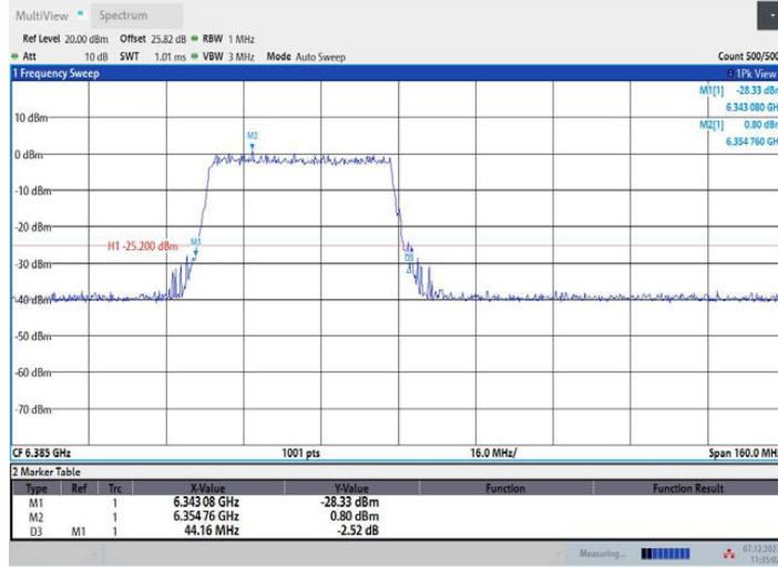
11AX80MIMO_Ant2_6385_26Tone_RU0
