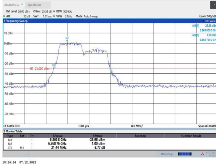
11AX40MIMO_Ant1_6885_242Tone_RU61
