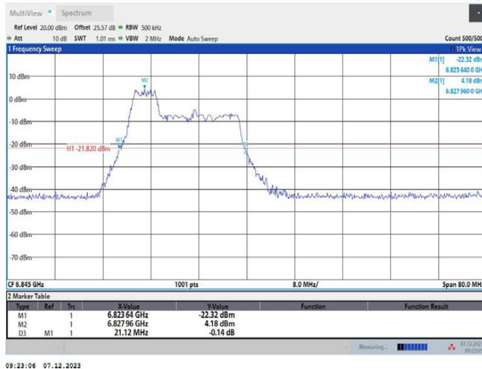
11AX40MIMO_Ant1_6845_106Tone_RU53
