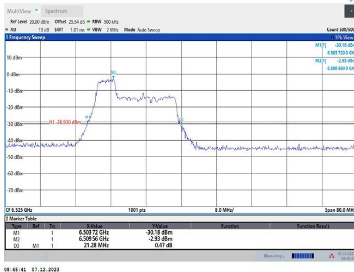
11AX40MIMO_Ant1_6525_106Tone_RU53
