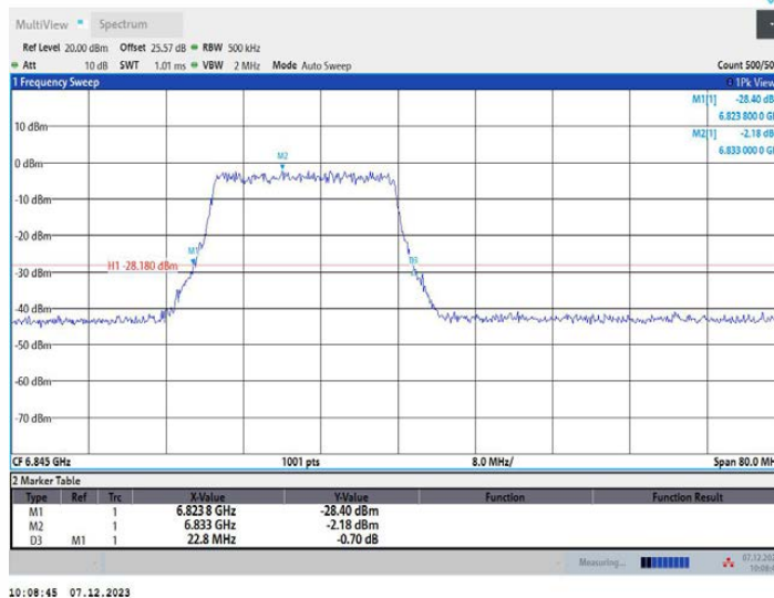
11AX40MIMO_Ant2_6845_26Tone_RU0
