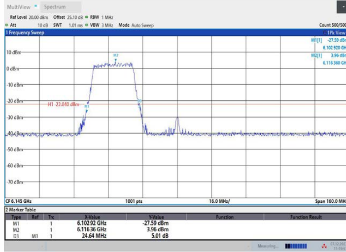
11AX80MIMO_Ant2_6145_484Tone_RU65
