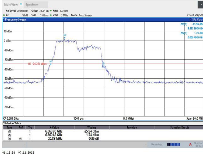
11AX40MIMO_Ant1_6685_242Tone_RU61
