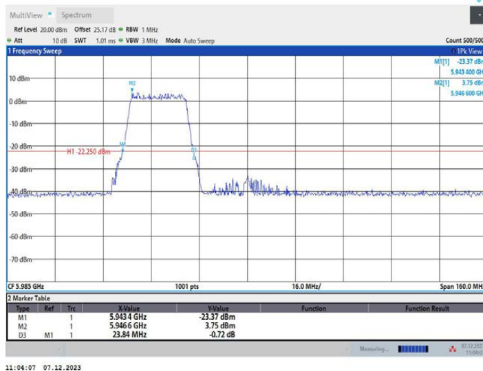
11AX80MIMO_Ant1_5985_484Tone_RU65
