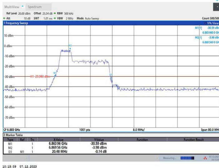
11AX40MIMO_Ant2_6885_106Tone_RU53
