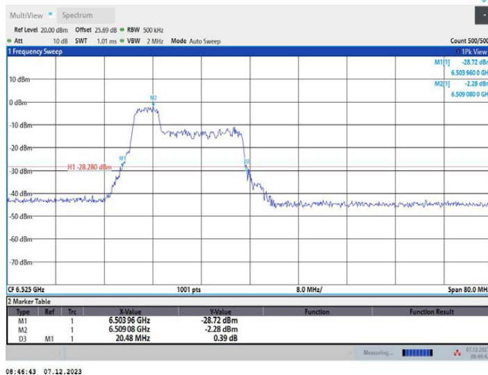
11AX40MIMO_Ant2_6525_106Tone_RU53
