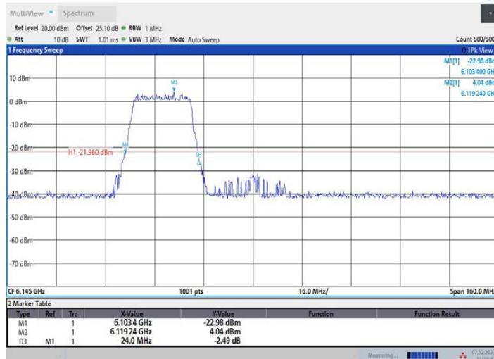
11AX80MIMO_Ant1_6145_484Tone_RU65
