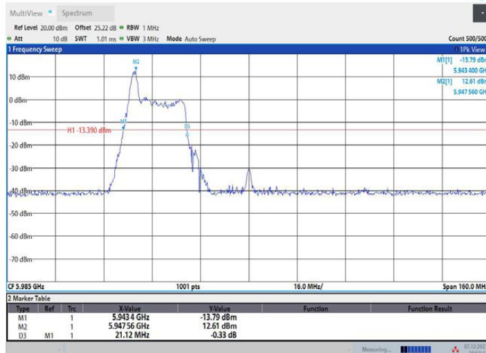
11AX80MIMO_Ant2_5985_52Tone_RU37
