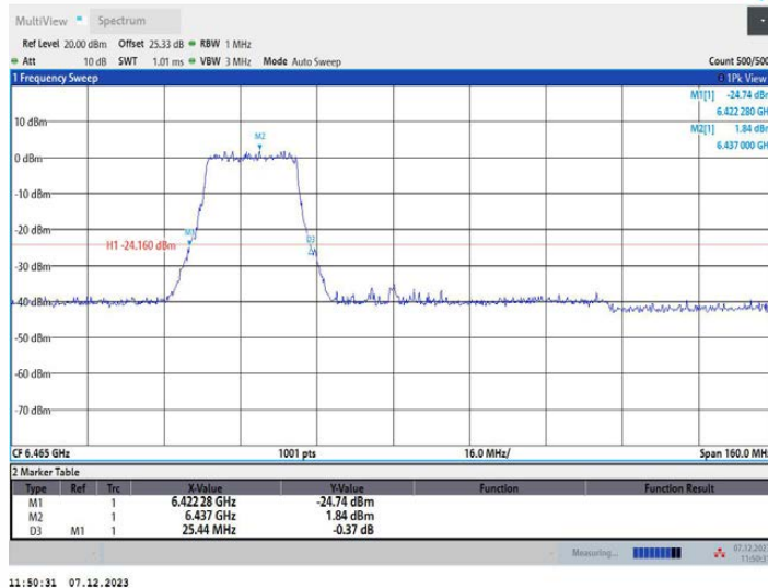
11AX80MIMO_Ant1_6465_484Tone_RU65
