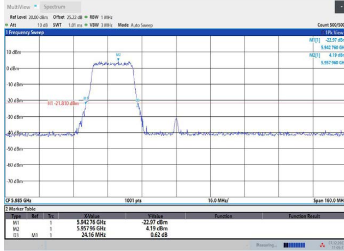
11AX80MIMO_Ant2_5985_484Tone_RU65
