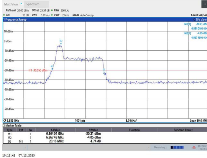
11AX40MIMO_Ant2_6885_52Tone_RU37
