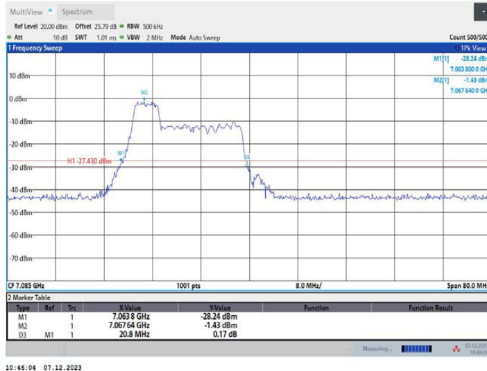
11AX40MIMO_Ant2_7085_106Tone_RU53
