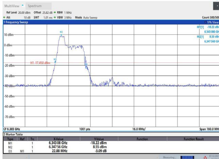
11AX80MIMO_Ant1_6385_106Tone_RU53
