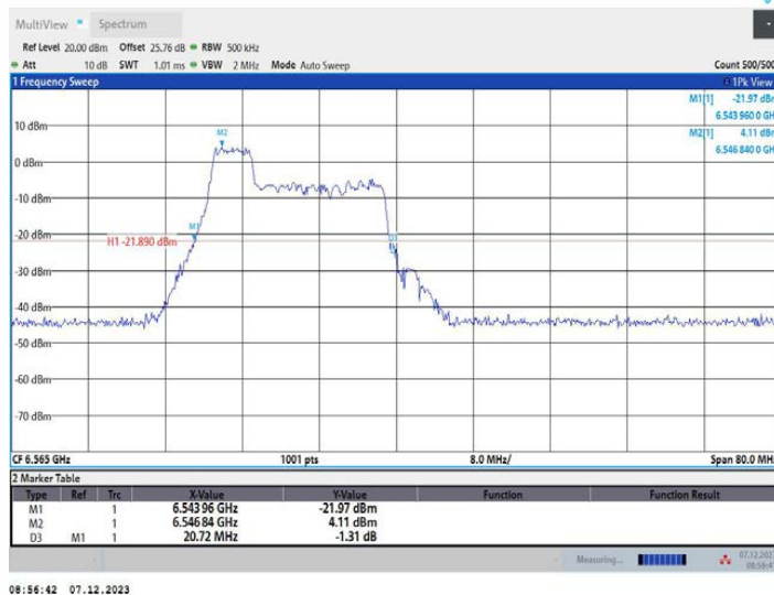
11AX40MIMO_Ant2_6565_106Tone_RU53
