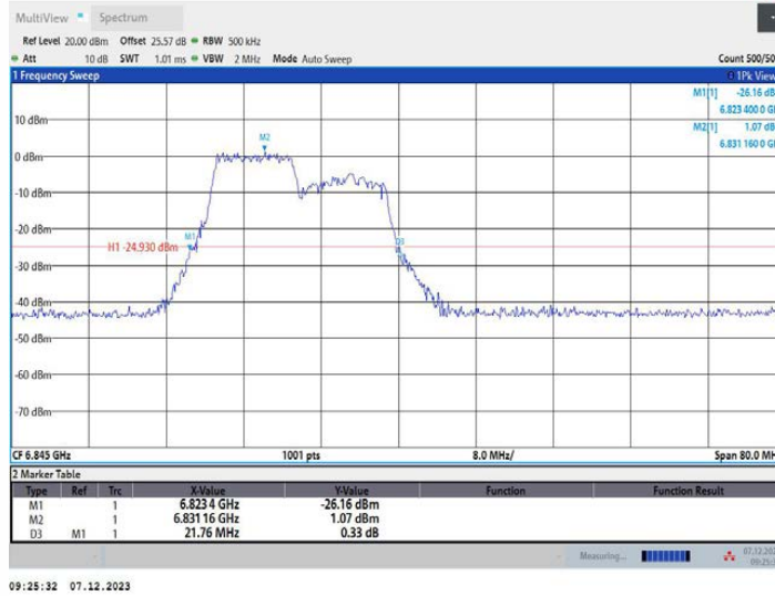
11AX40MIMO_Ant1_6845_242Tone_RU61
