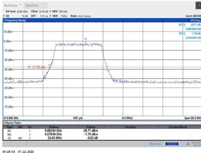
11AX40MIMO_Ant2_6685_26Tone_RU0
