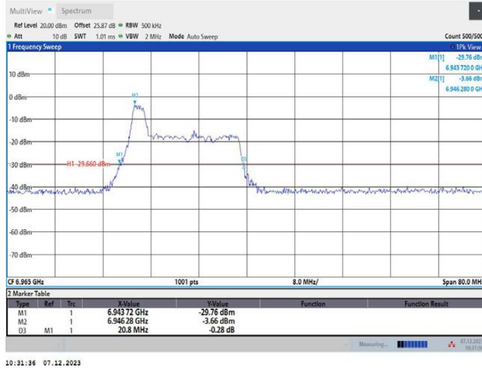
11AX40MIMO_Ant1_6965_52Tone_RU37
