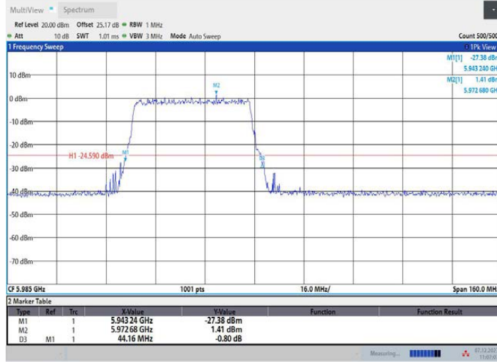
11AX80MIMO_Ant2_5985_26Tone_RU0
