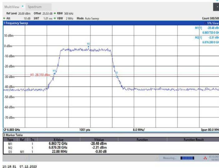
11AX40MIMO_Ant2_6885_26Tone_RU0
