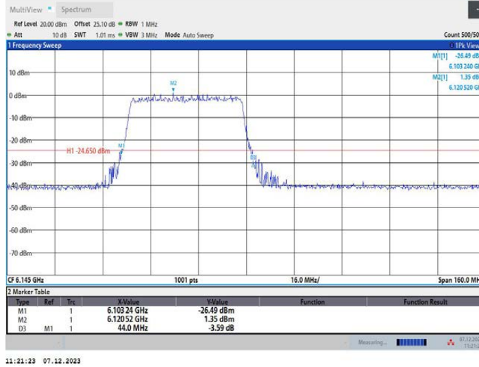
11AX80MIMO_Ant2_6145_26Tone_RU0
