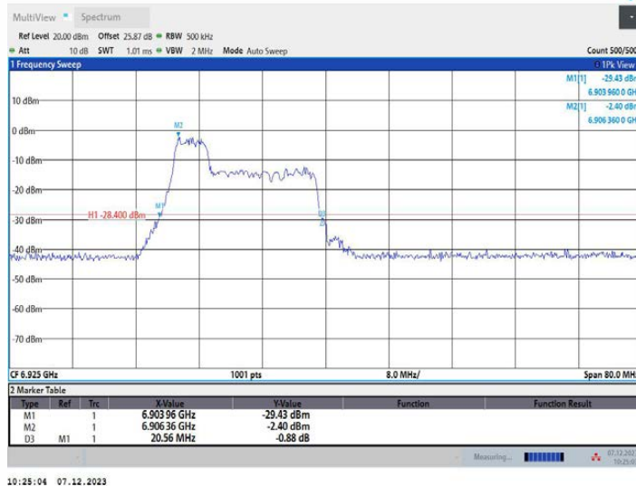
11AX40MIMO_Ant2_6925_106Tone_RU53
