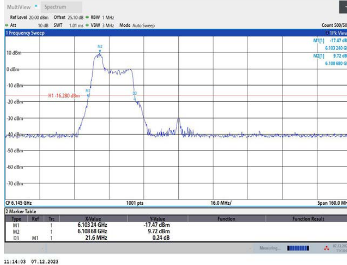
11AX80MIMO_Ant2_6145_106Tone_RU53
