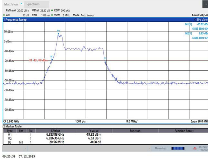
11AX40MIMO_Ant1_6845_52Tone_RU37
