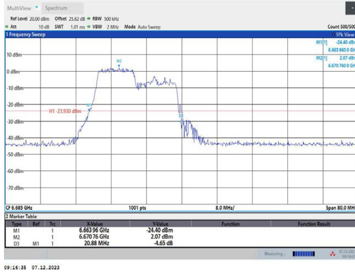
11AX40MIMO_Ant2_6685_242Tone_RU61
