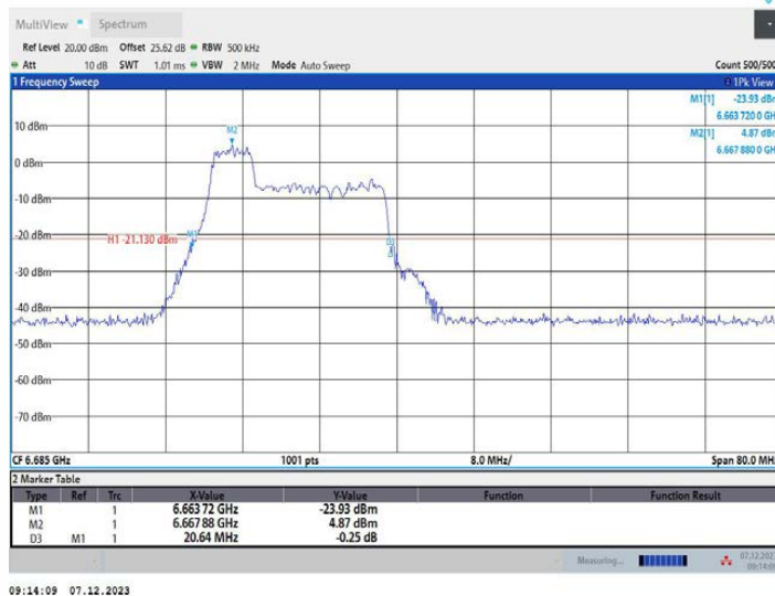
11AX40MIMO_Ant2_6685_106Tone_RU53
