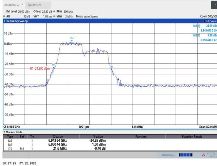
11AX40MIMO_Ant1_6965_242Tone_RU61
