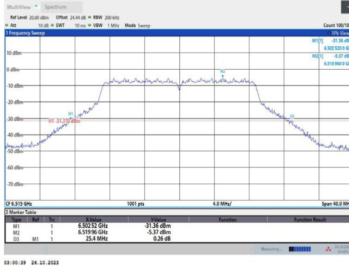
11AC20MIMO_Ant2_6515
