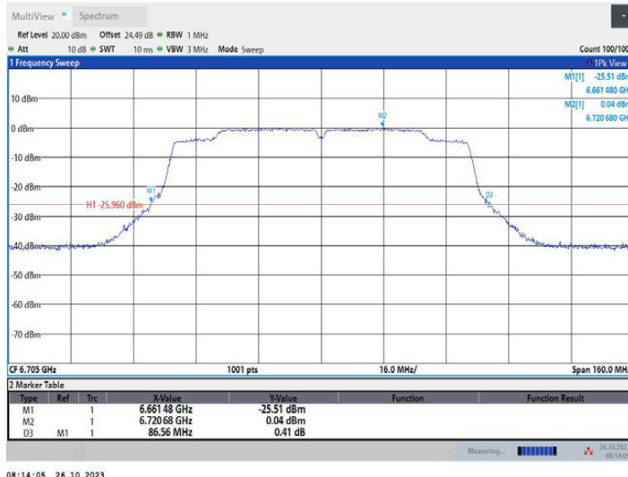
11AC80MIMO_Ant2_6705
