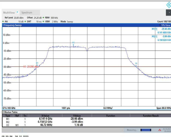
11AC40MIMO_Ant2_6165
