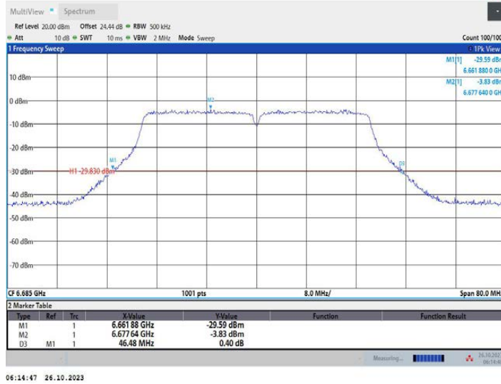
11AC40MIMO_Ant2_6685
