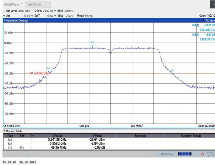
11AC40MIMO_Ant2_5965
