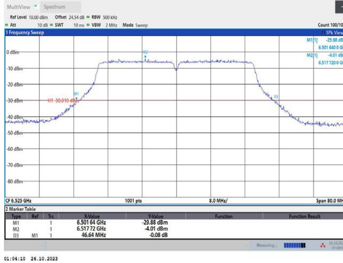
11N40MIMO_Ant2_6525
