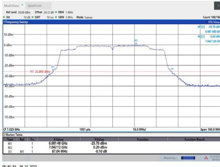
11AC80MIMO_Ant2_7025
