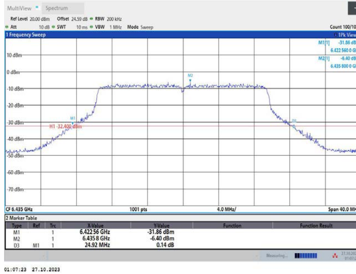
11AX20MIMO_Ant2_6435
