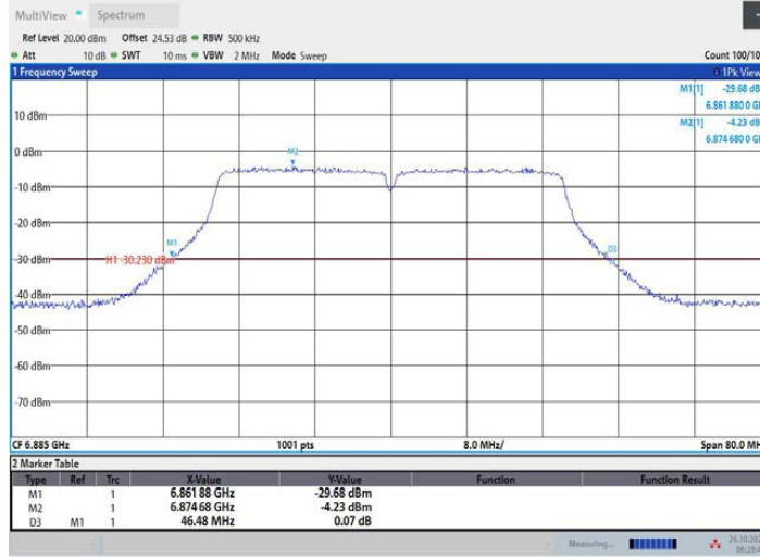
11AC40MIMO_Ant2_6885
