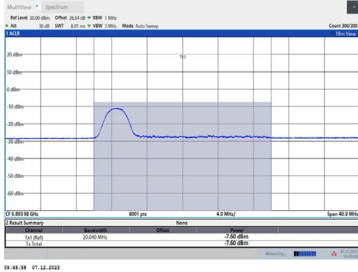
11AX20MIMO_Ant1_6895_52Tone_RU37
