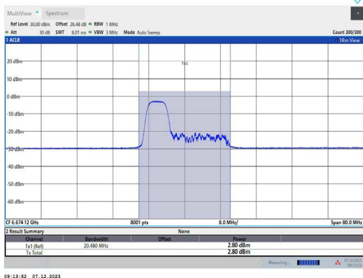
11AX40MIMO_Ant1_6685_106Tone_RU53
