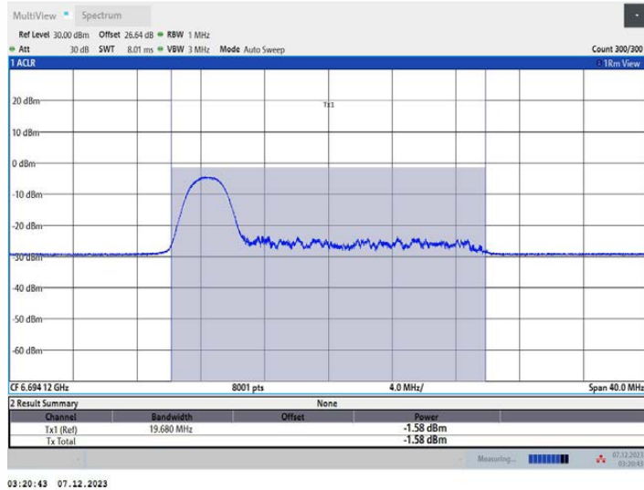
11AX20MIMO_Ant2_6695_52Tone_RU37
