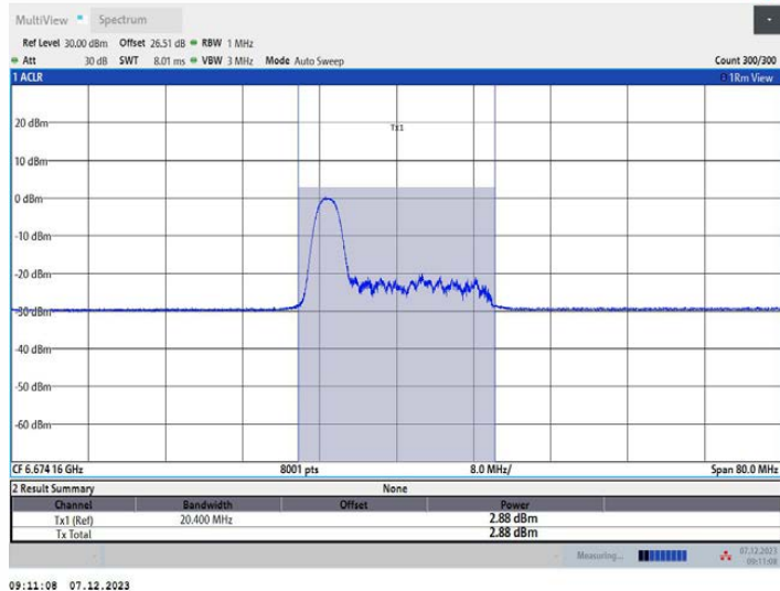
11AX40MIMO_Ant1_6685_52Tone_RU37
