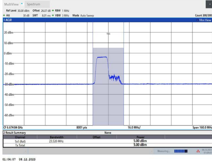
11AX80MIMO_Ant1_6705_242Tone_RU61
