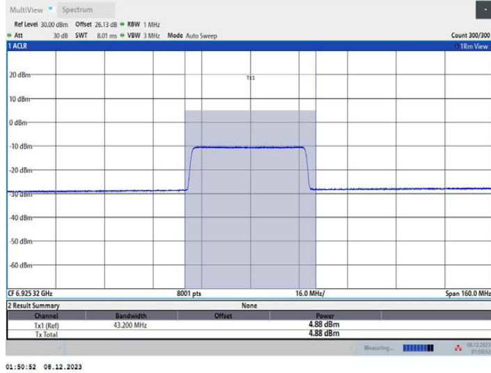
11AX80MIMO_Ant2_6945_26Tone_RU0
