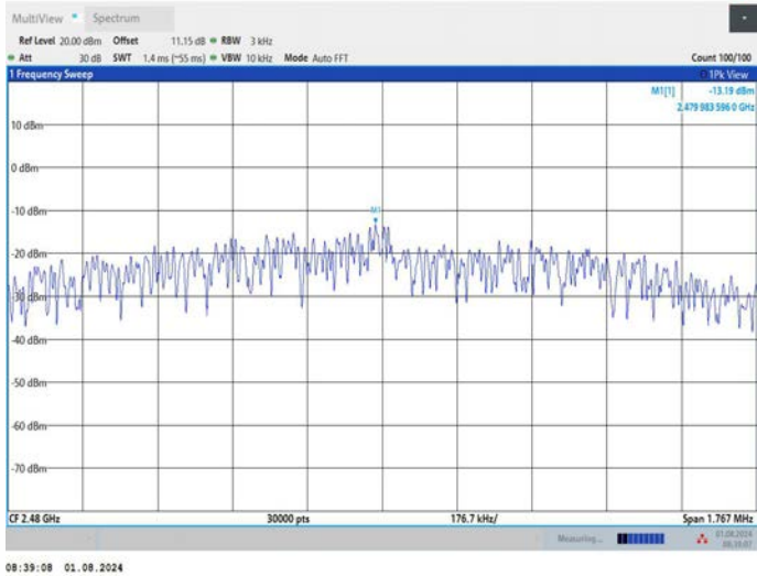
BLE_2M_Ant1_2480
