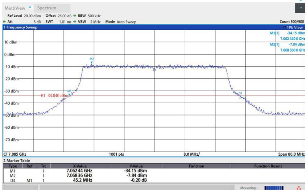
11AX40MIMO-Ant1-7085
