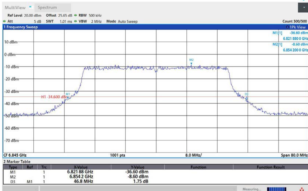
11AX40MIMO-Ant2-6845
