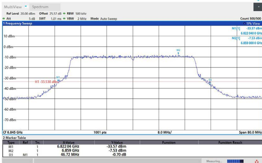
11AX40MIMO-Ant1-6845
