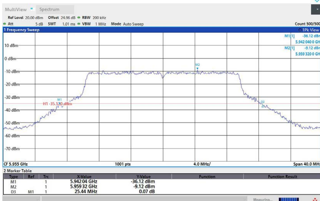
11AX20MIMO-Ant2-5955
