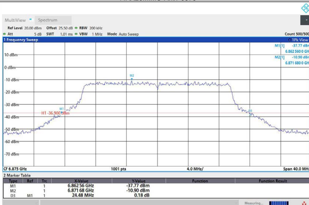
11AX20MIMO-Ant2-6875
