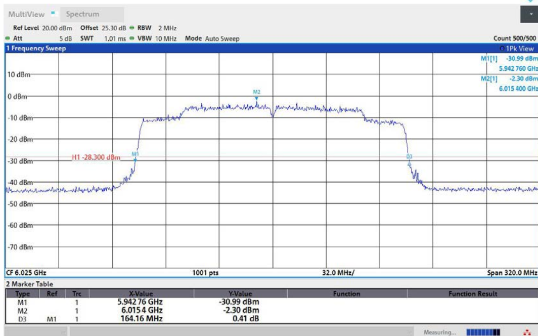
11AX160MIMO-Ant1-6025
