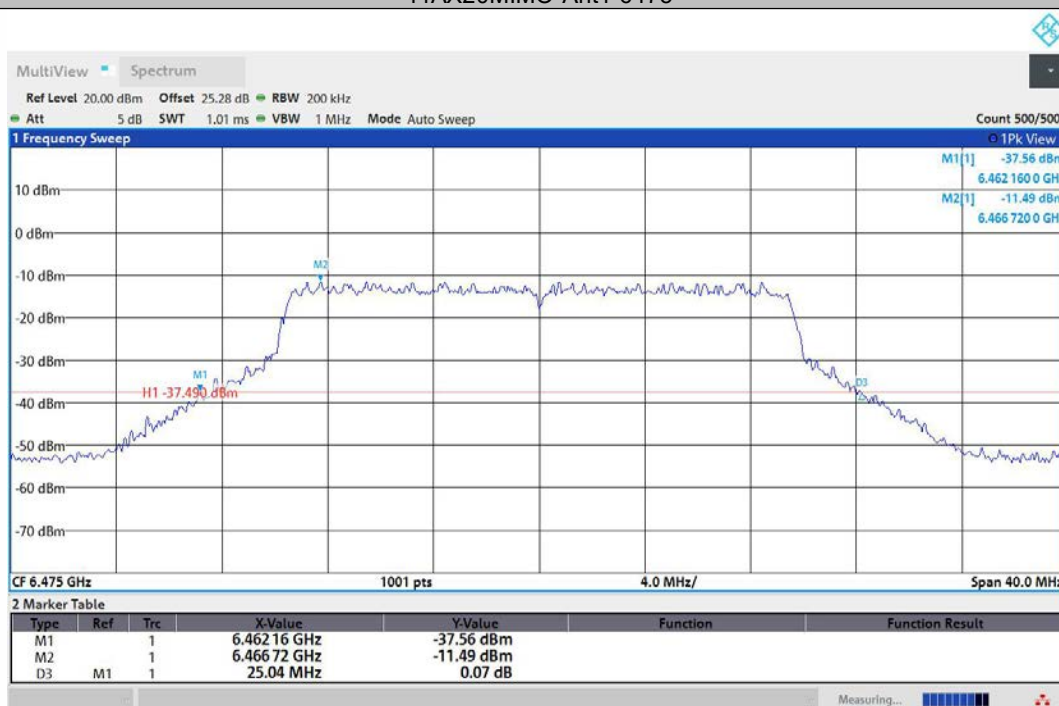
11AX20MIMO-Ant2-6475
