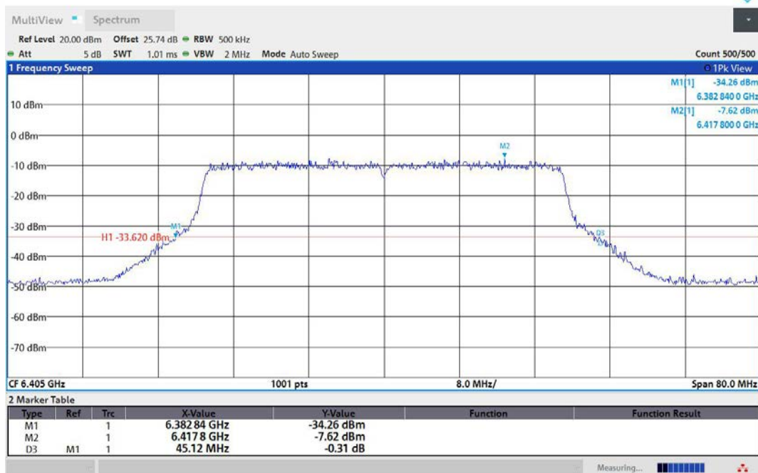
11AX40MIMO-Ant1-6405
