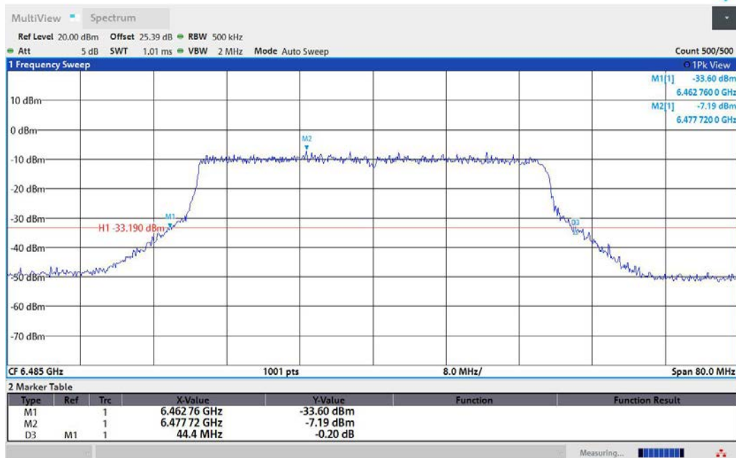
11AX40MIMO-Ant1-6485
