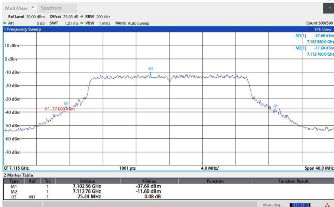
11AX20MIMO-Ant2-7115
