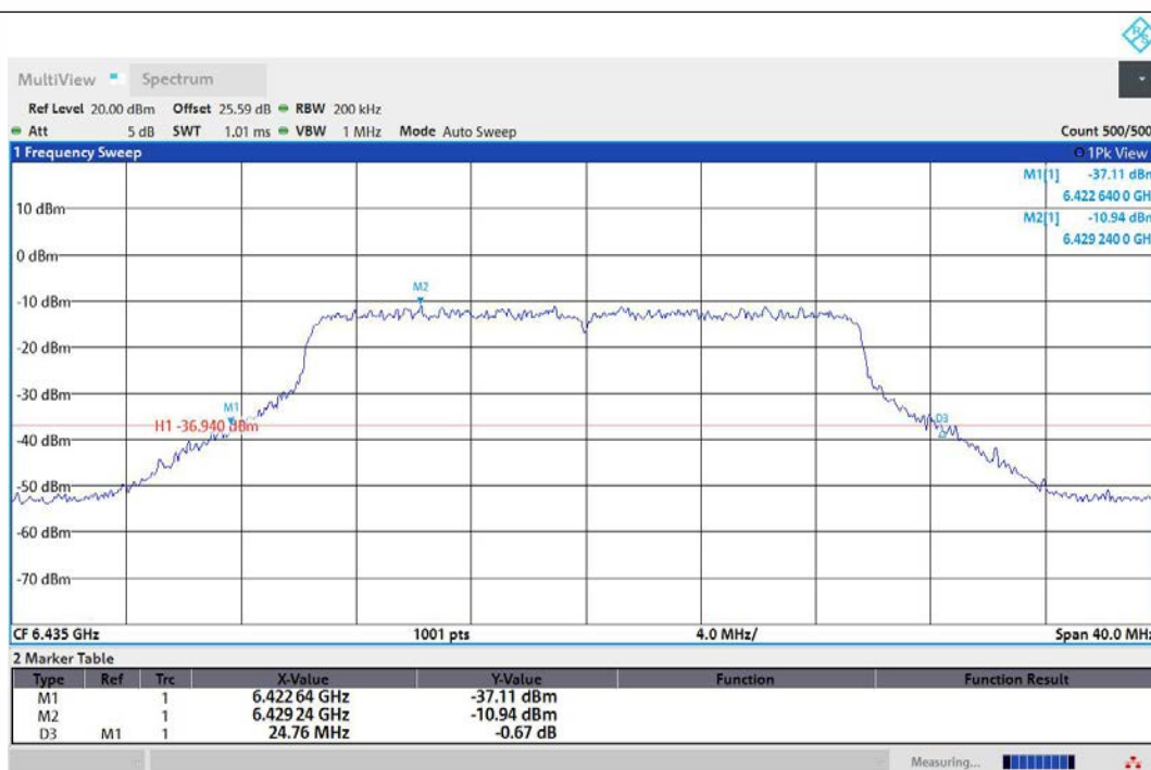
11AX20MIMO-Ant1-6435
