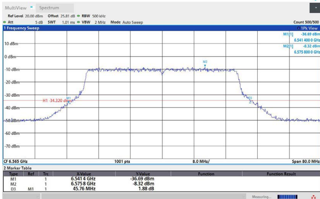
11AX40MIMO-Ant1-6565
