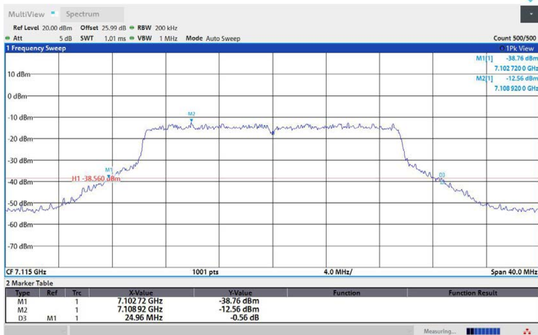
11AX20MIMO-Ant1-7115
