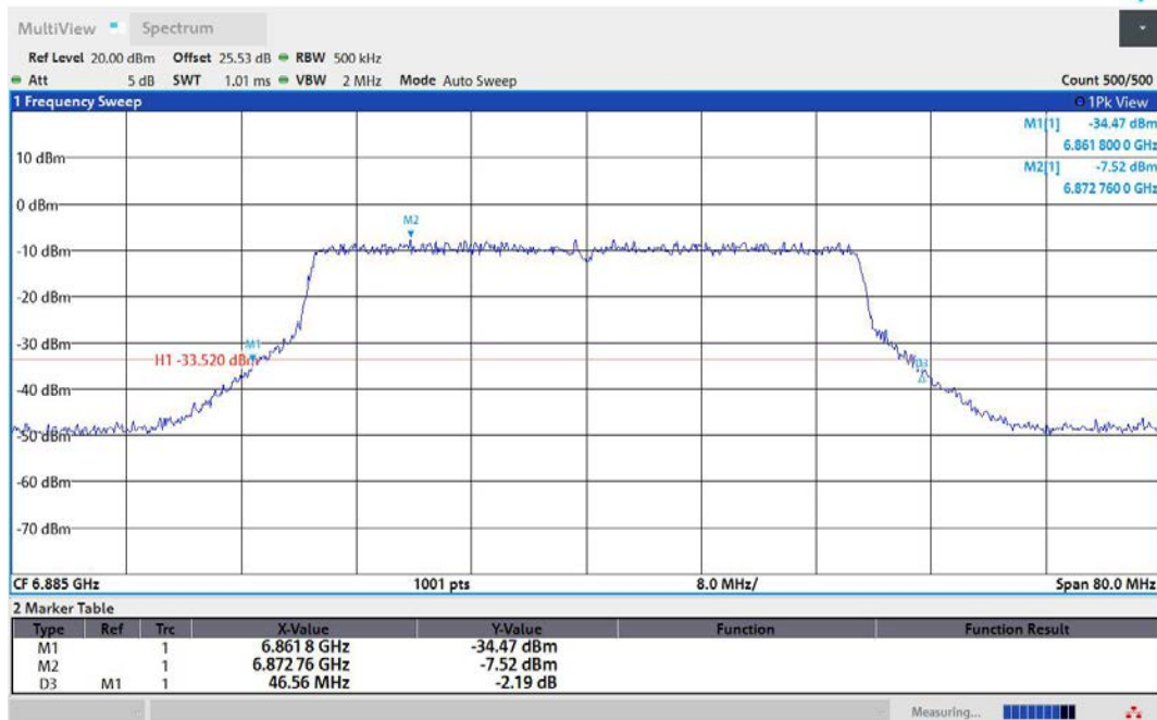
11AX40MIMO-Ant1-6885
