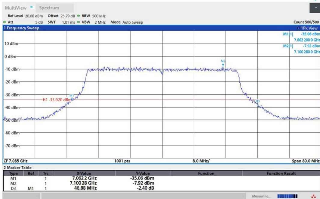
11AX40MIMO-Ant2-7085
