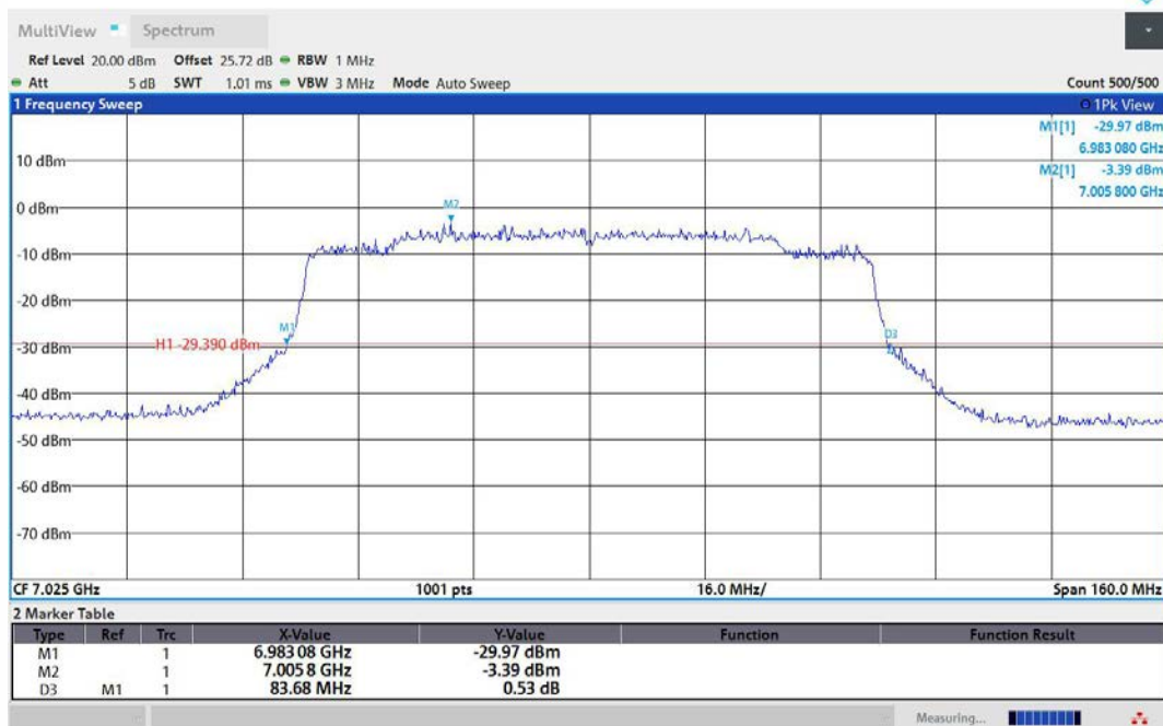
11AX80MIMO-Ant1-7025
