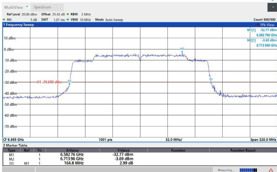
11AX160MIMO-Ant1-6665
