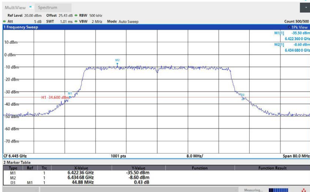
11AX40MIMO-Ant2-6445
