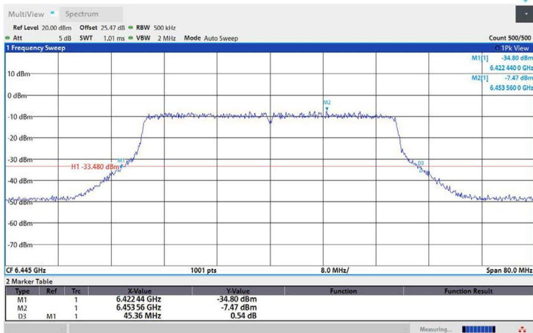
11AX40MIMO-Ant1-6445
