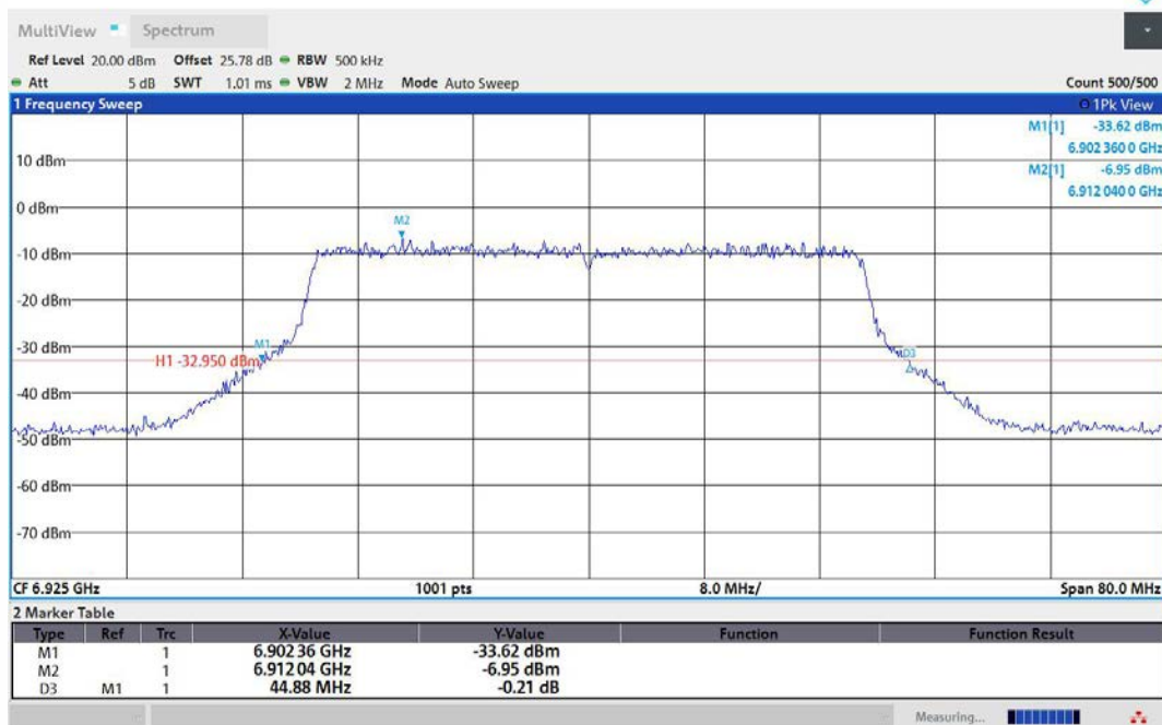
11AX40MIMO-Ant1-6925
