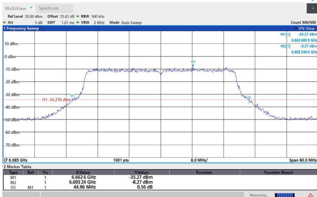
11AX40MIMO-Ant2-6685
