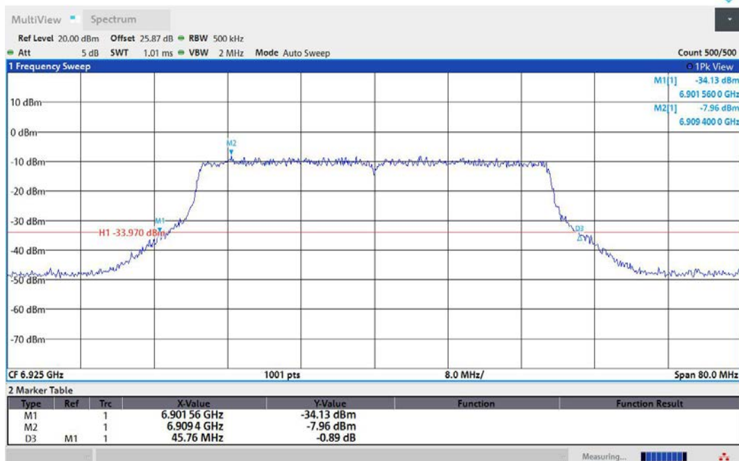
11AX40MIMO-Ant2-6925
