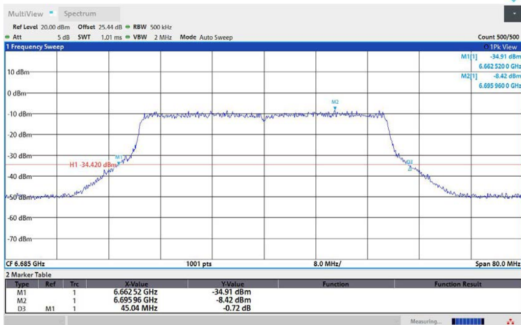
11AX40MIMO-Ant1-6685
