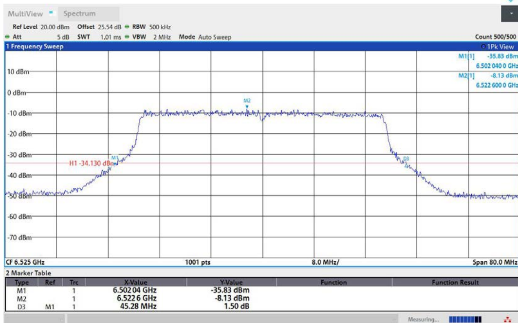
11AX40MIMO-Ant1-6525
