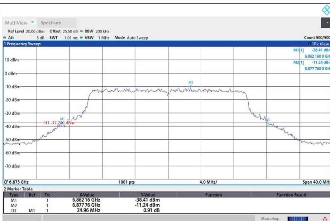
11AX20MIMO-Ant1-6875
