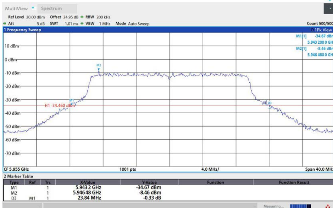
11AX20MIMO-Ant1-5955
