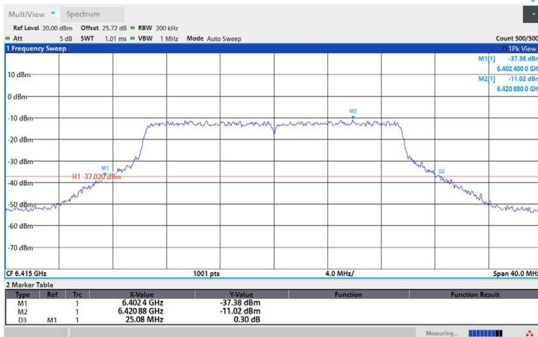
11AX20MIMO-Ant1-6415
