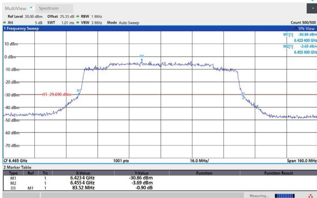
11AX80MIMO-Ant1-6465
