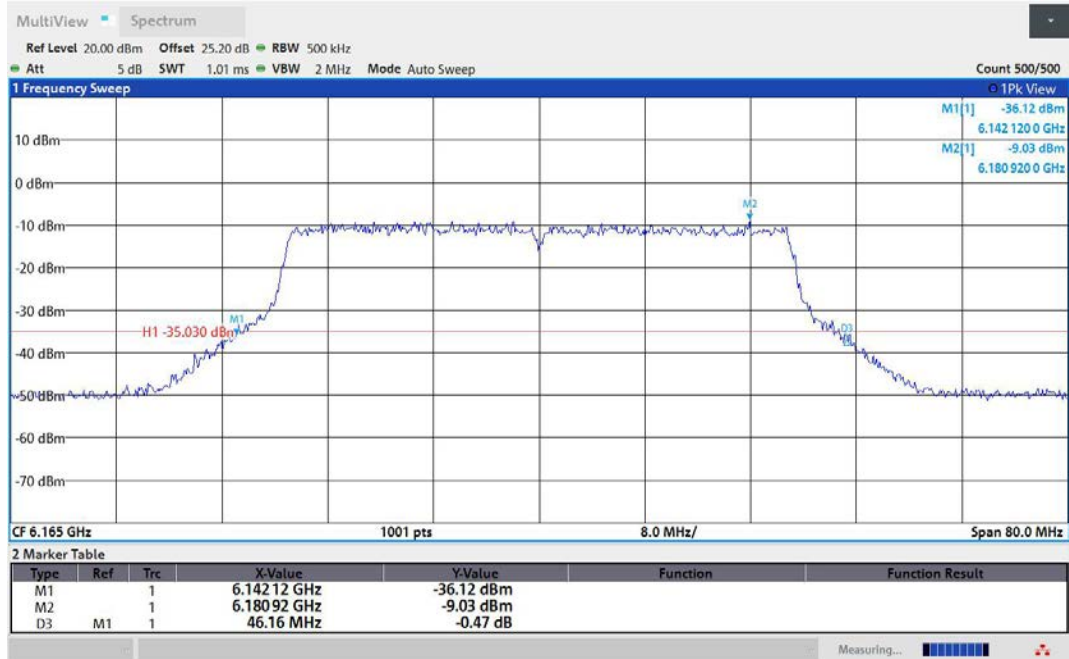
11AX40MIMO-Ant1-6165
