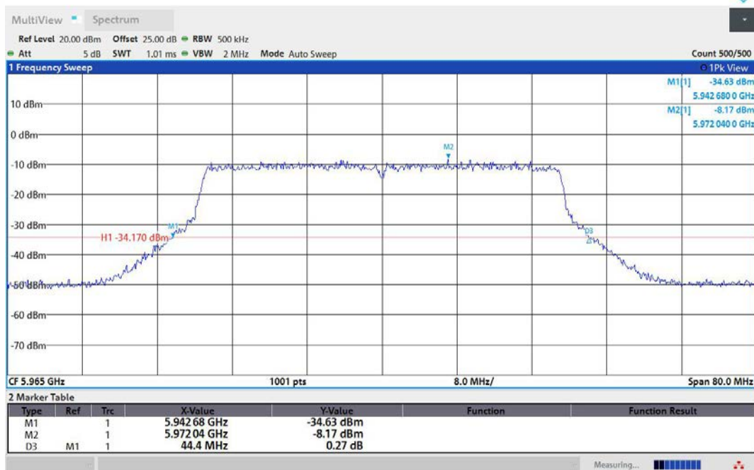
11AX40MIMO-Ant1-5965
