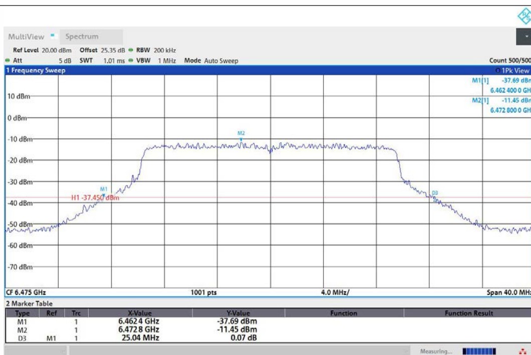
11AX20MIMO-Ant1-6475
