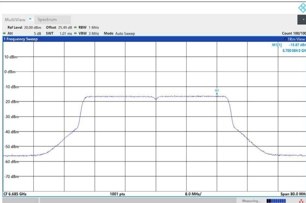
11AX40MIMO-Ant1-6685-PASS
