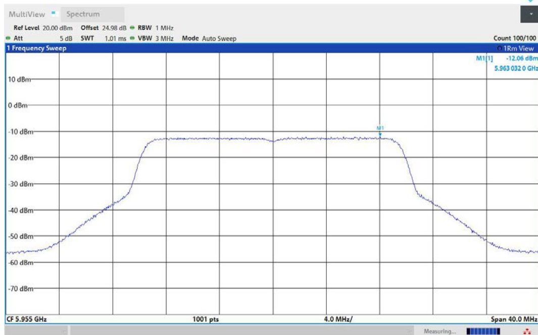
11AX20MIMO-Ant1-5955-PASS
