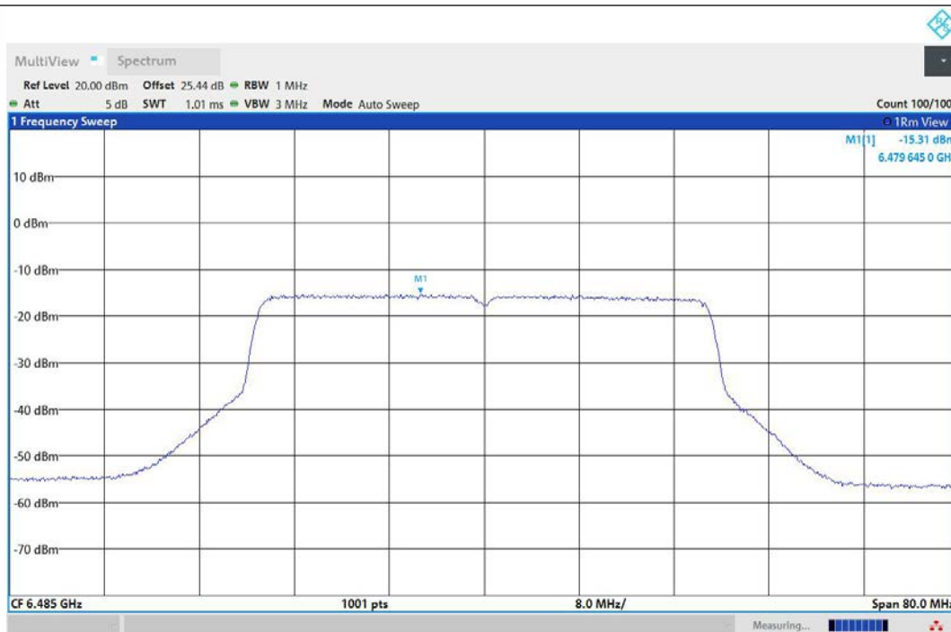
11AX40MIMO-Ant1-6485-PASS
