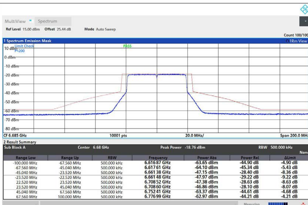
NTNV-11AX40MIMO-Ant1-6685-PASS
