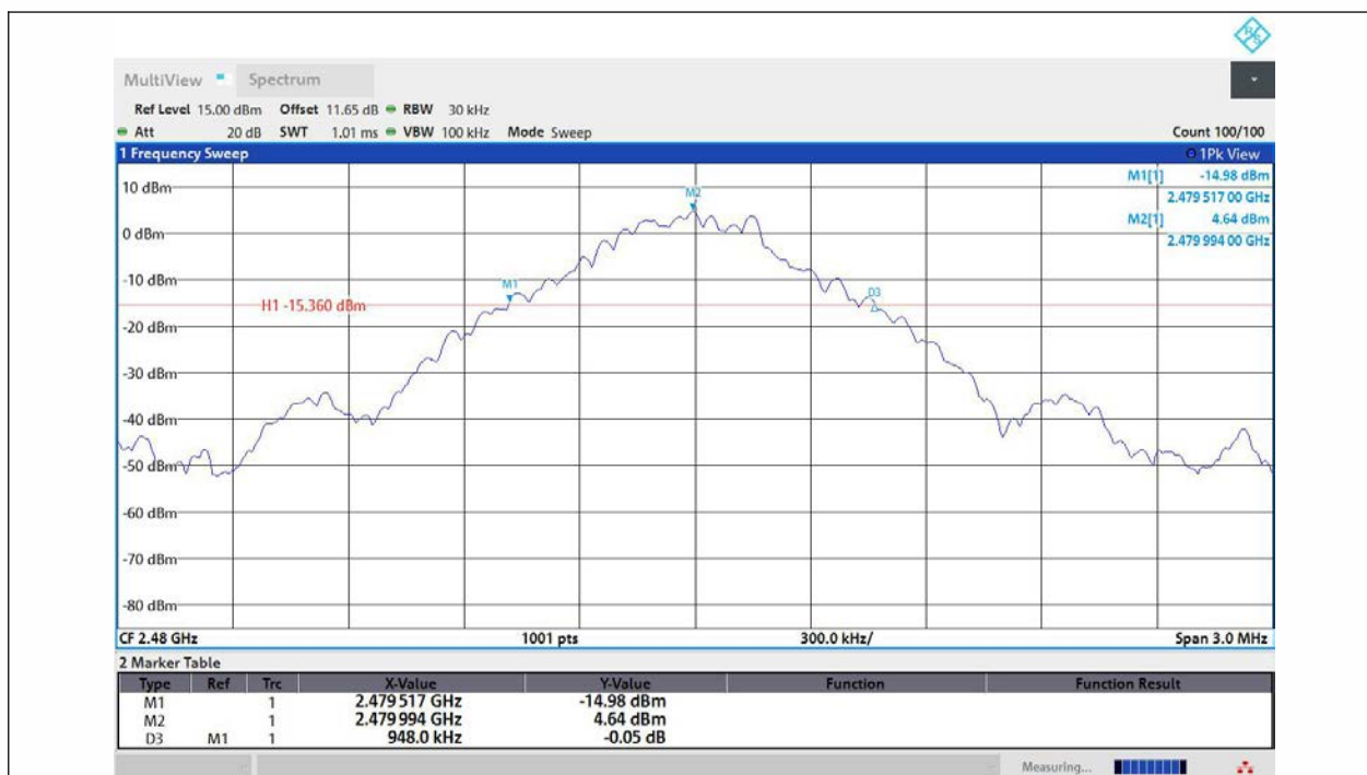
DH5-Ant1-2480
