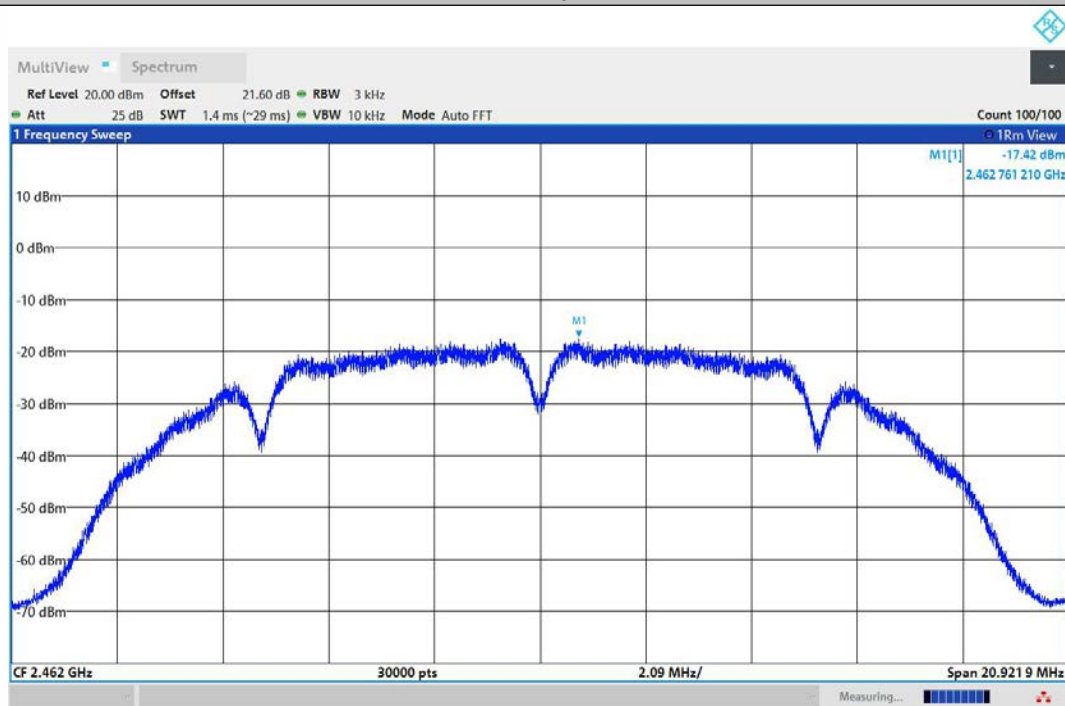
11B-Ant2-2462-PASS
