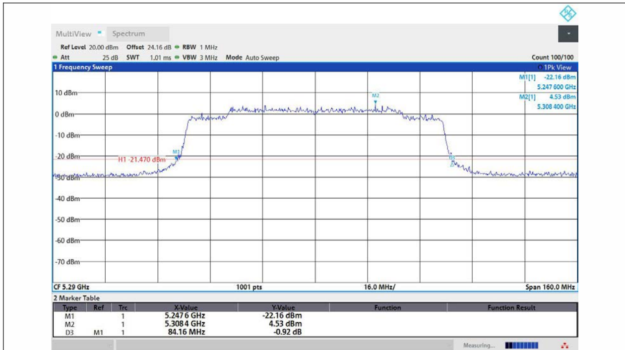
11AX80MIMO-Ant1-5290
