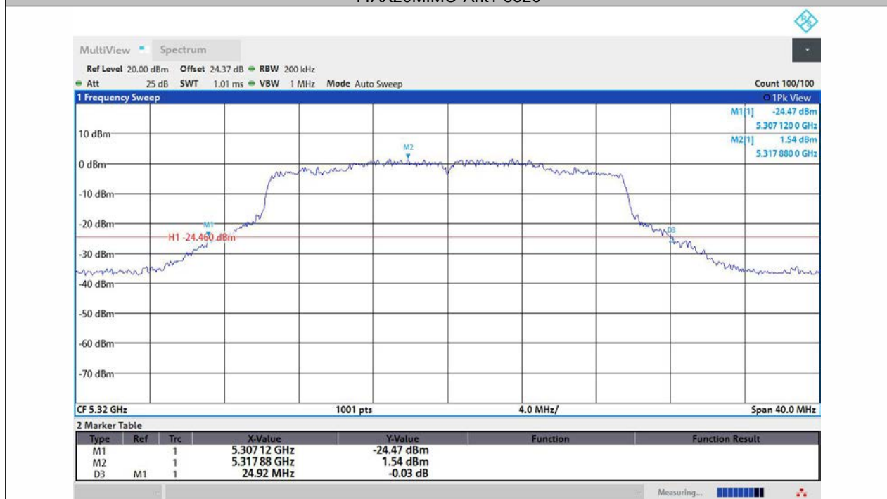
11AX20MIMO-Ant2-5320
