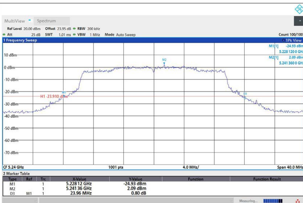
11AX20MIMO-Ant1-5240
