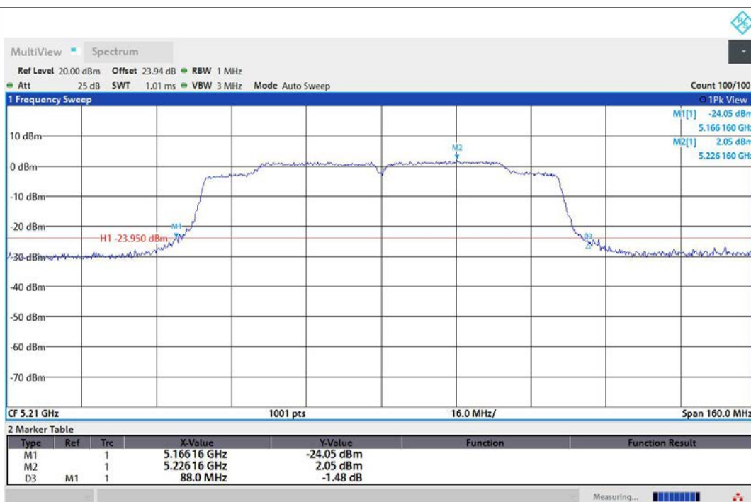
11AC80MIMO-Ant1-5210
