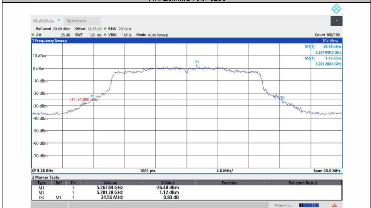
11AX20MIMO-Ant2-5280
