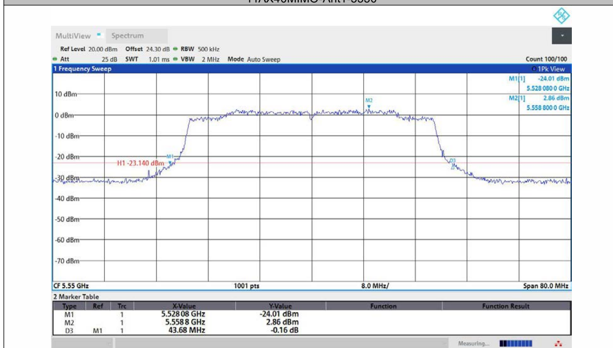
11AX40MIMO-Ant2-5550
