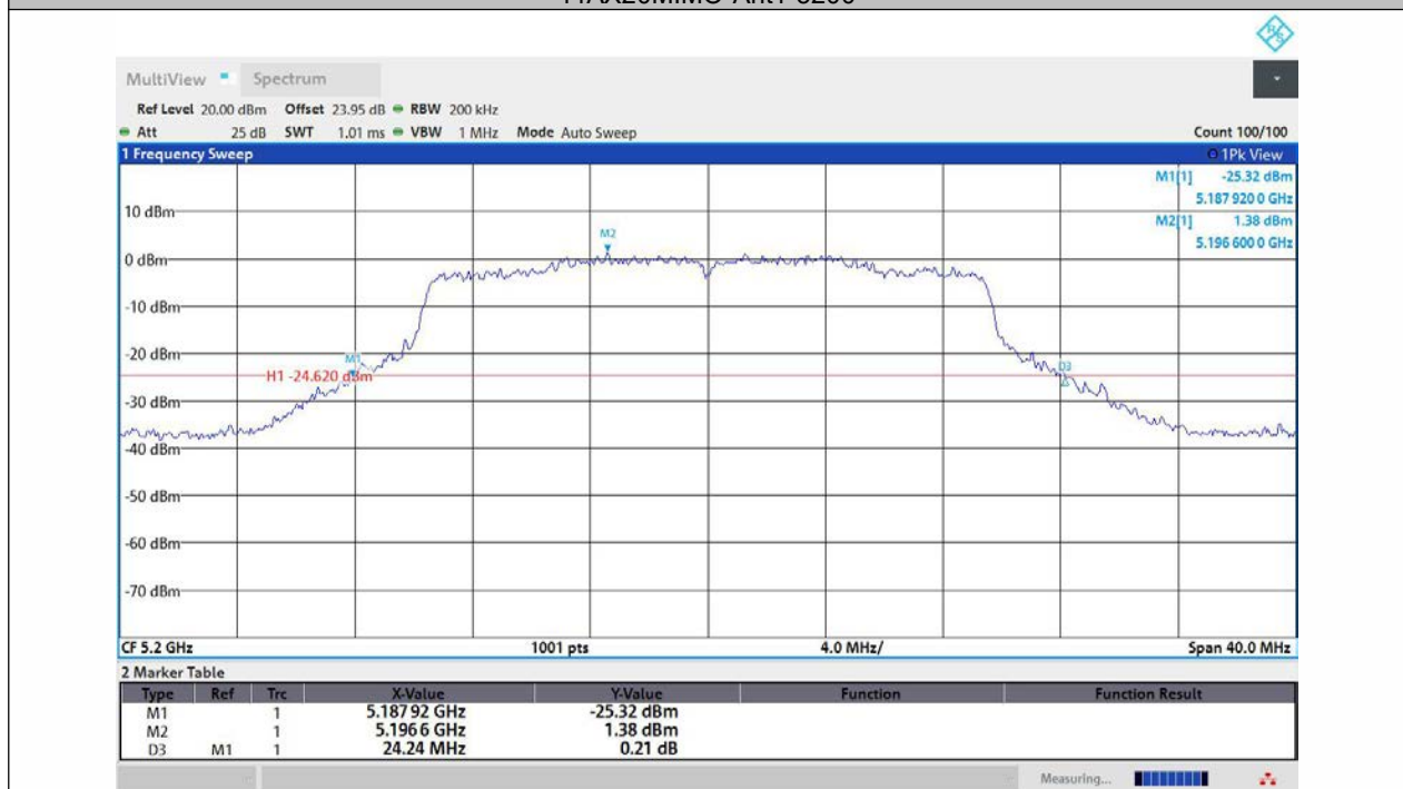
11AX20MIMO-Ant2-5200
