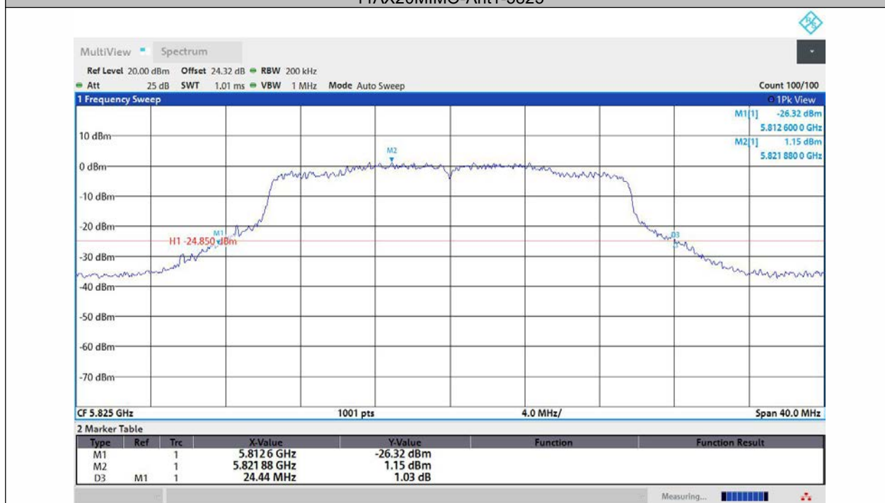
11AX20MIMO-Ant2-5825
