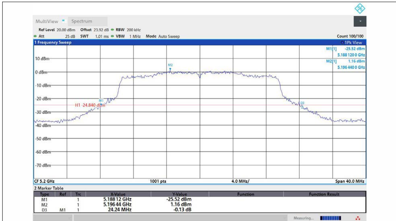
11AX20MIMO-Ant1-5200
