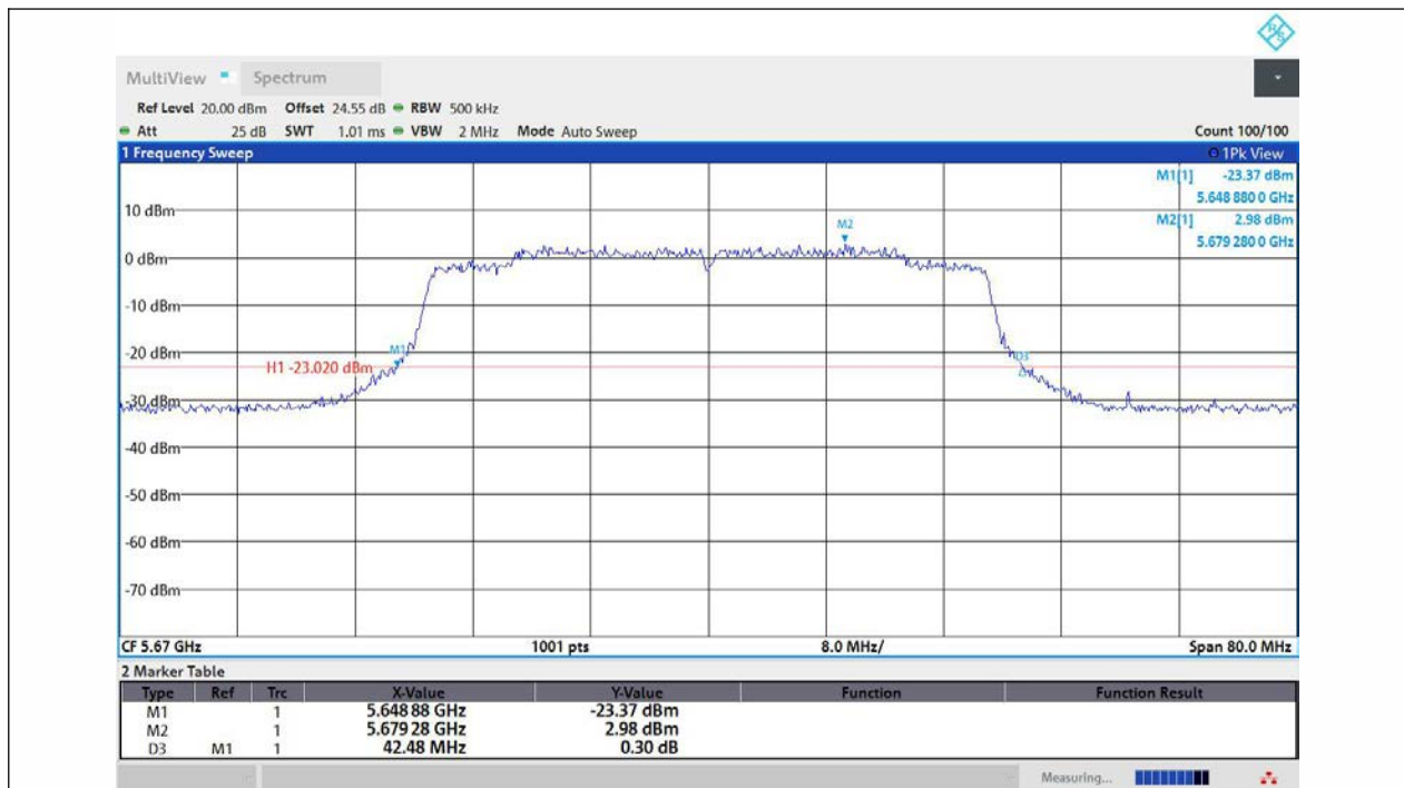
11AX40MIMO-Ant1-5670
