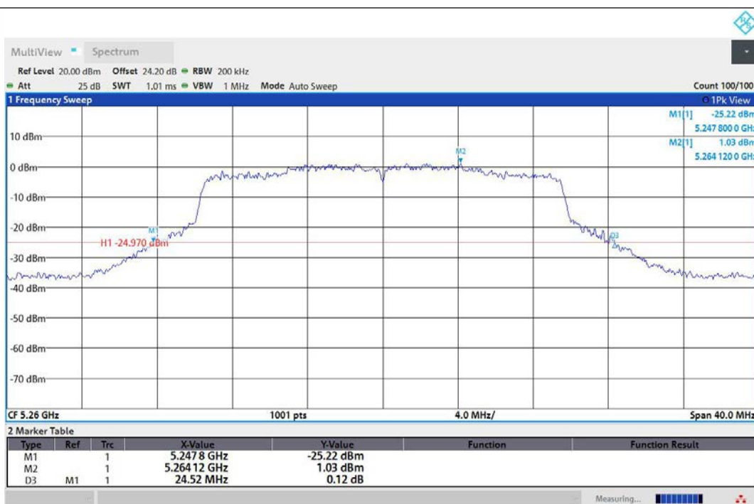
11AX20MIMO-Ant1-5260
