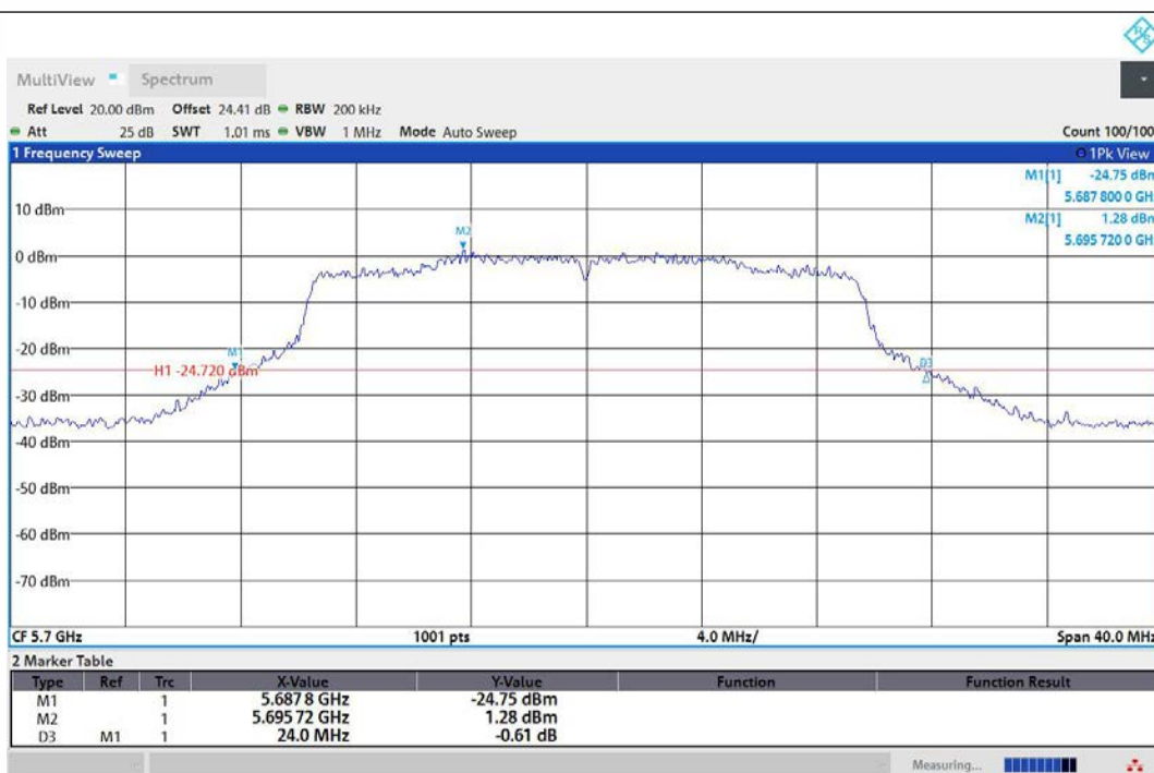
11AX20MIMO-Ant1-5700
