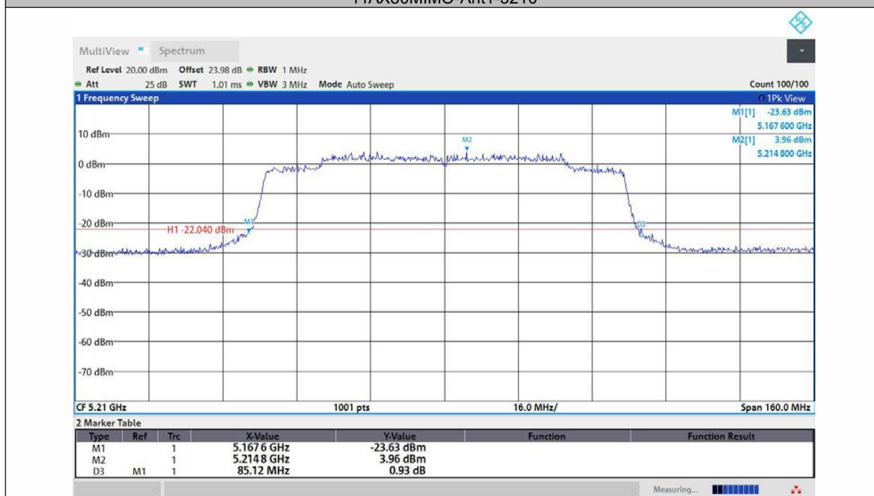
11AX80MIMO-Ant2-5210
