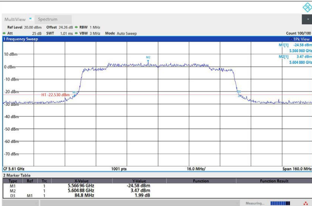
11AX80MIMO-Ant1-5610
