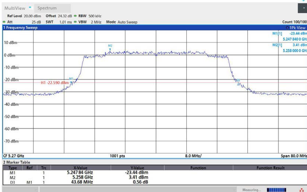
11AX40MIMO-Ant1-5270
