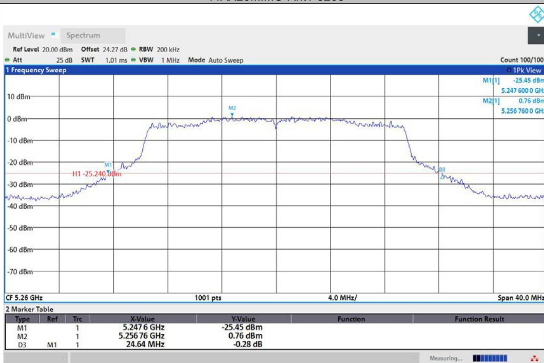
11AX20MIMO-Ant2-5260
