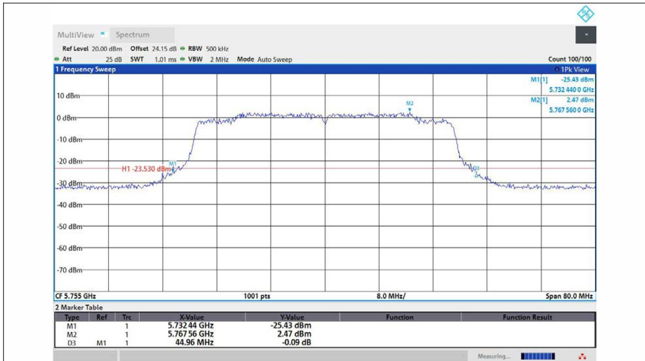
11AX40MIMO-Ant1-5755
