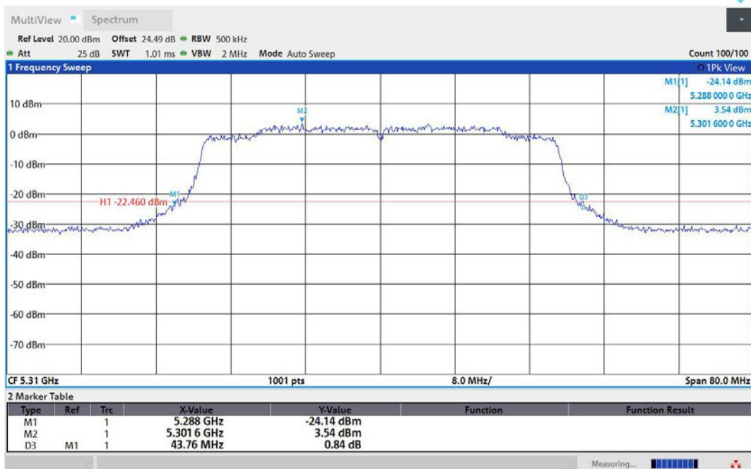
11AX40MIMO-Ant1-5310
