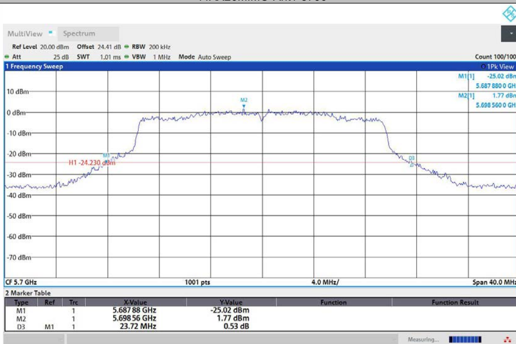
11AX20MIMO-Ant2-5700
