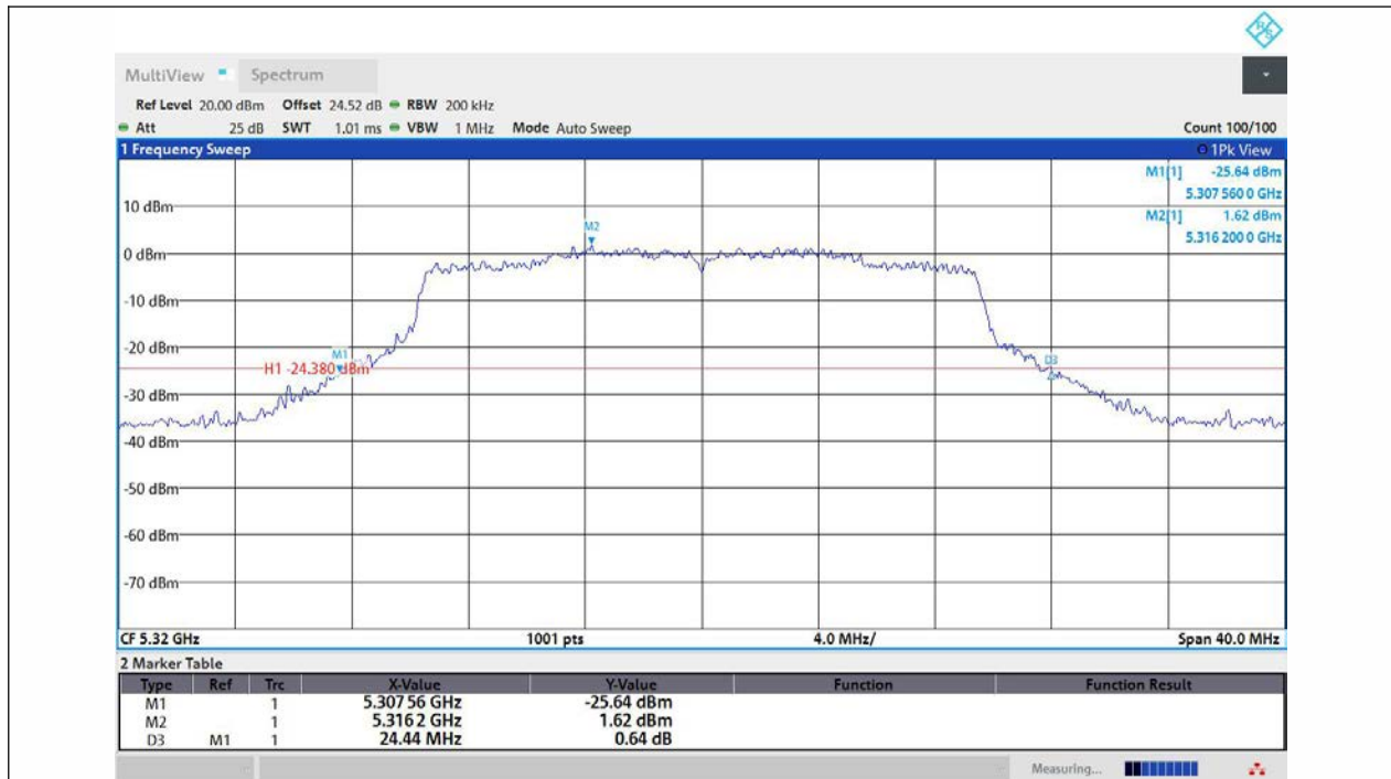
11AX20MIMO-Ant1-5320
