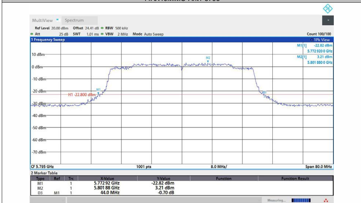
11AX40MIMO-Ant2-5795
