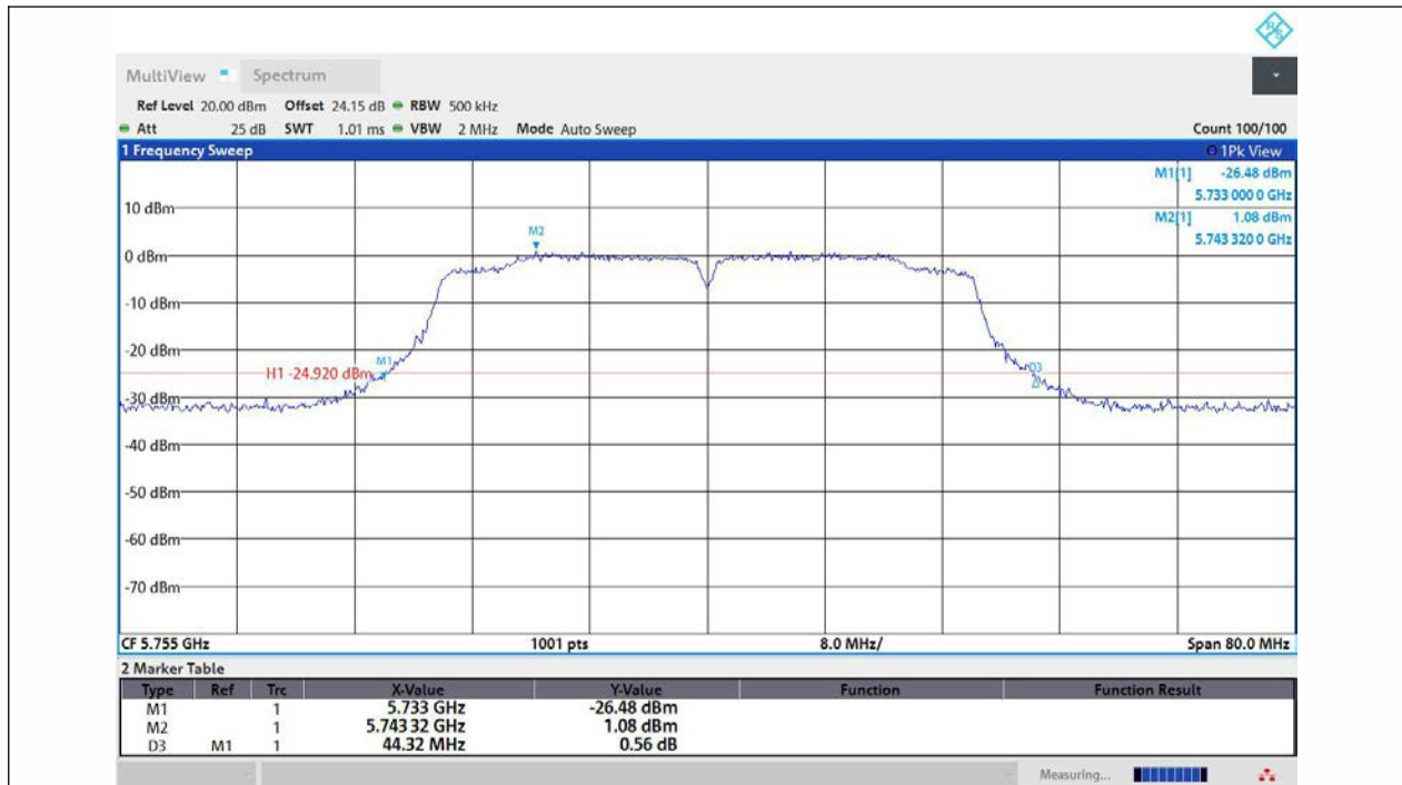
11AC40MIMO-Ant1-5755
