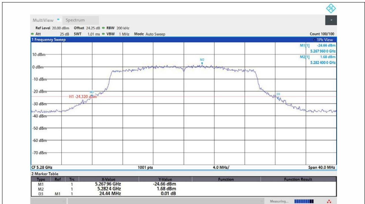
11AX20MIMO-Ant1-5280
