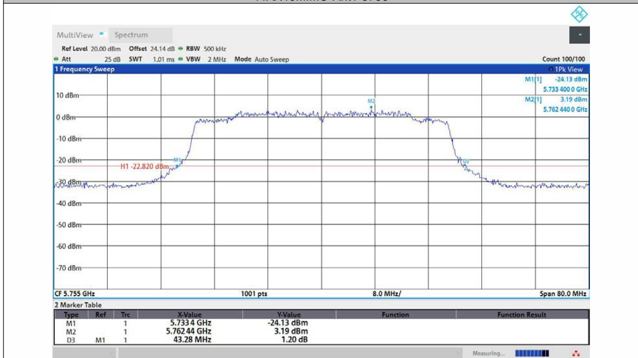
11AX40MIMO-Ant2-5755
