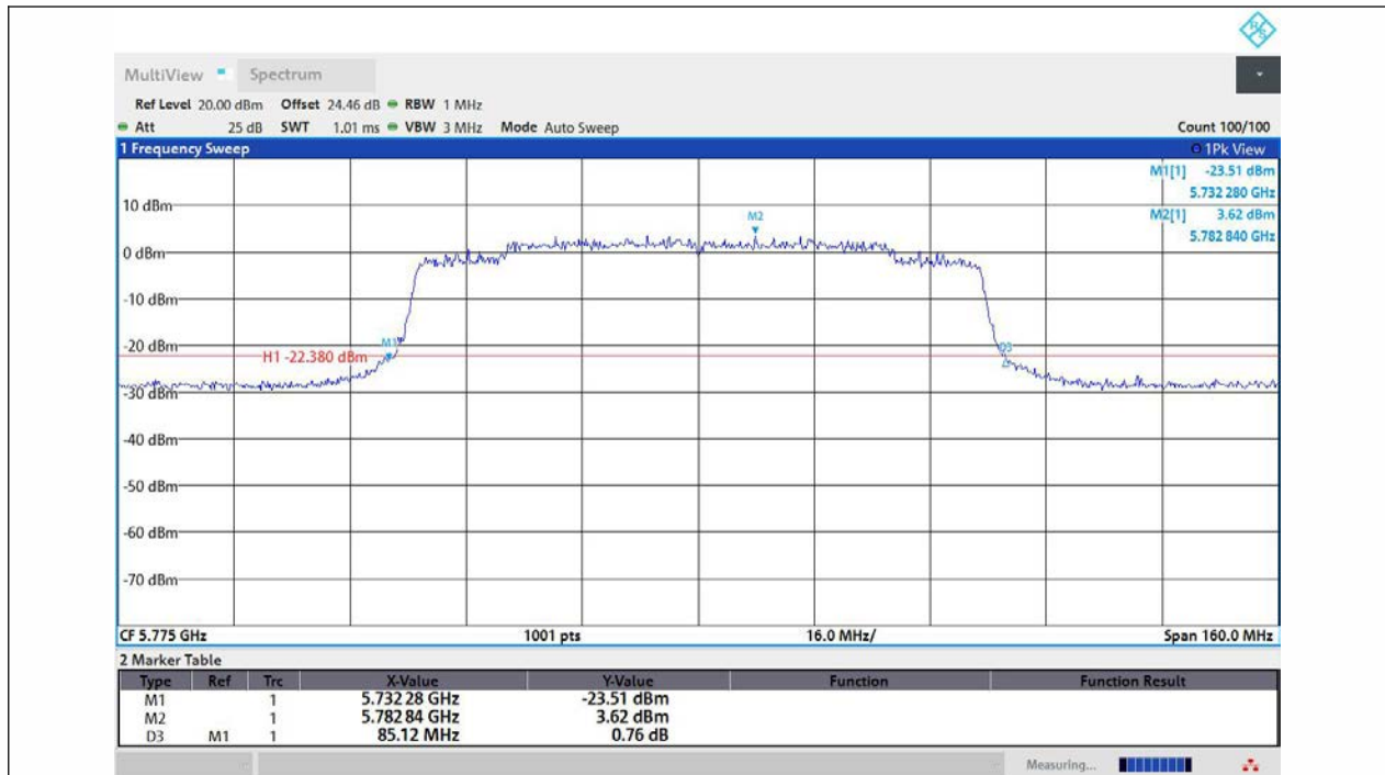
11AX80MIMO-Ant1-5775
