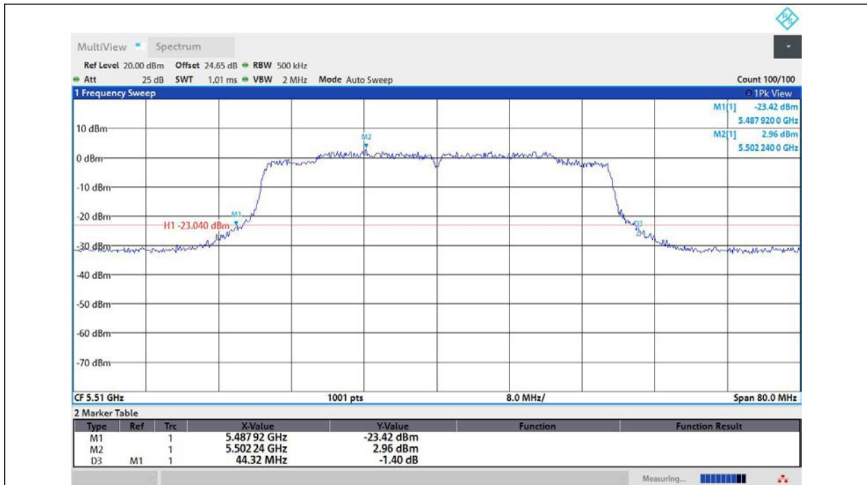
11AX40MIMO-Ant1-5510
