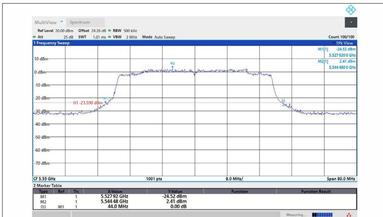
11AX40MIMO-Ant1-5550
