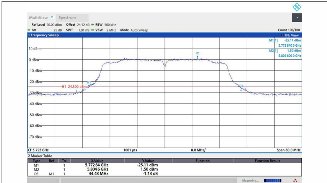
11AC40MIMO-Ant1-5795
