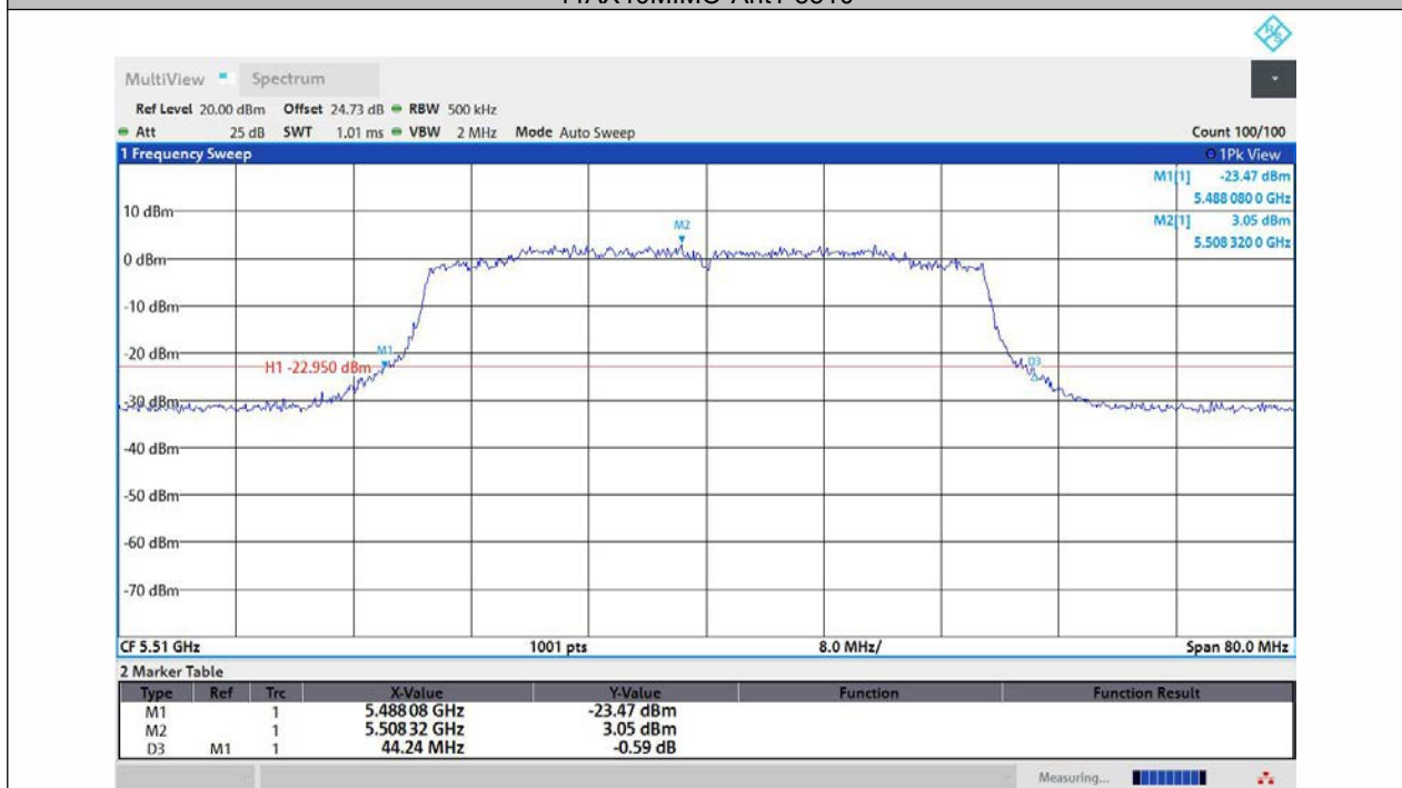
11AX40MIMO-Ant2-5510
