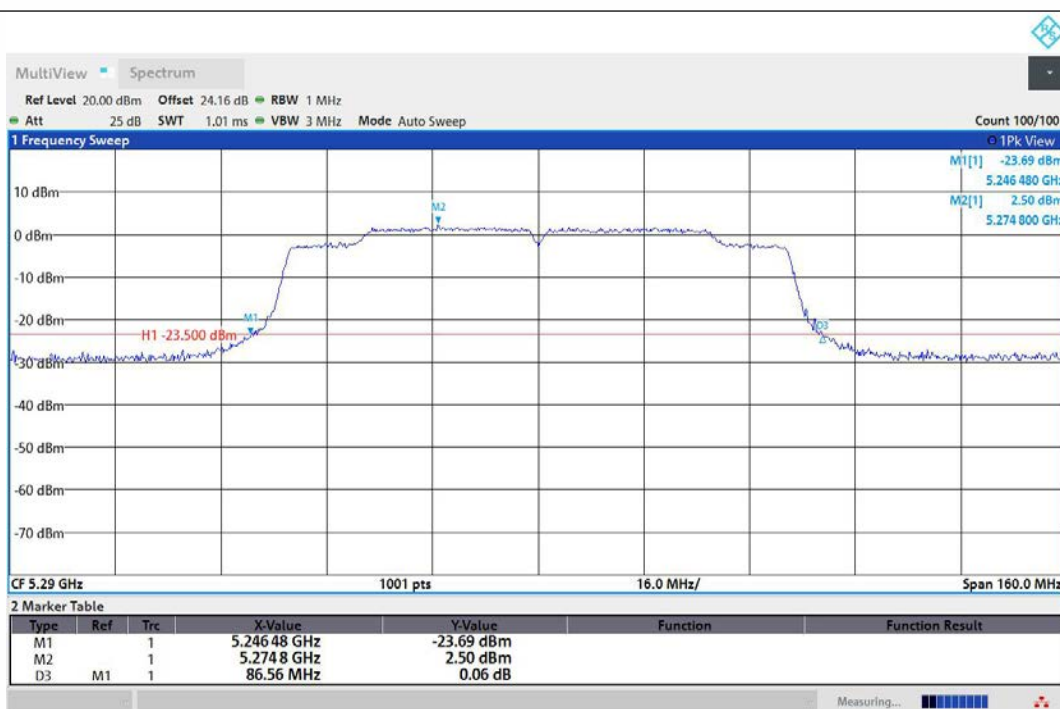
11AC80MIMO-Ant1-5290
