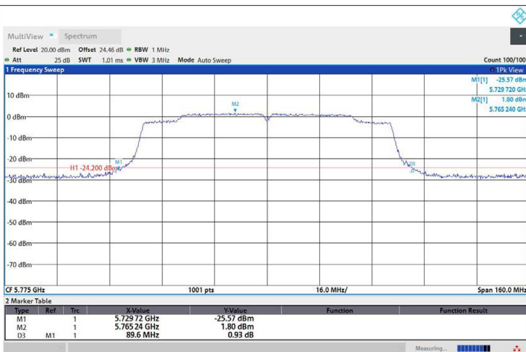
11AC80MIMO-Ant1-5775
