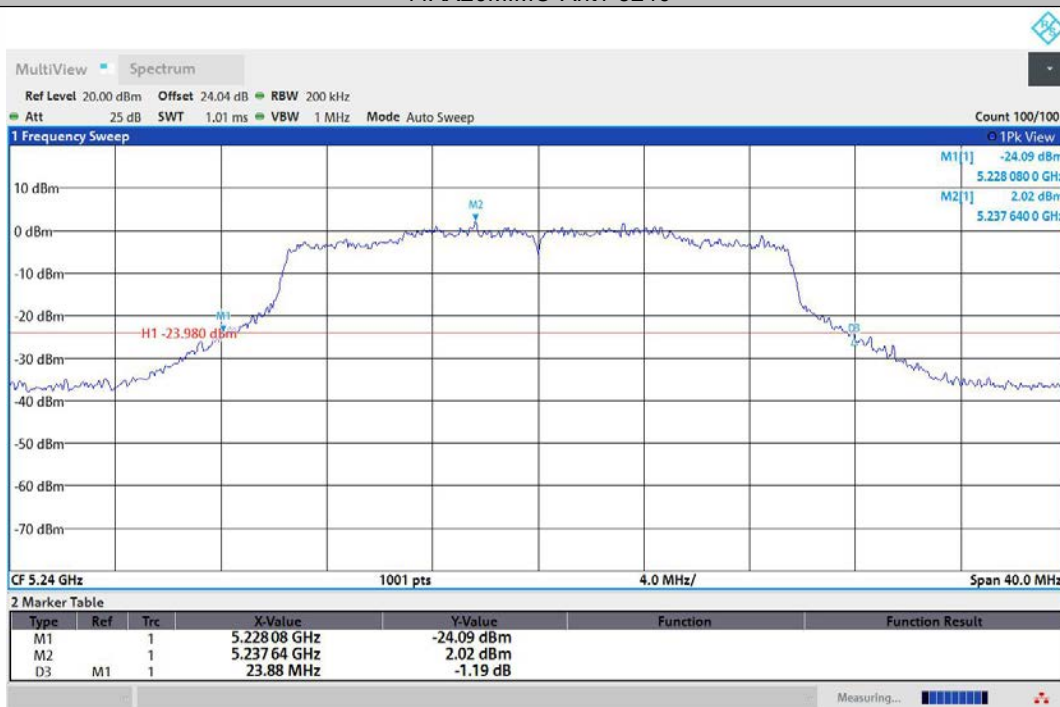
11AX20MIMO-Ant2-5240
