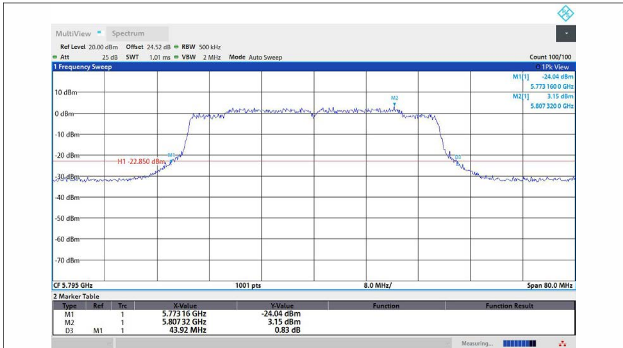
11AX40MIMO-Ant1-5795
