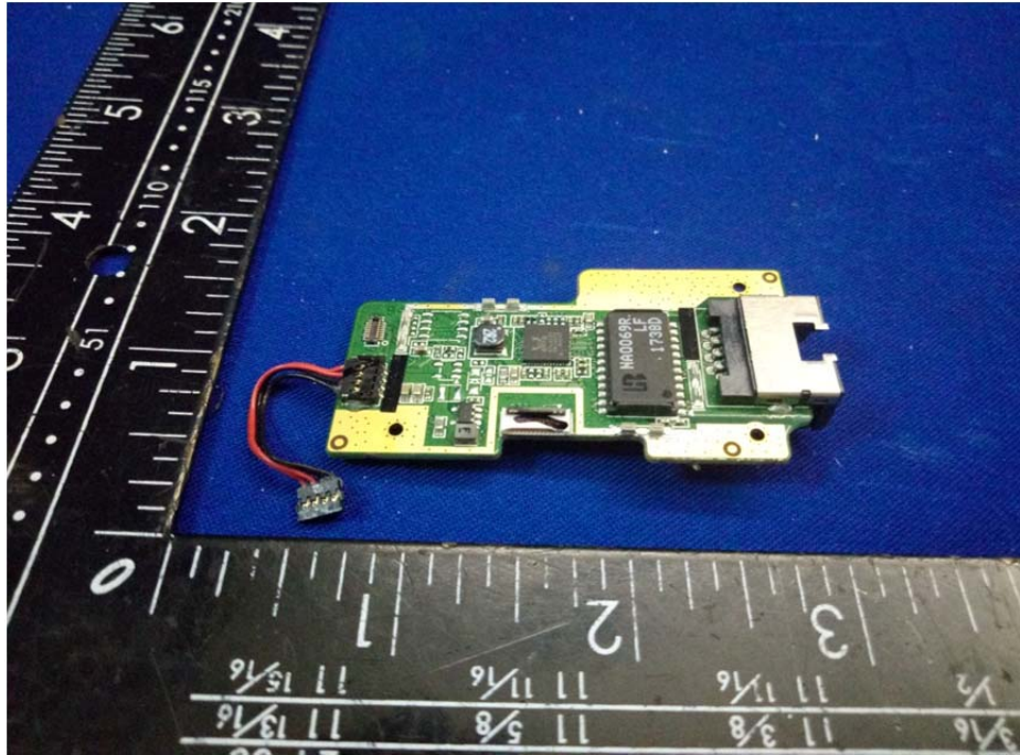
NFC Module
