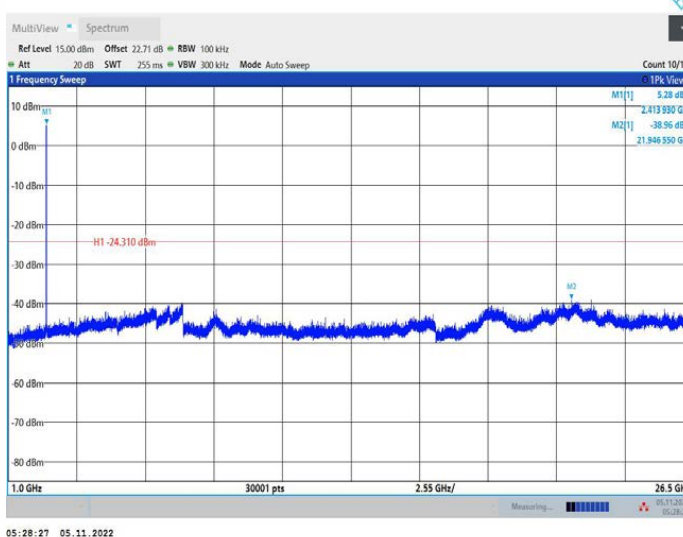
11B_Ant1_2412_1000~26500
