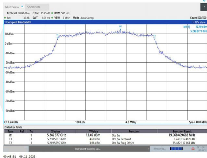
11AX20MIMO_Ant2_5240
