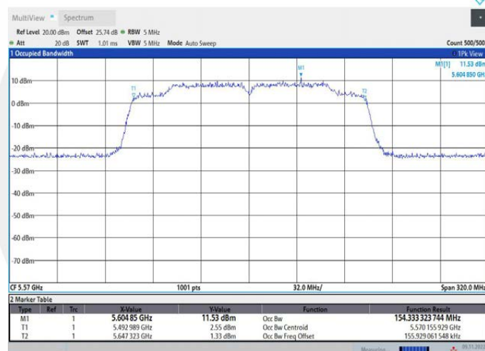
11AC160MIMO_Ant2_5570
