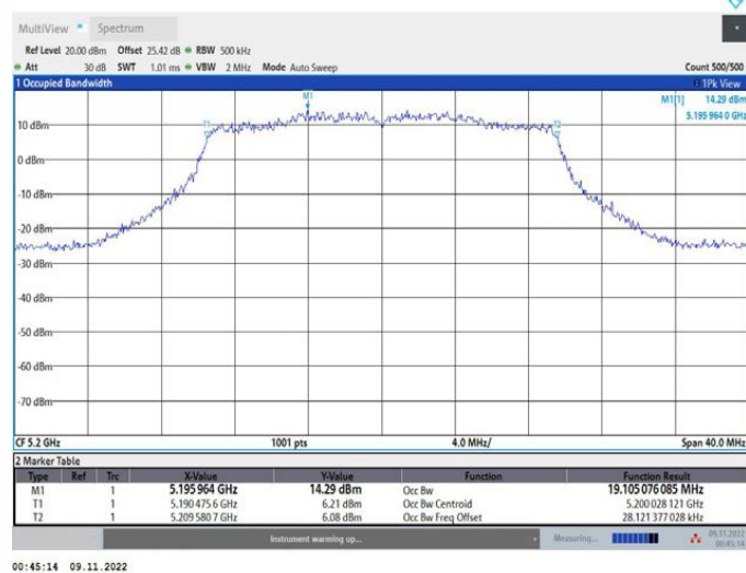
11AX20MIMO_Ant2_5200
