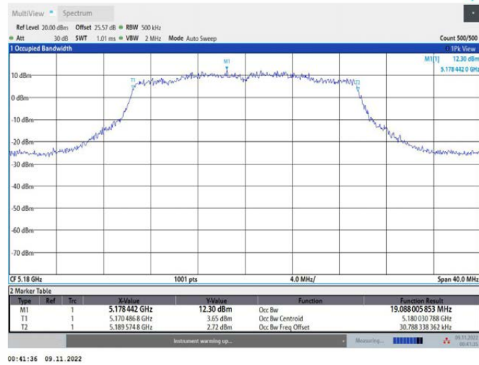
11AX20MIMO_Ant2_5180
