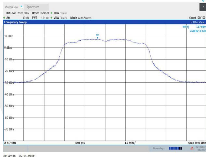
11A_Ant2_5700
