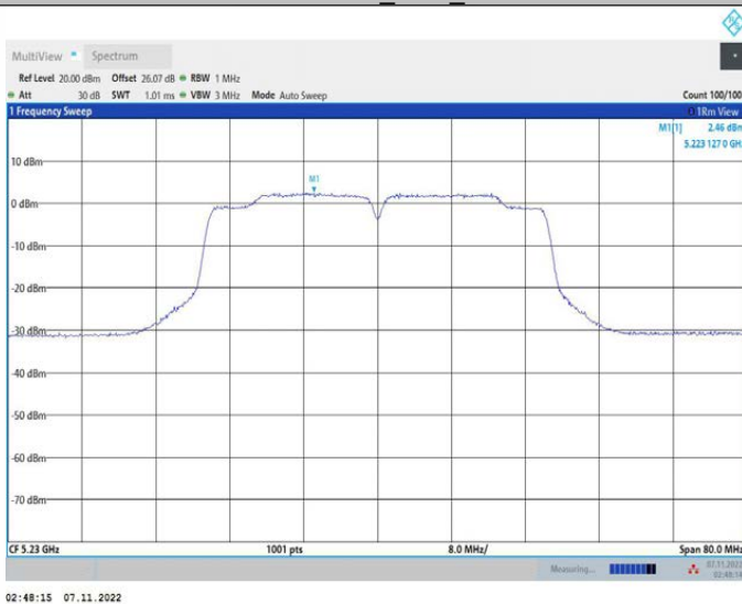
11N40MIMO_Ant2_5230
