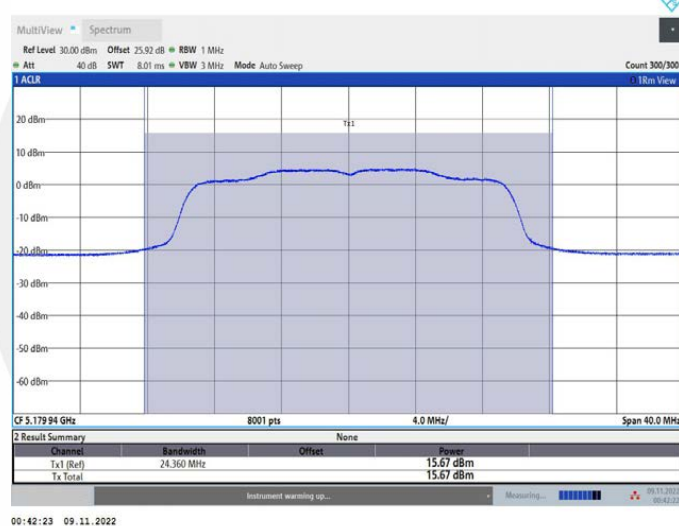
11AX20MIMO_Ant2_5180
