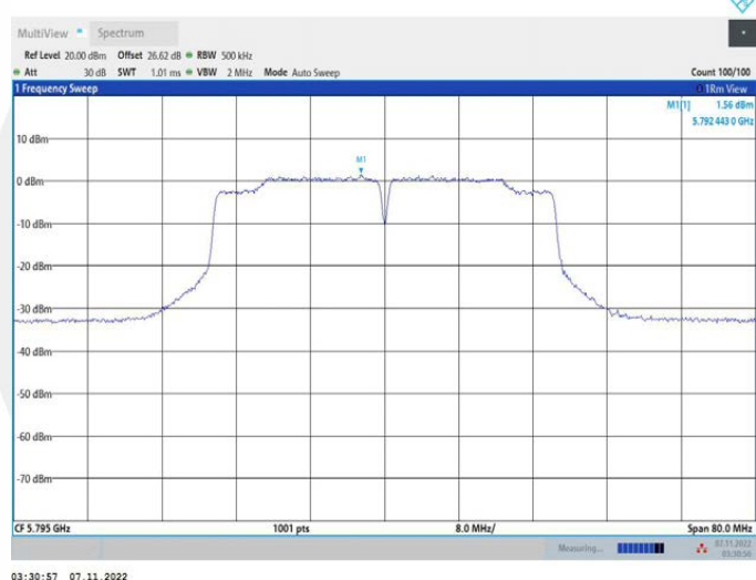
11N40MIMO_Ant2_5795
