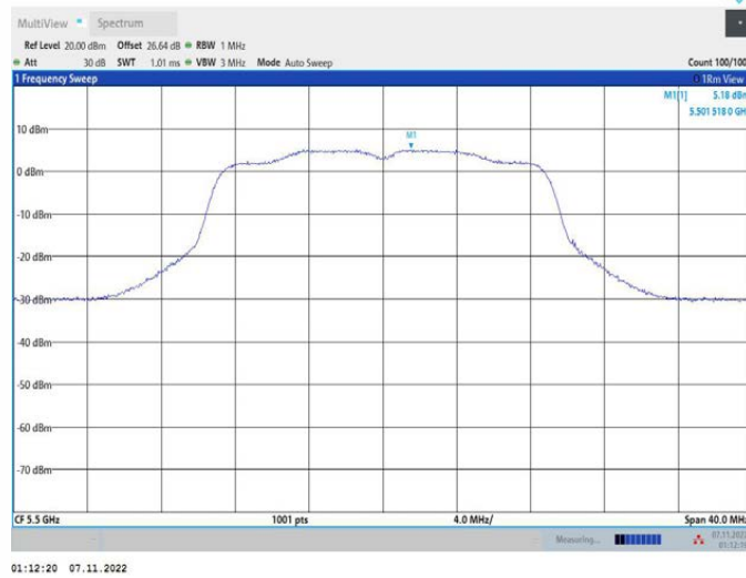
11N20MIMO_Ant2_5500
