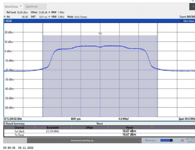
11AX20MIMO_Ant1_5240
