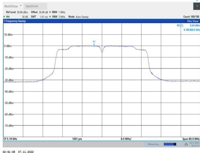
11N40MIMO_Ant2_5190
