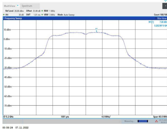
11N20MIMO_Ant2_5200
