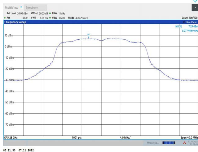
11AC20MIMO_Ant2_5280
