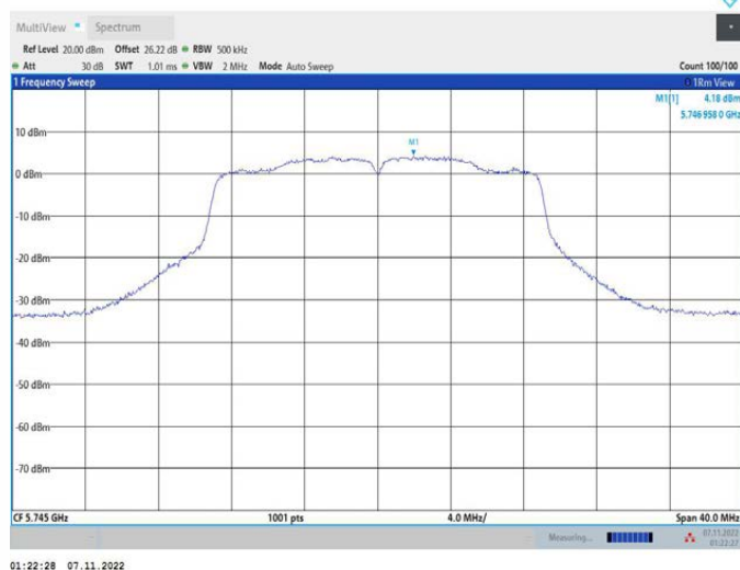
11N20MIMO_Ant2_5745
