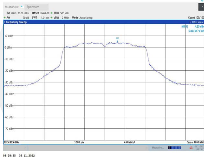
11A_Ant2_5825
