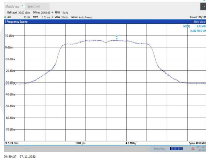
11N20MIMO_Ant2_5240
