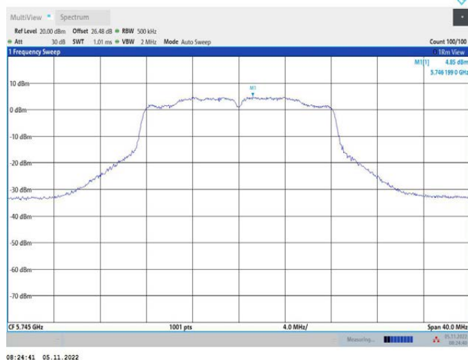
11A_Ant2_5745
