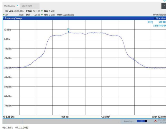
11N20MIMO_Ant2_5580
