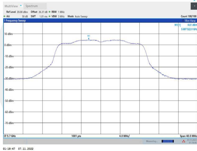
11N20MIMO_Ant2_5700
