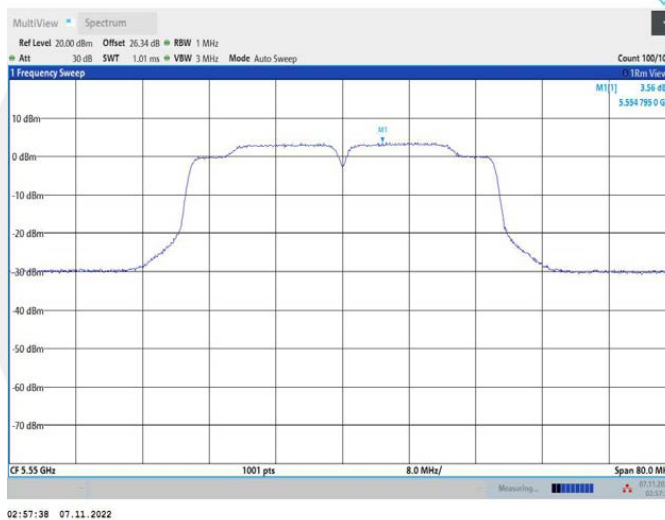
11N40MIMO_Ant2_5550
