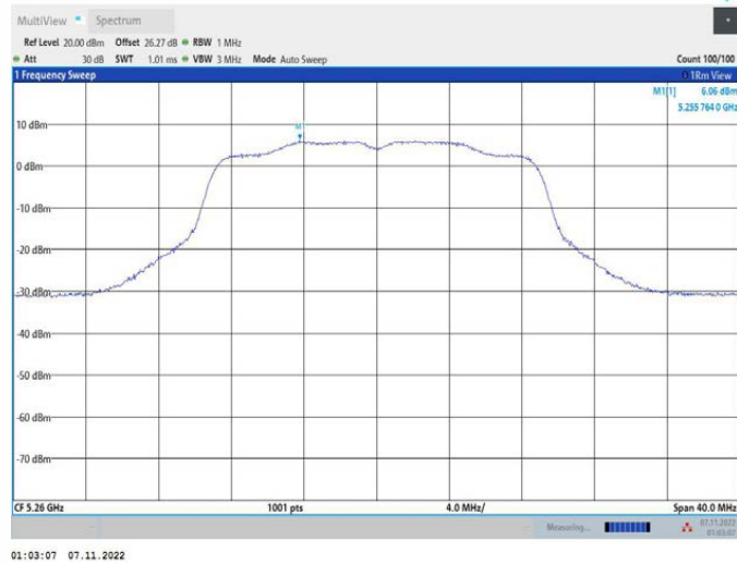
11N20MIMO_Ant2_5260
