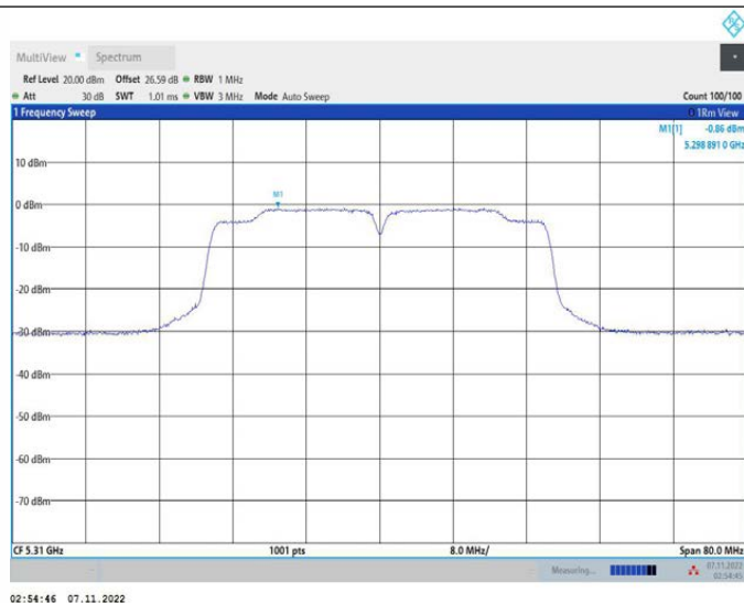
11N40MIMO_Ant2_5310
