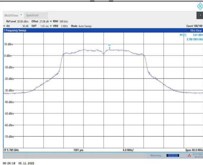
11A_Ant2_5785
