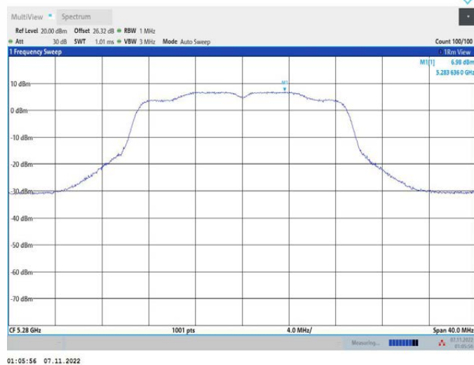
11N20MIMO_Ant2_5280
