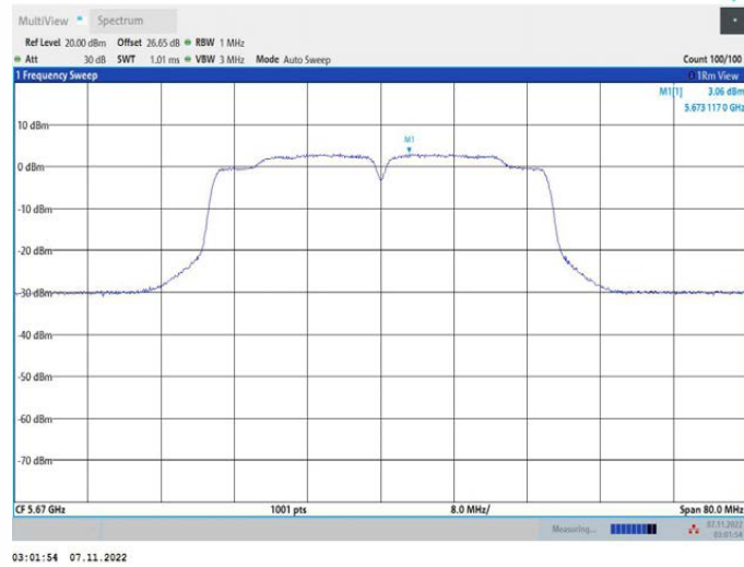
11N40MIMO_Ant2_5670
