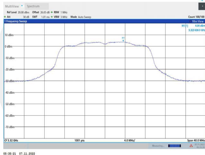
11AC20MIMO_Ant2_5320
