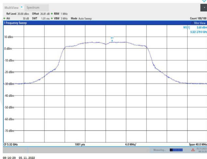
11A_Ant2_5320
