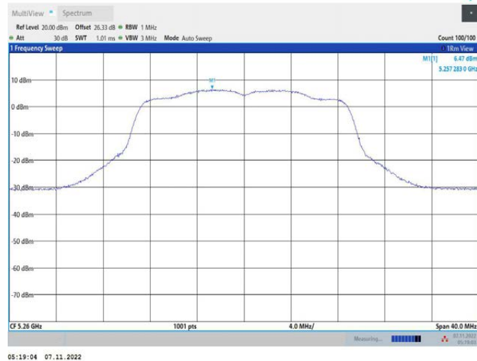
11AC20MIMO_Ant2_5260
