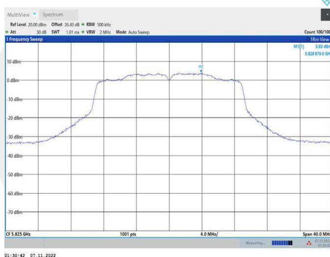
11N20MIMO_Ant2_5825
