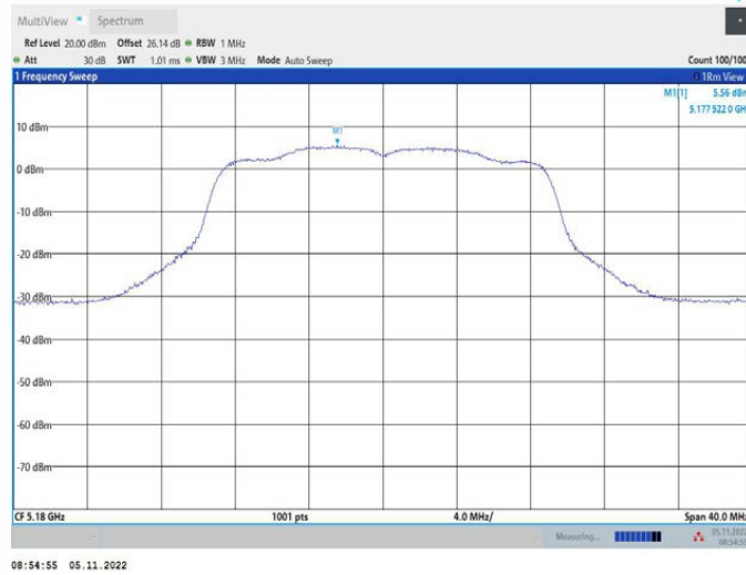
11N20MIMO_Ant2_5180
