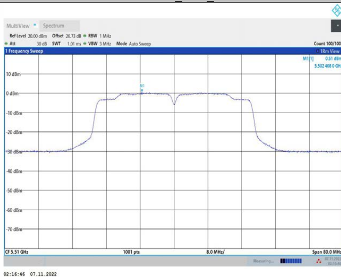
11N40MIMO_Ant2_5510
