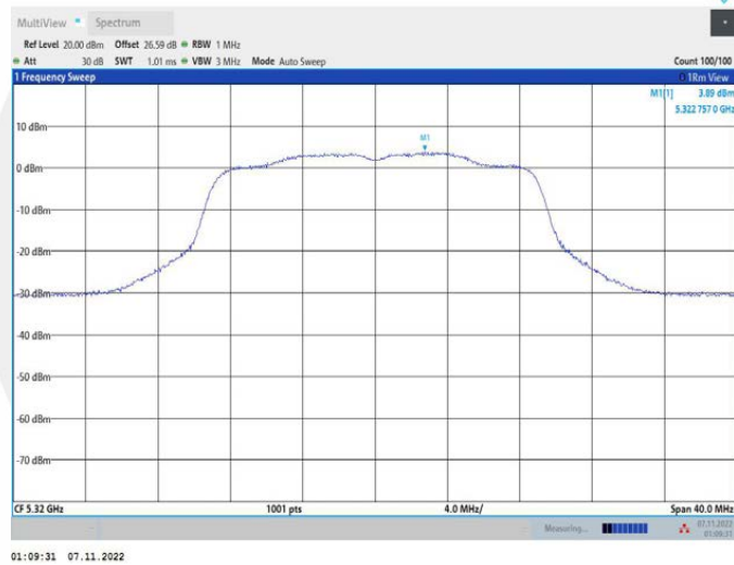
11N20MIMO_Ant2_5320
