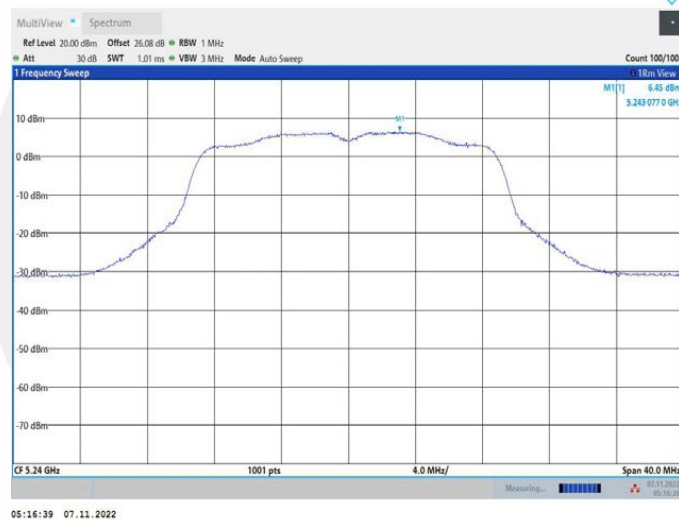
11AC20MIMO_Ant2_5240
