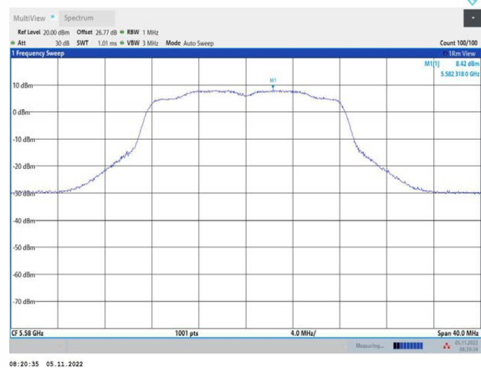
11A_Ant2_5580
