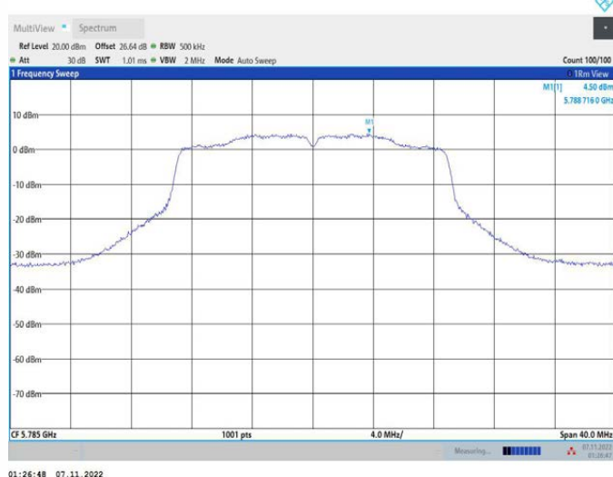
11N20MIMO_Ant2_5785
