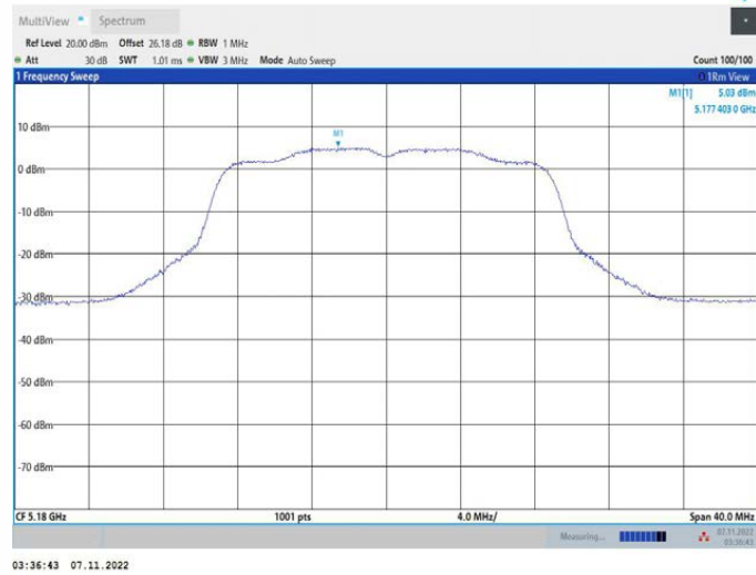
11AC20MIMO_Ant2_5180
