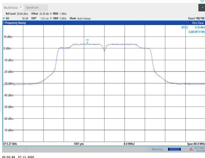
11N40MIMO_Ant2_5270
