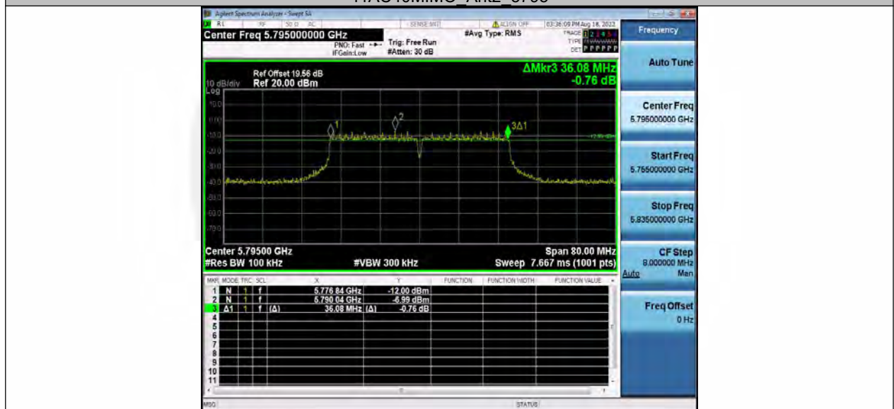
11AC80MIMO_Ant1_5775
