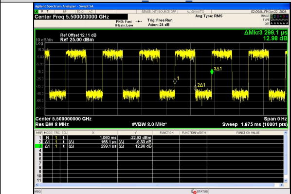
IEEE 802.11n 20MHz Channel 100
