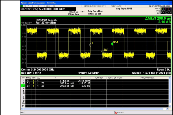
IEEE 802.11n 20MHz Channel 48
