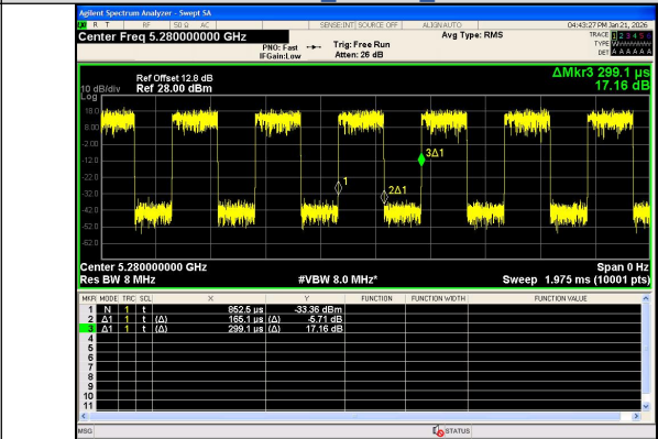
IEEE 802.11n 20MHz Channel 56
