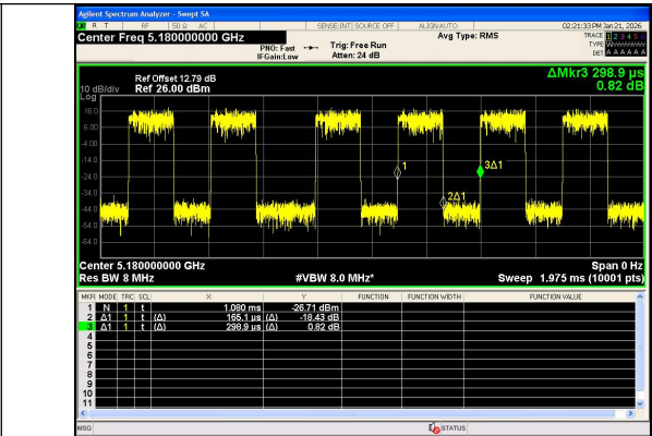
IEEE 802.11n 20MHz Channel 36
