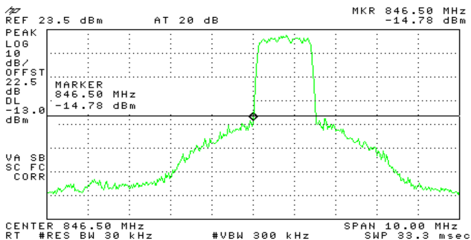
Middle block edge (2) 742
