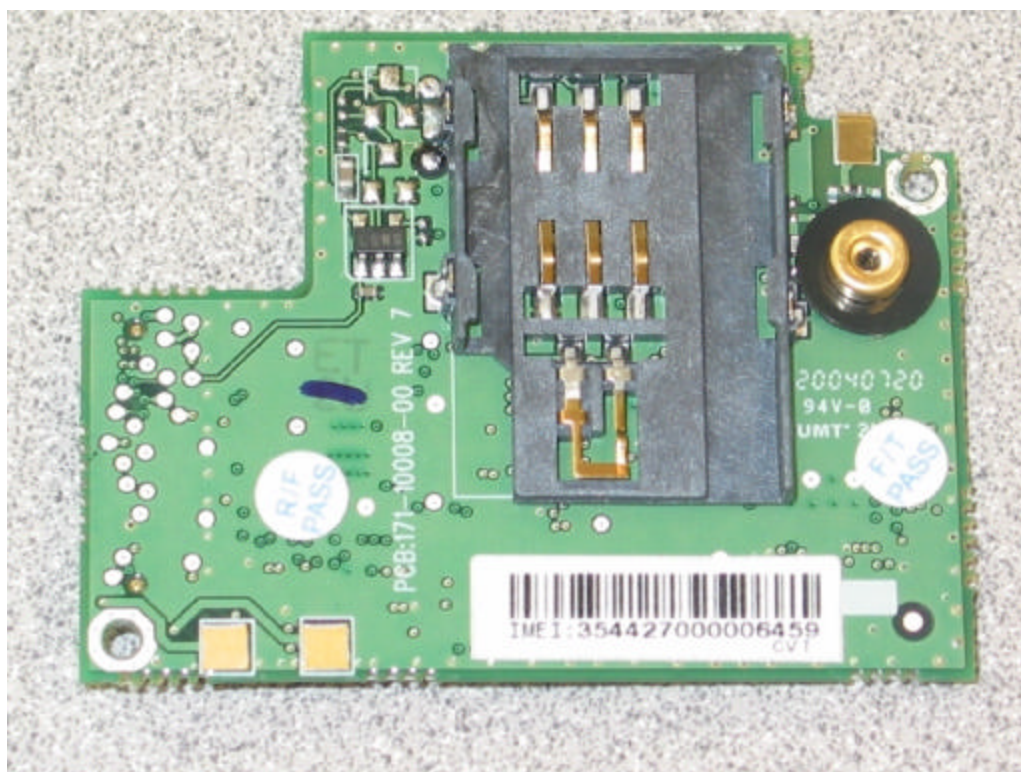
RF Module, SIM side
