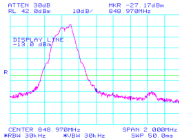
High block edge
