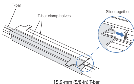
15.9-mm (5/8-in) T-bar
