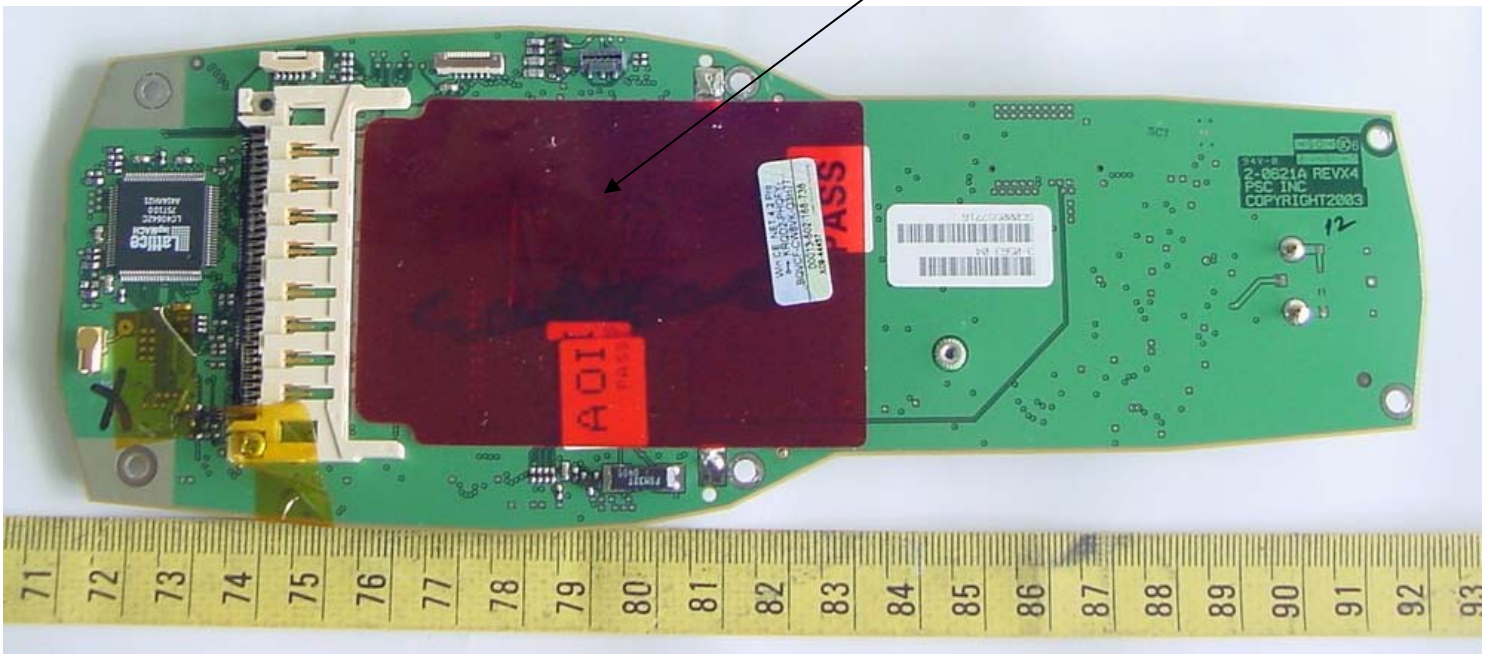
802.11b Antenna
