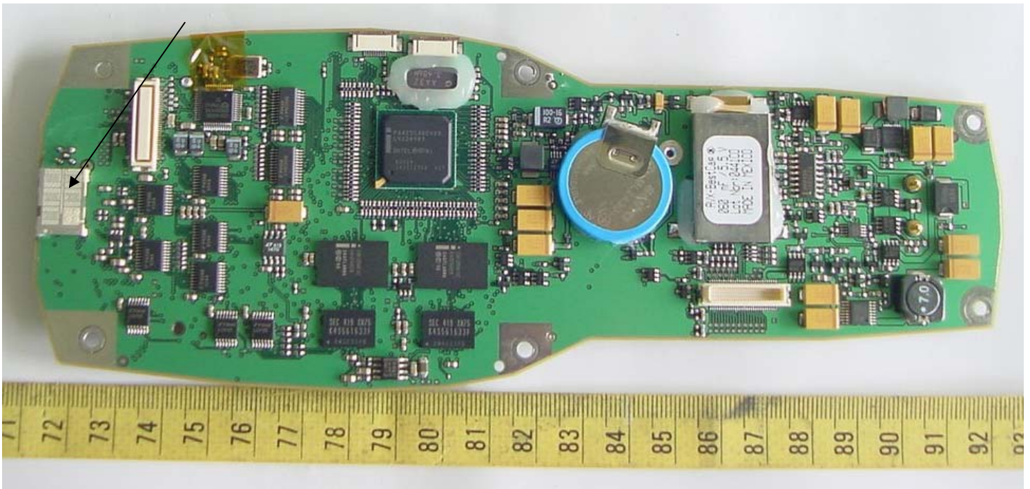
802.11b Antenna
