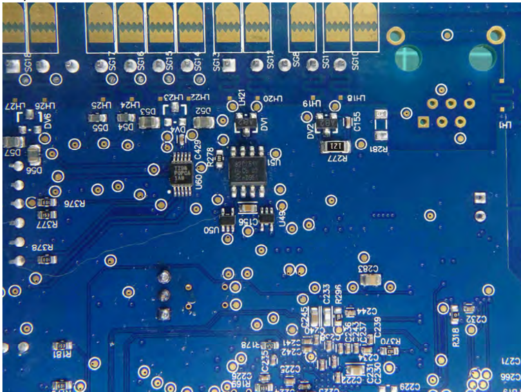
(195) EUT Photo
