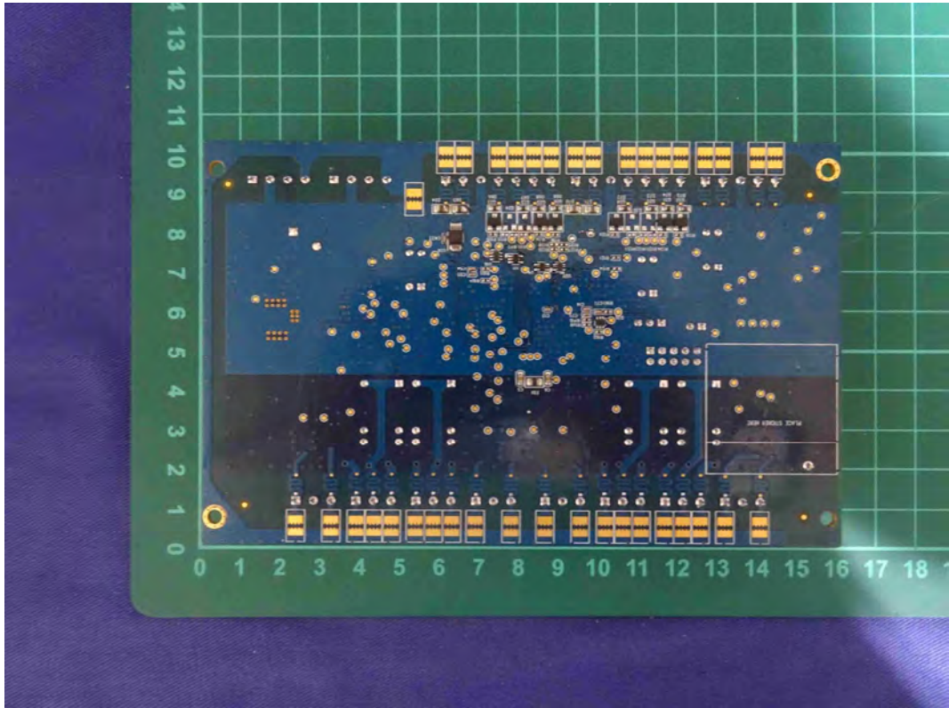
(200) EUT Photo
