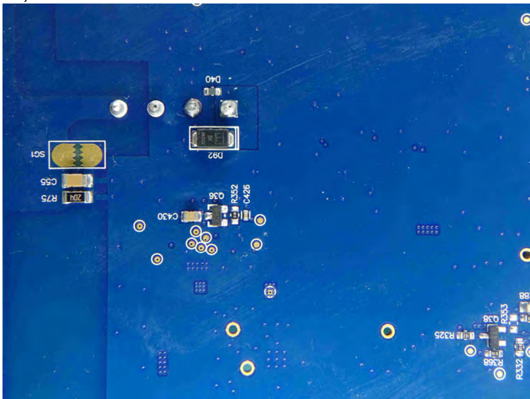
(196) EUT Photo
