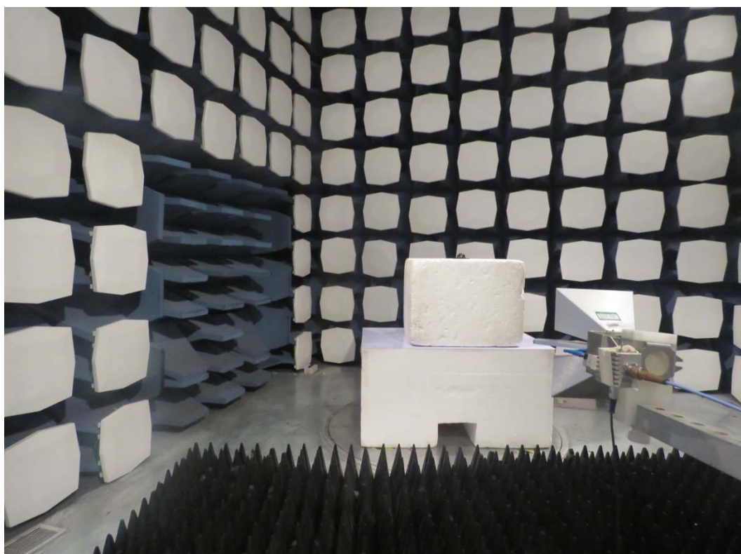
1GHz-18GHz
