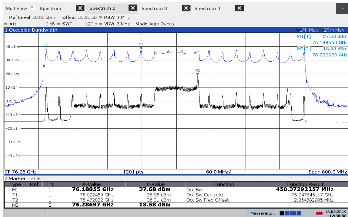
Plot 30: Mode 8, OBW, T_{\text{nom}} / V_{\text{nom}}
