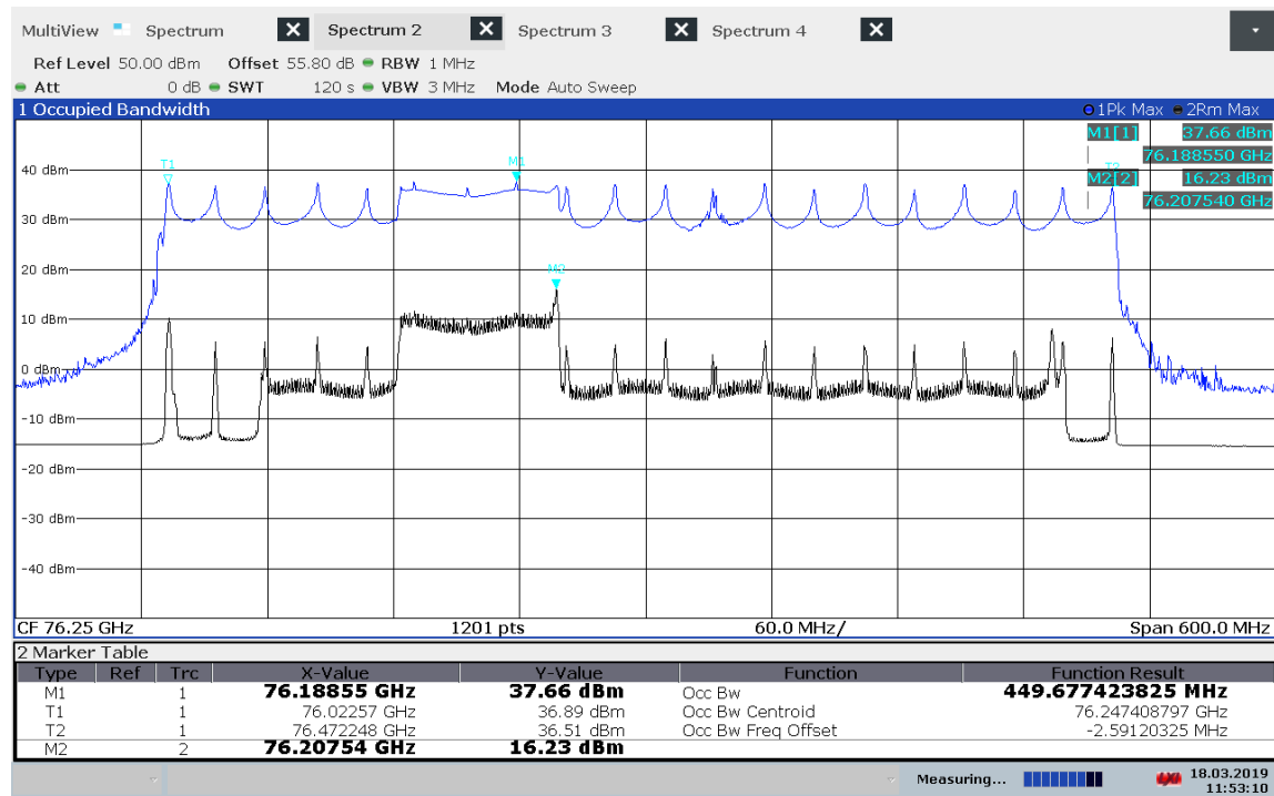
Plot 29: Mode 7, OBW, T_{\text{nom}} / V_{\text{nom}}
