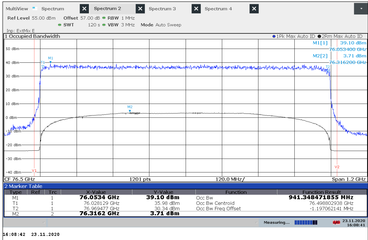
Plot 37: Mode 3, OBW, -30^{\circ}\text{C} / V_{\text{nom}}
