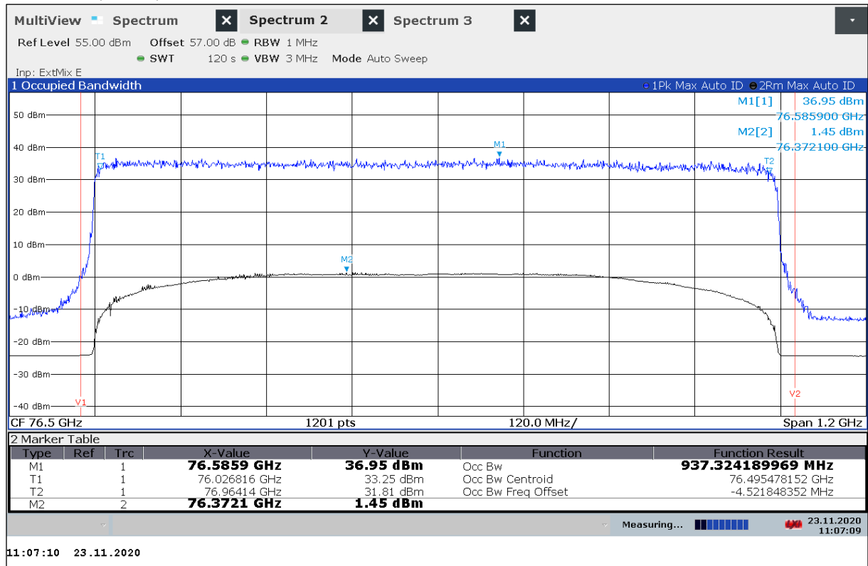
Plot 46: Mode 3, OBW, T_{\max} / V_{\text{nom}}
