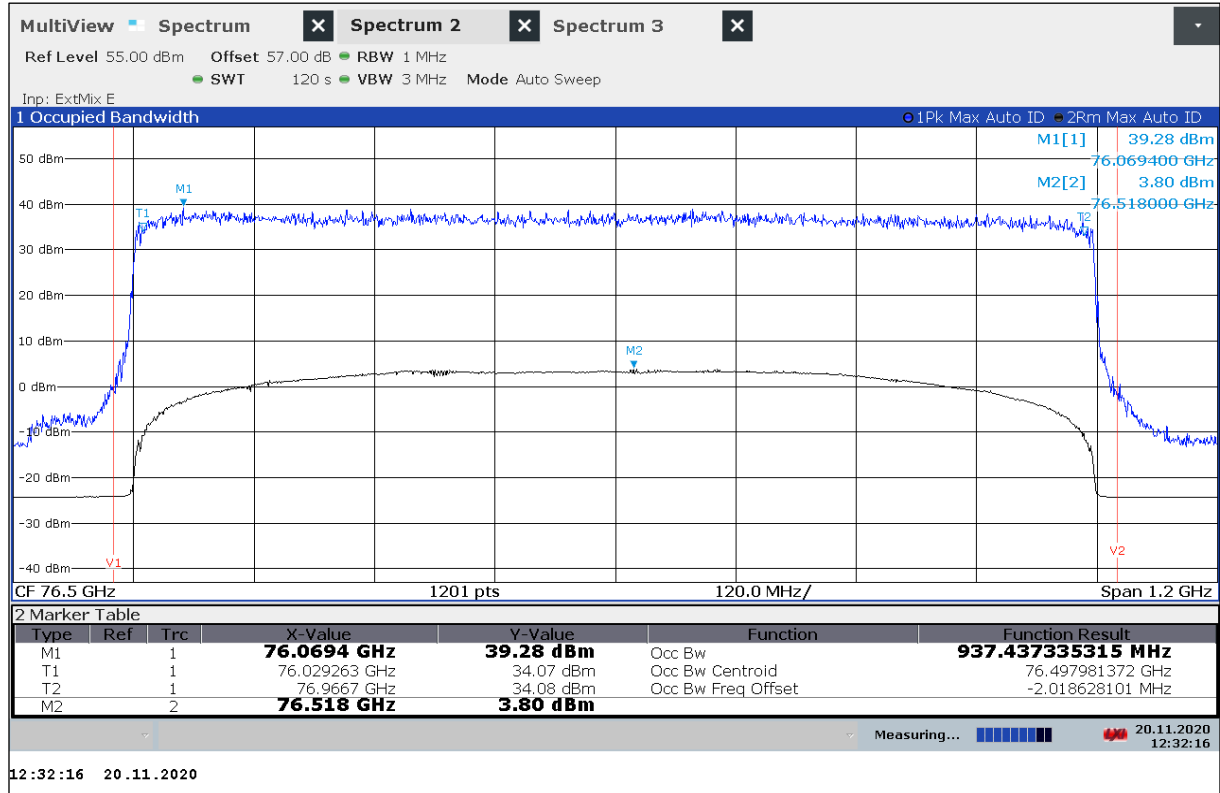
Plot 36: Mode 3, OBW, T_{\min} / V_{\text{nom}}
