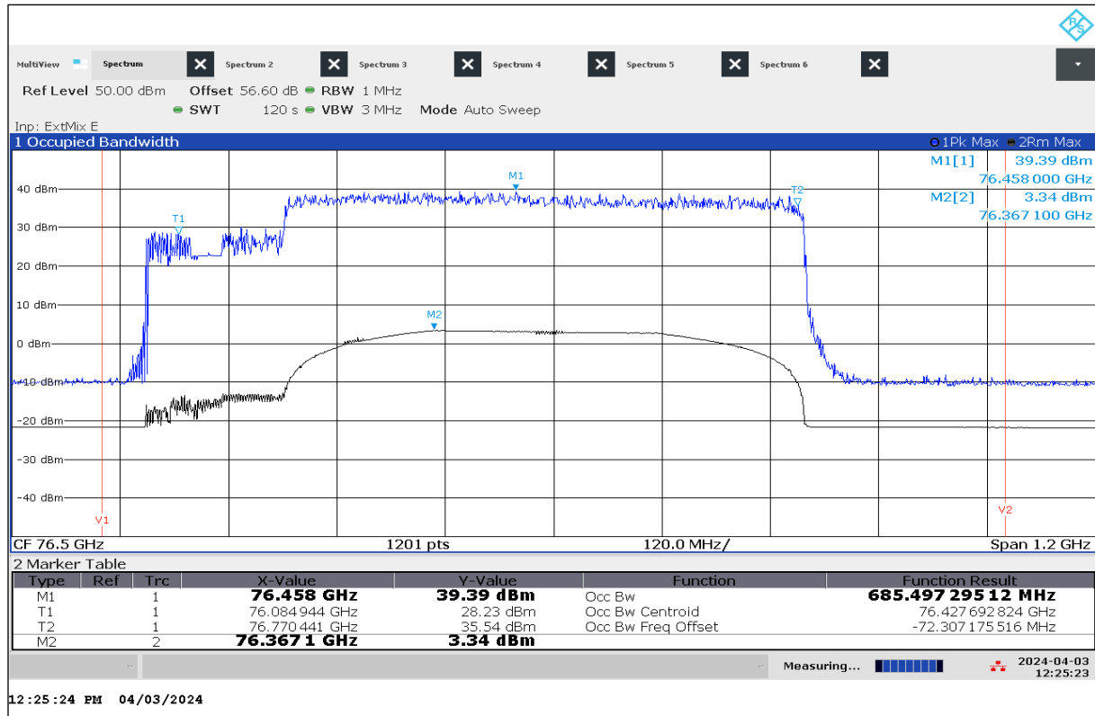
Plot 15: OBW, Mode 27, T_{\text{nom}} / V_{\text{nom}}
