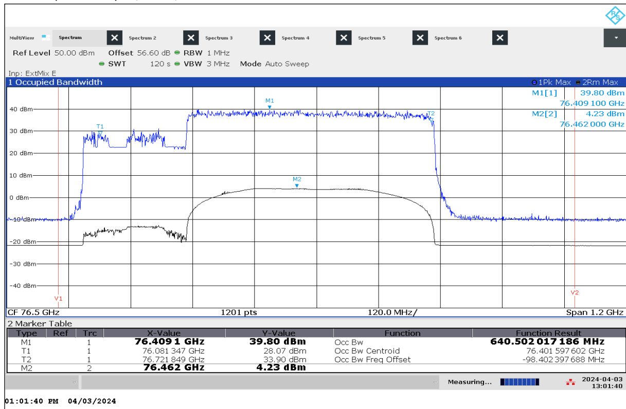
Plot 16: OBW, Mode 39, T_{\text{nom}} / V_{\text{nom}}
