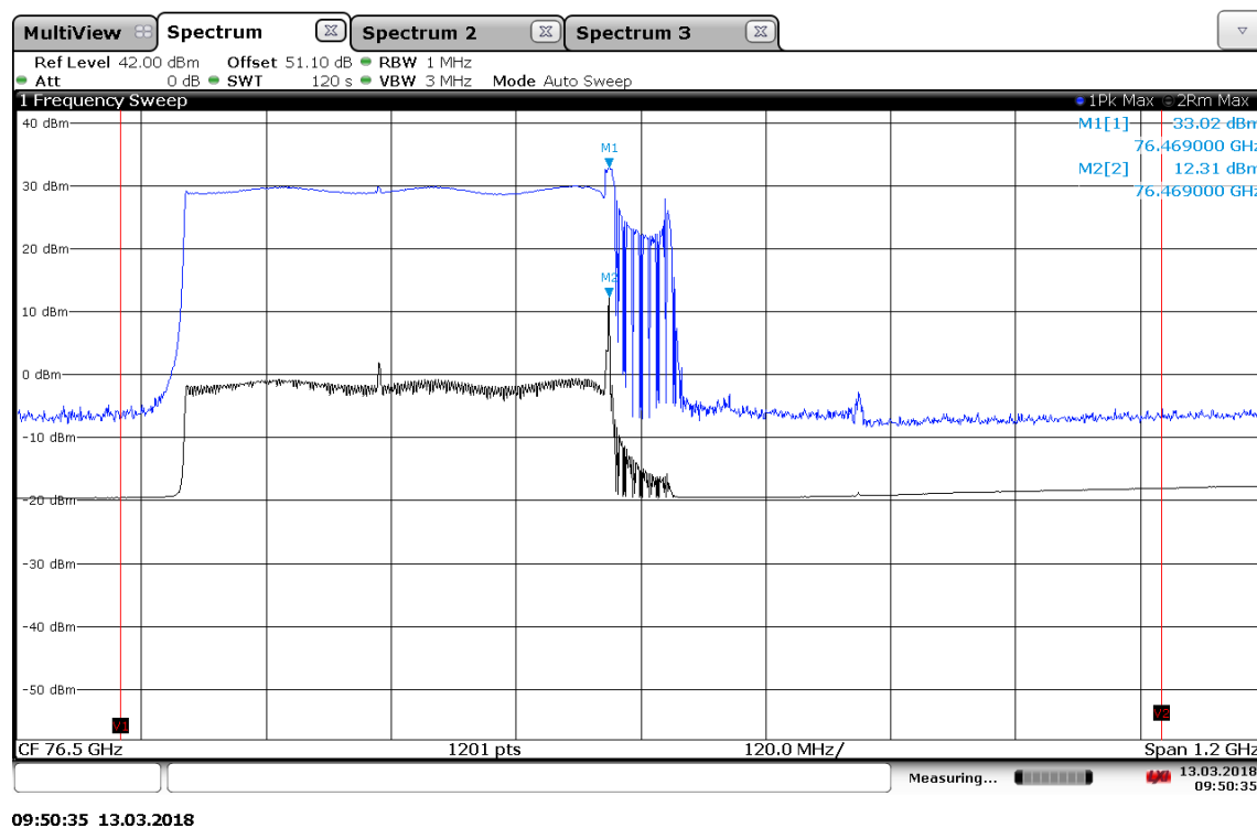
Plot 90: Mode 9, T_{nom} / V_{nom}
