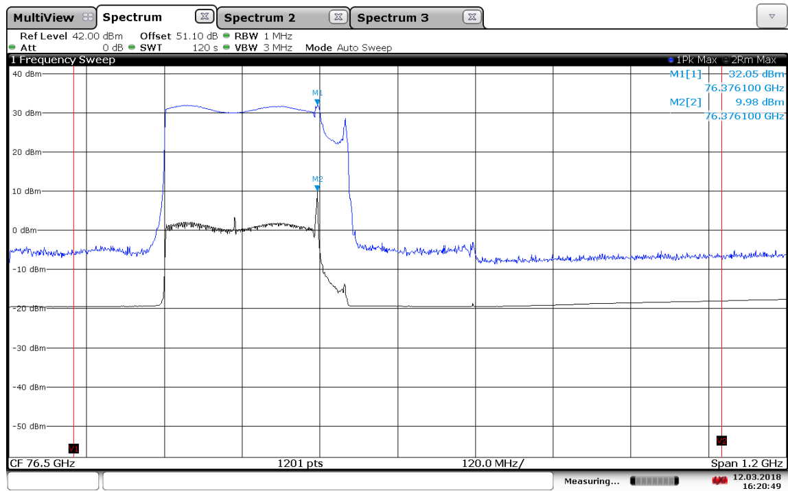
Plot 87: Mode 5, T_{nom} / V_{nom}
