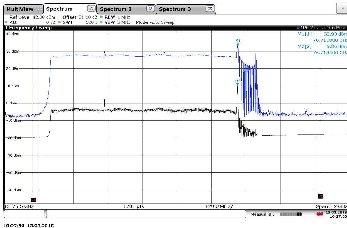
Plot 91: Mode 160, T_{nom} / V_{nom}
