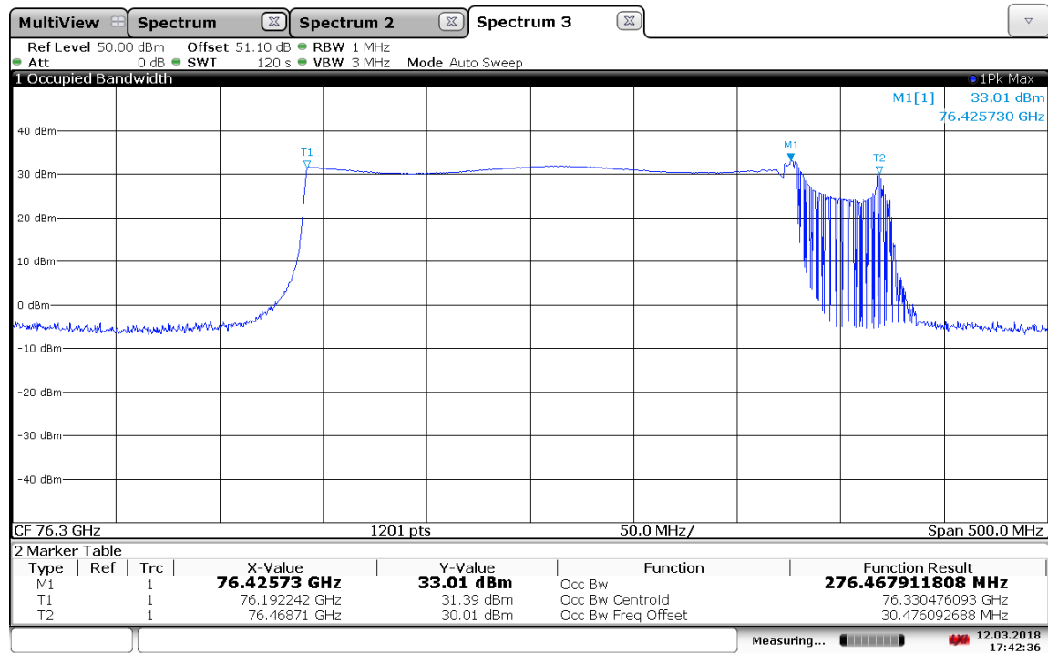
Plot 32: Mode 7, T_{\text{nom}} / V_{\text{nom}}
