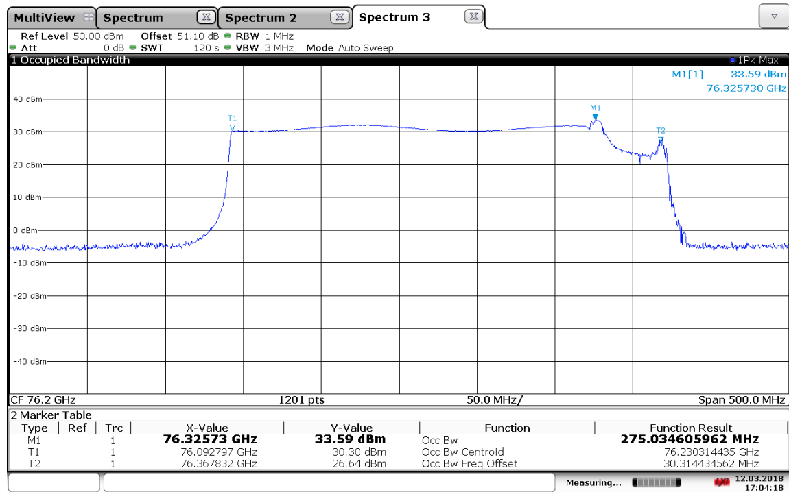
Plot 31: Mode 6, T_{\text{nom}} / V_{\text{nom}}
