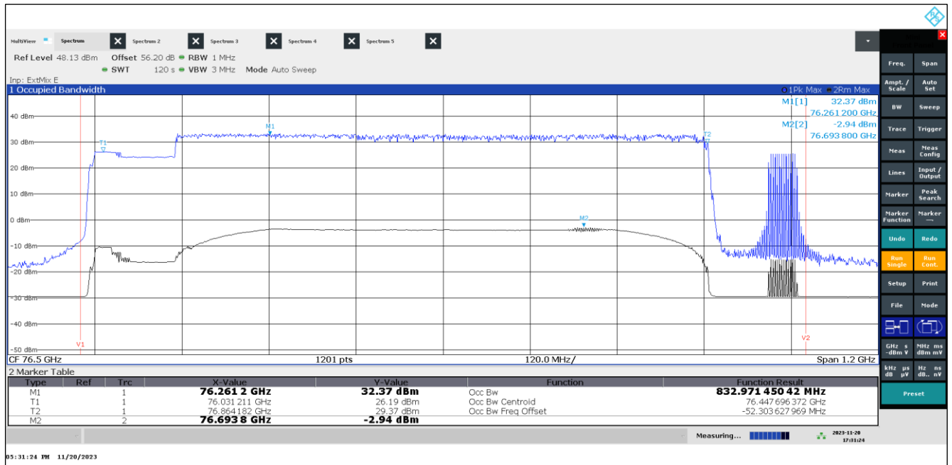
Plot 19: OBW, Mode 51, T_{\text{nom}} / V_{\text{min-max}}
