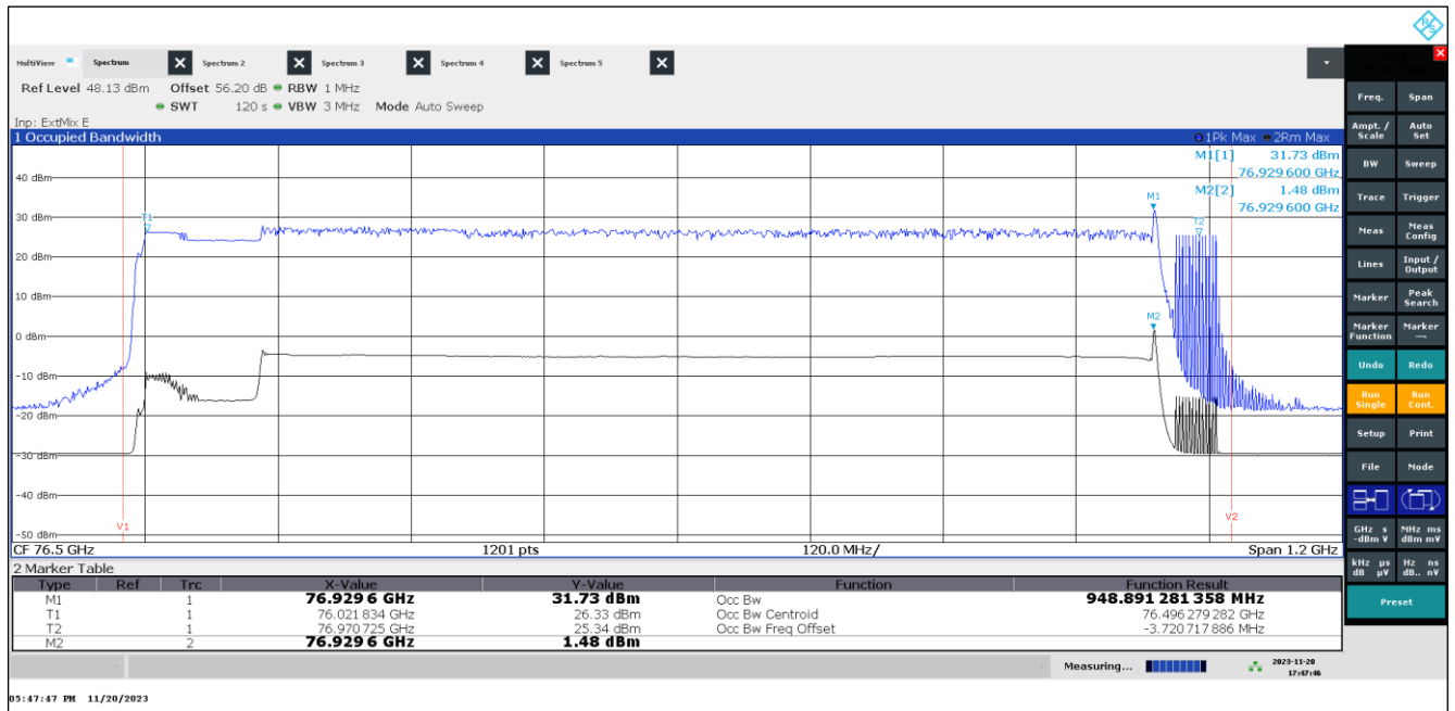
Plot 25: OBW, Mode 80, T_{\text{nom}} / V_{\text{min-max}}
