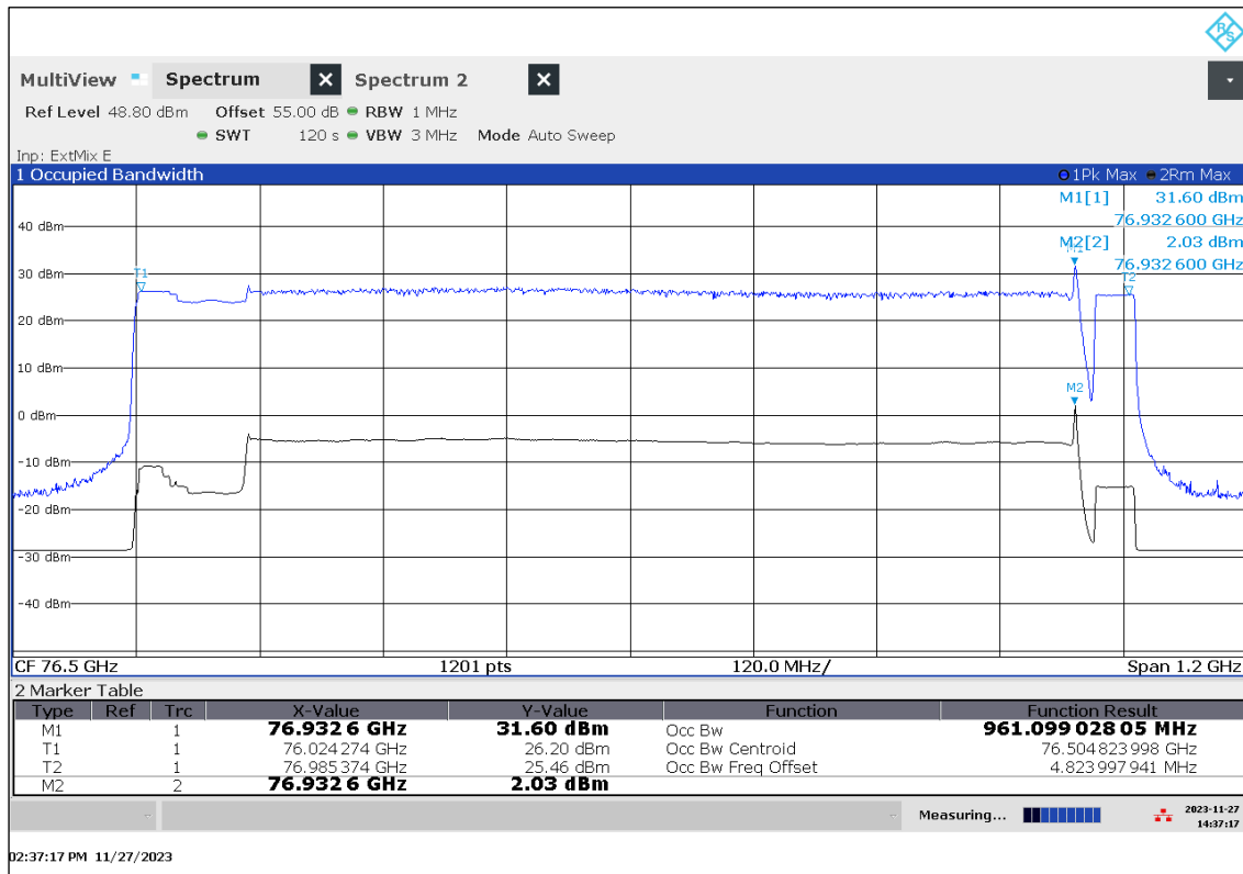
Plot 26: OBW, Mode 80, T_{\text{min}} / V_{\text{min-max}}
