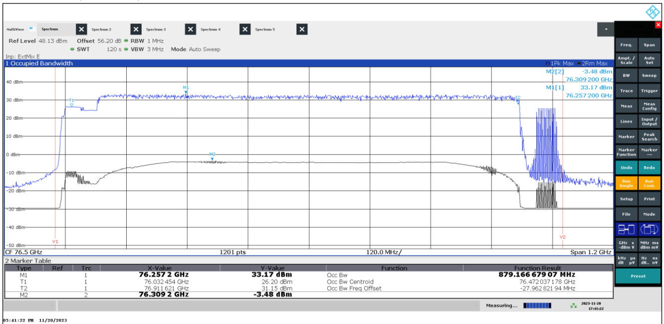
Plot 22: OBW, Mode 63, T_{\text{nom}} / V_{\min-\max}
