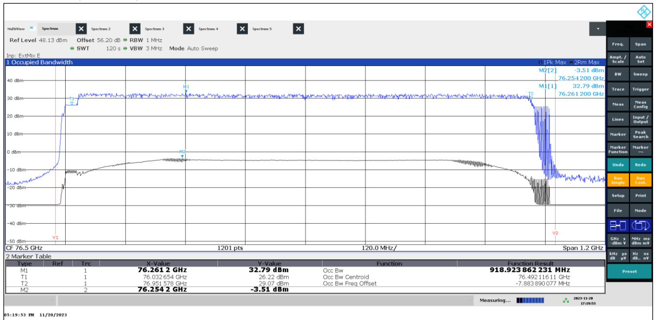
Plot 16: OBW, Mode 39, T_{\text{nom}} / V_{\min-\max}
