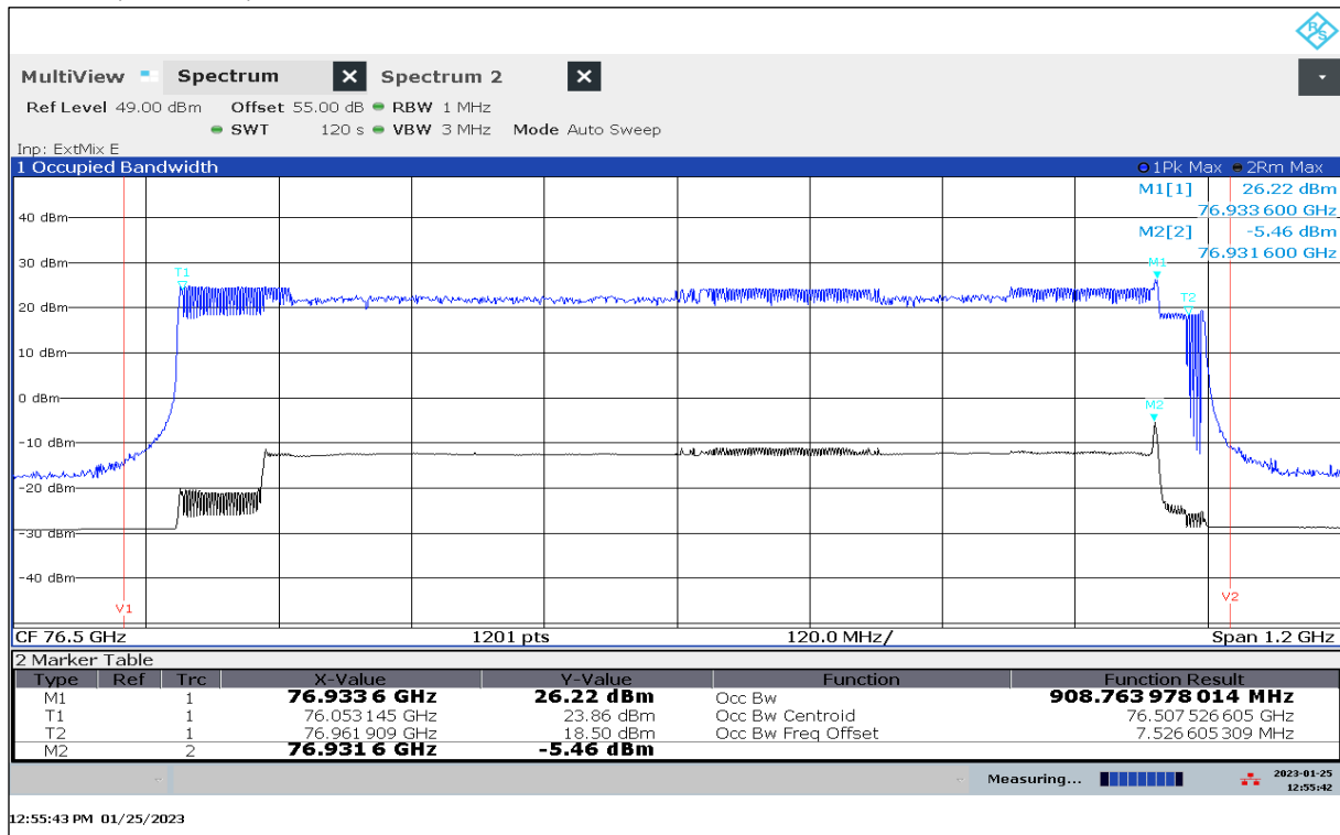
Plot 26: OBW, Mode 80, T_{\text{min}} / V_{\text{min-max}}
