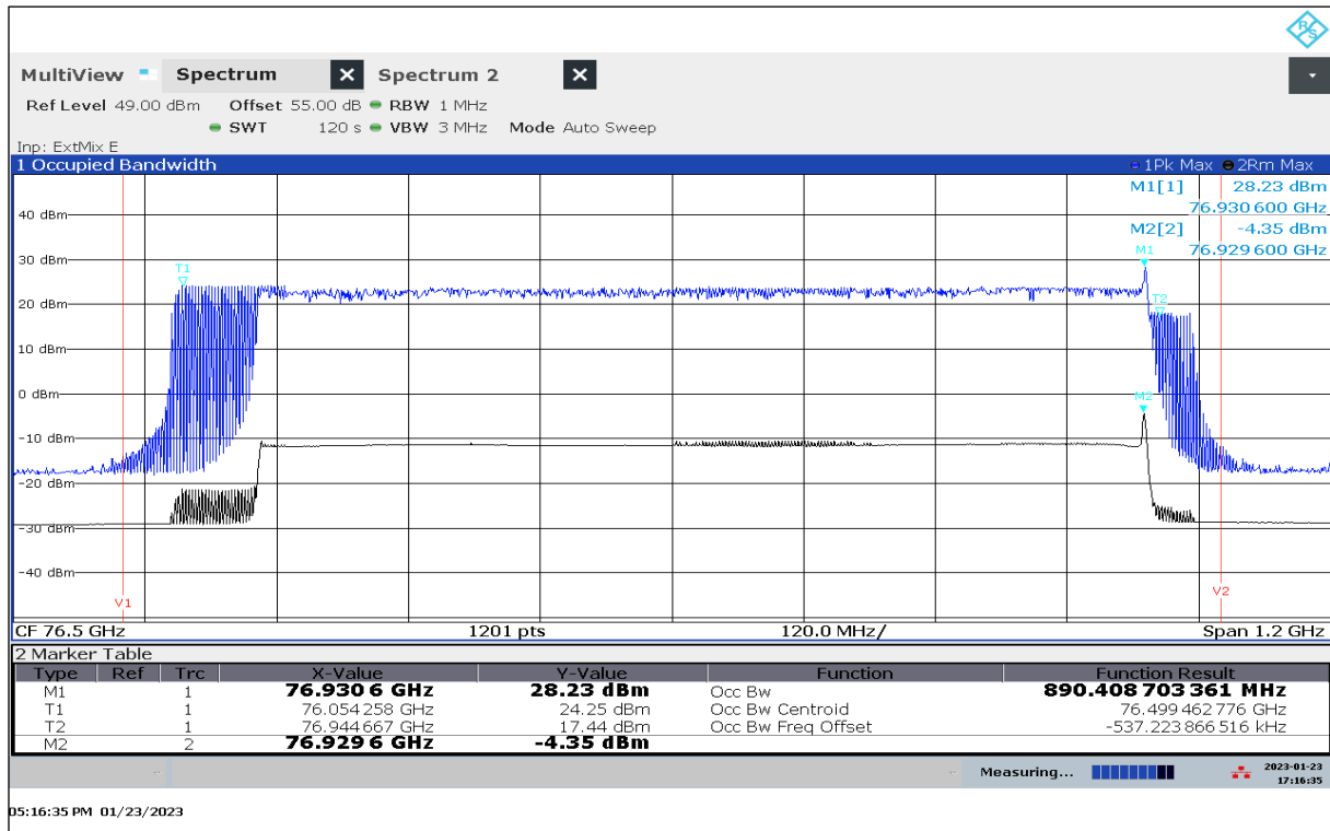
Plot 25: OBW, Mode 80, T_{\text{nom}} / V_{\text{min-max}}
