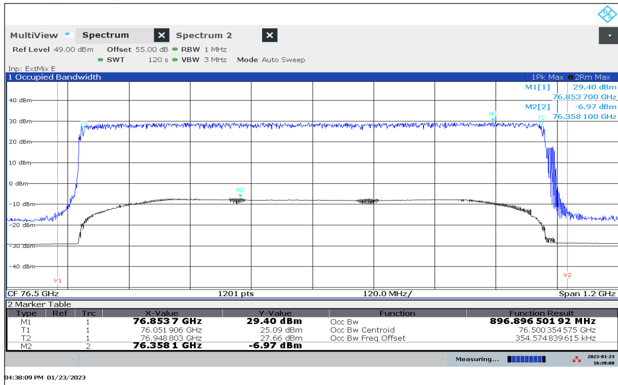
Plot 16: OBW, Mode 39, T_{\text{nom}} / V_{\min-\max}
