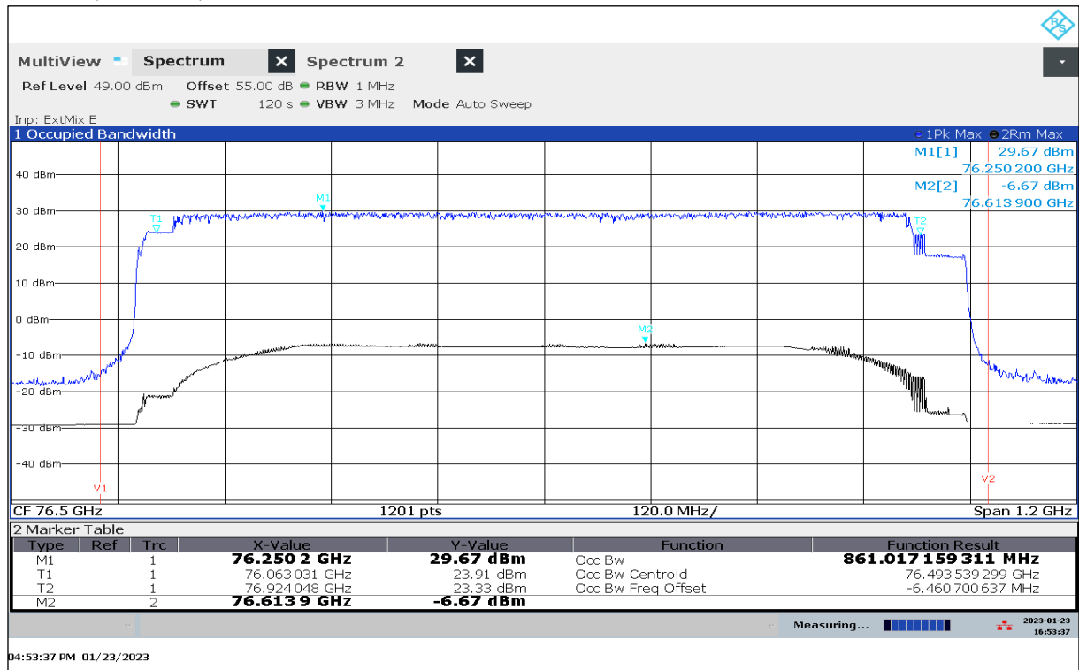
Plot 22: OBW, Mode 63, T_{\text{nom}} / V_{\min-\max}
