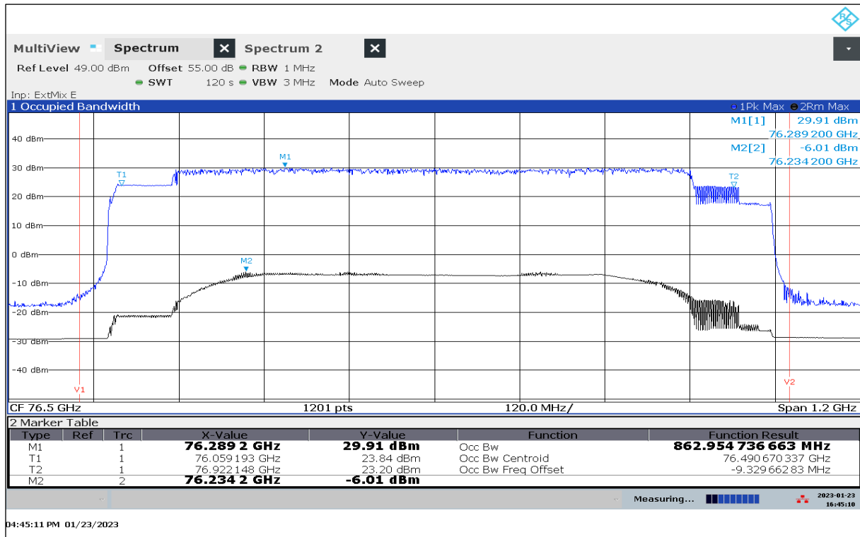
Plot 19: OBW, Mode 51, T_{\text{nom}} / V_{\text{min-max}}
