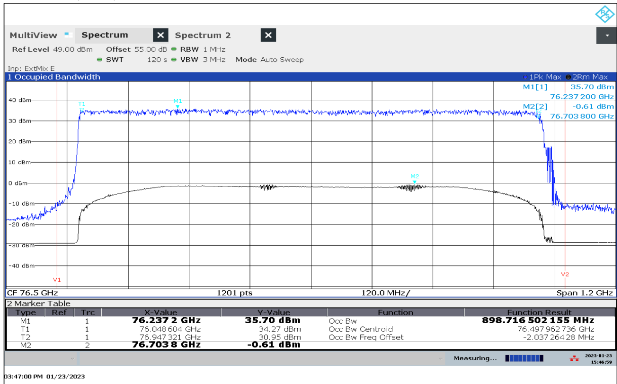
Plot 82: Mode 09, OBW, 20 °C / V min-max
