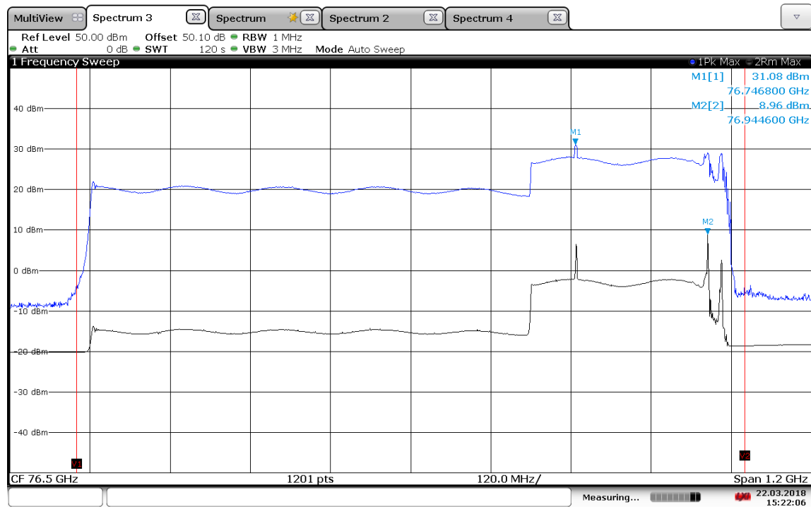
Plot 64: Mode 49, T_{\text{nom}} / V_{\text{nom}}
