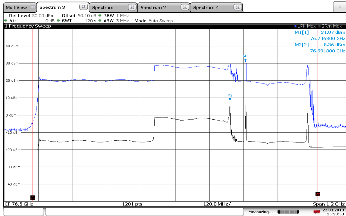
Plot 65: Mode 50, T_{\text{nom}} / V_{\text{nom}}
