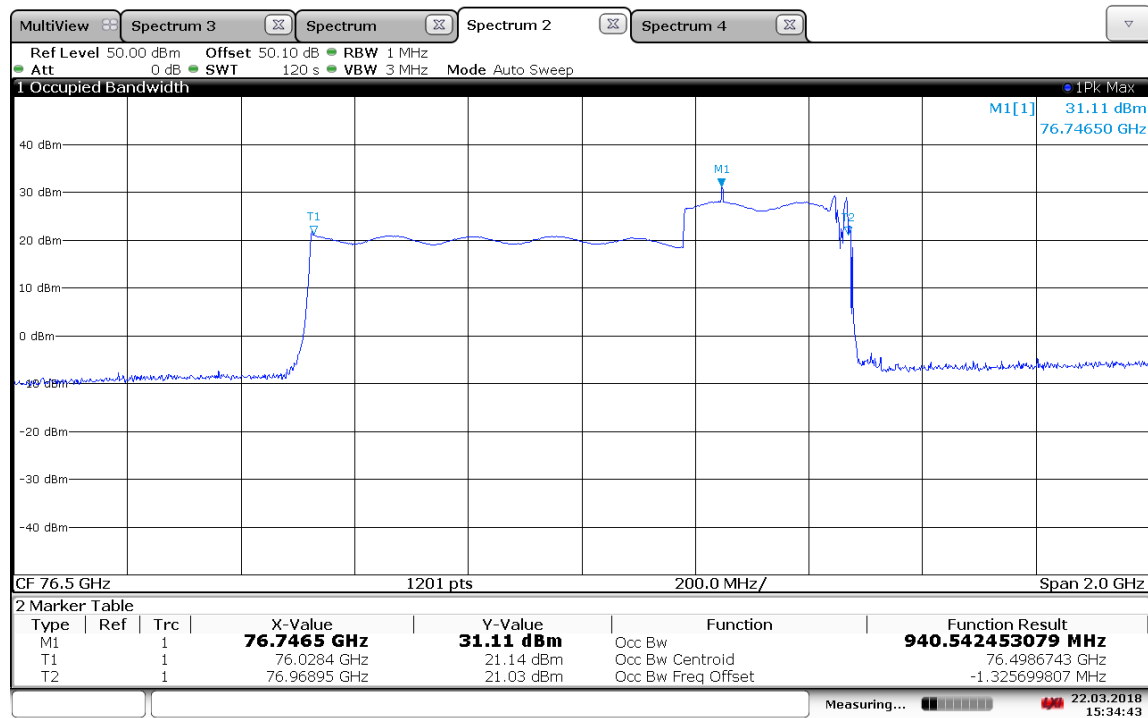
Plot 19: Mode 49, T_{\text{nom}} / V_{\text{nom}}
