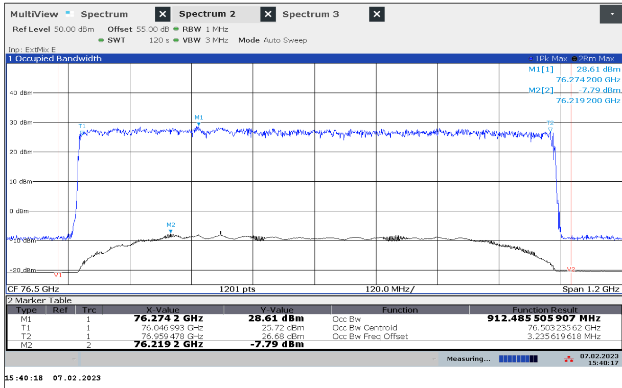
Plot 13: OBW, Mode 33, T_{\text{nom}} / V_{\text{min-max}}
