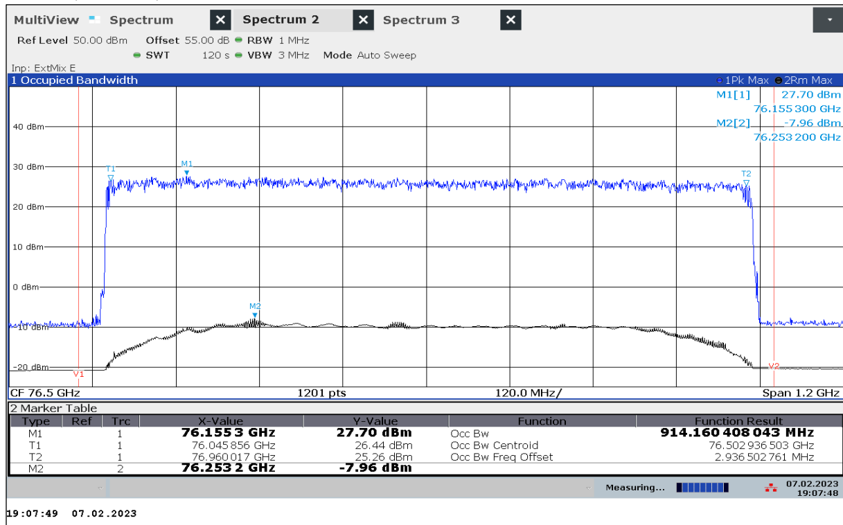
Plot 14: OBW, Mode 33, T_{\text{min}} / V_{\text{min-max}}
