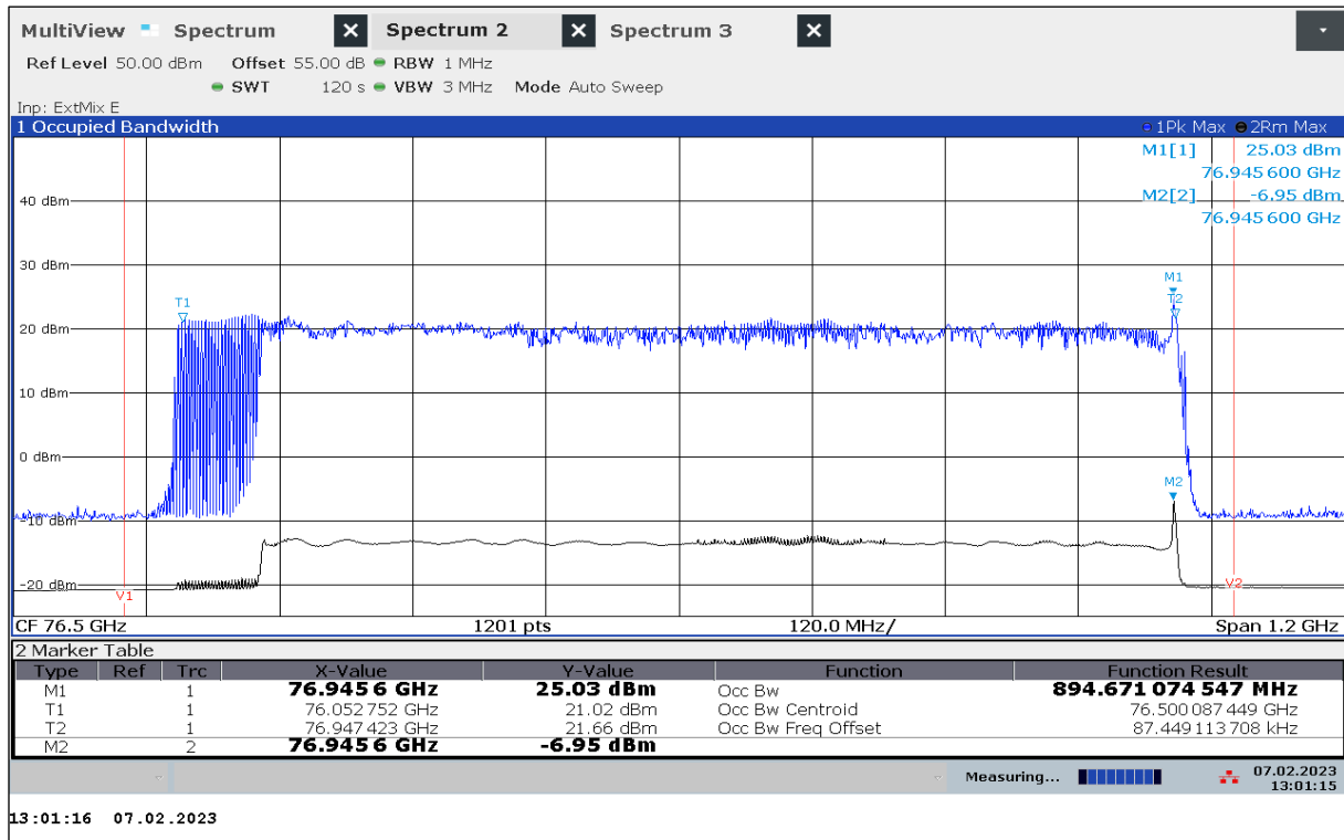
Plot 19: OBW, Mode 68, T_{\text{nom}} / V_{\text{min-max}}
