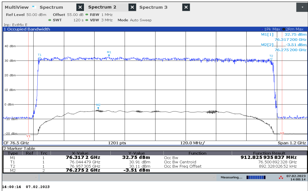
Plot 4: OBW, Mode 09, T_{\text{nom}} / V_{\min-\max}
