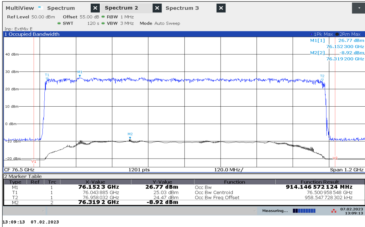
Plot 16: OBW, Mode 45, T_{\text{nom}} / V_{\min-\max}
