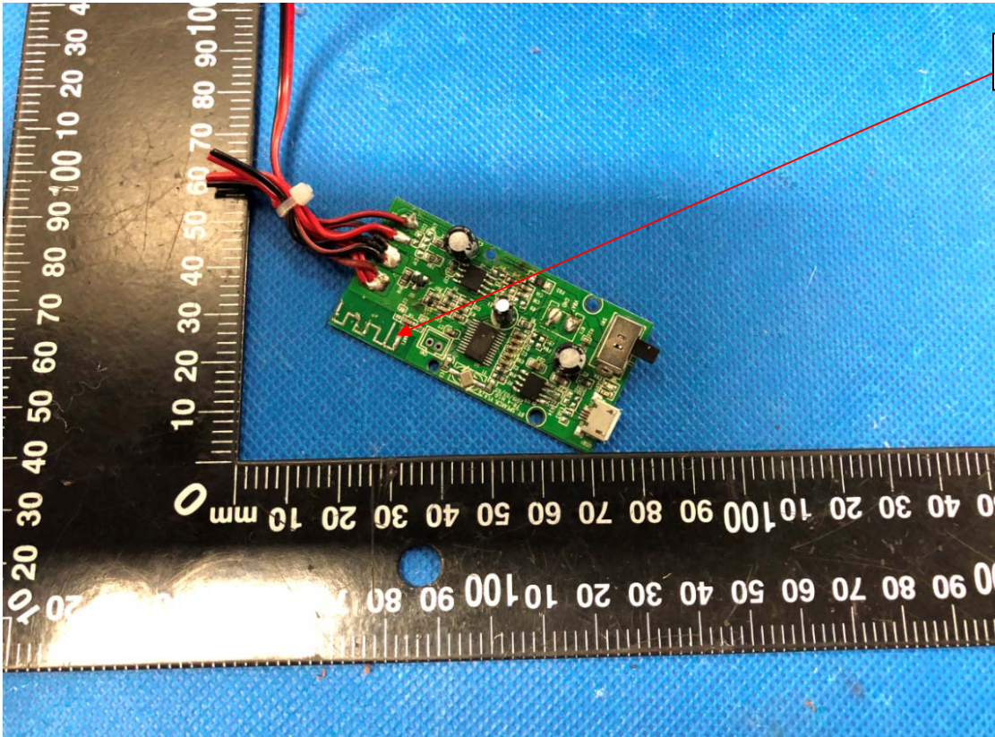
Antenna
