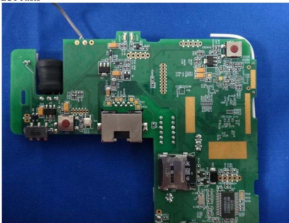
(18) EUT Photo
