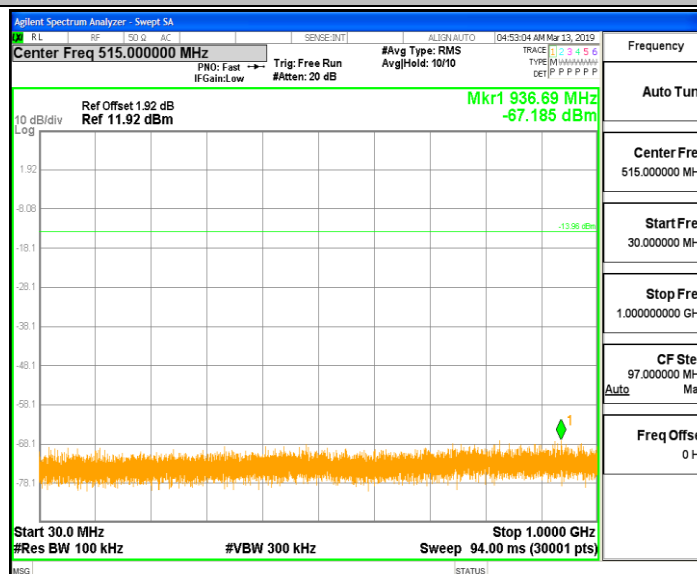
TX_Ant1_2442_30~1000
