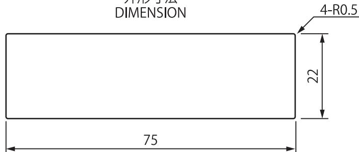
抜き型 CUTTING DIE
