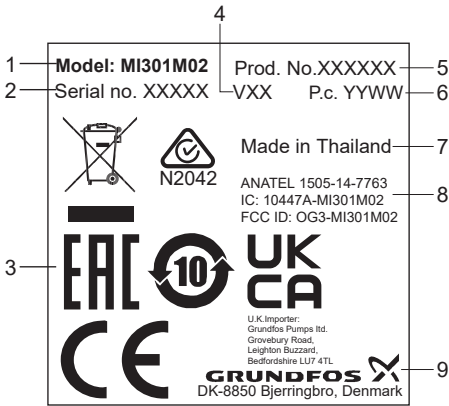
銘牌範例
