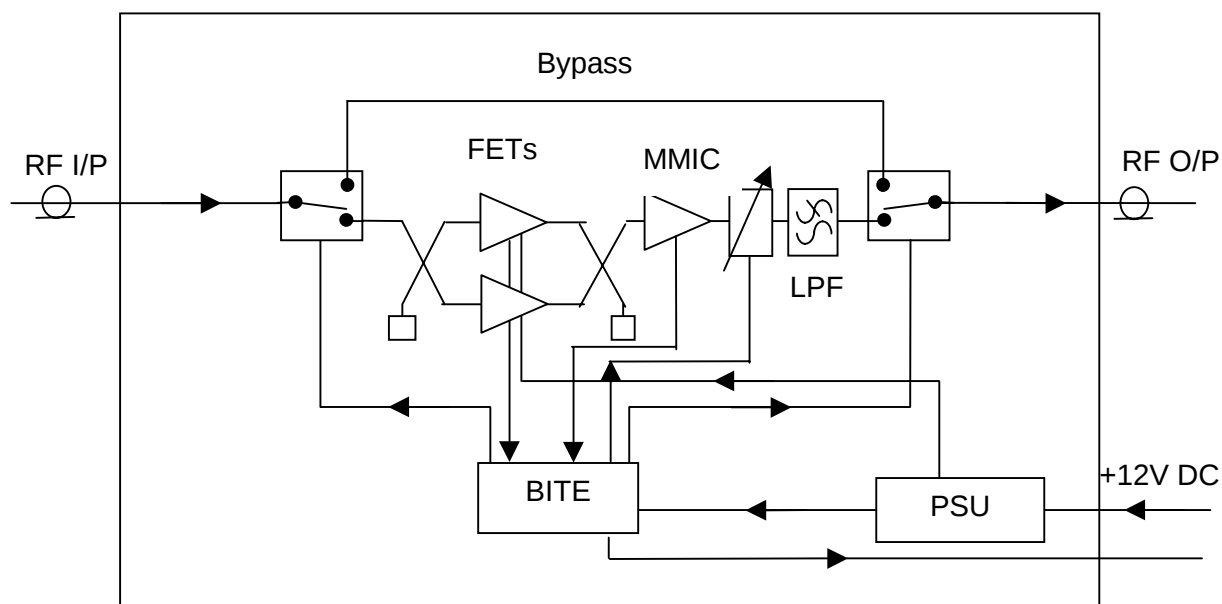
Figure 4 LNA Module
