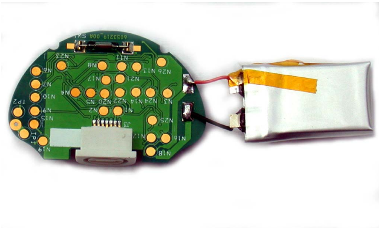
GST1 ( MMT7703) internal PCB : bottom
