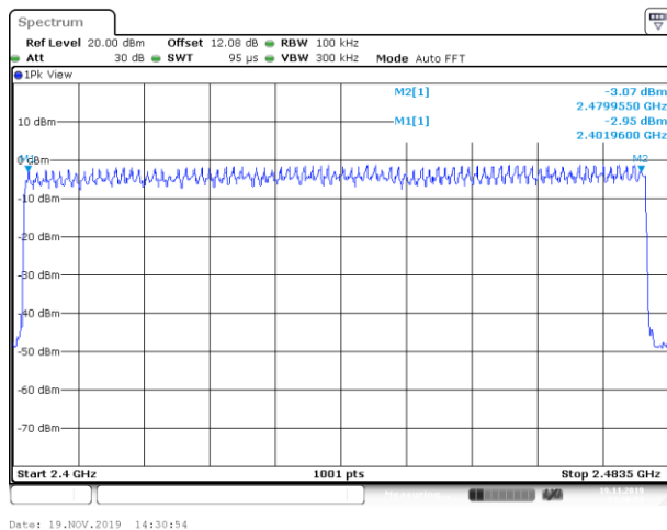
EDR-3Mbps mode
