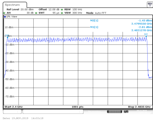
EDR-2Mbps mode
