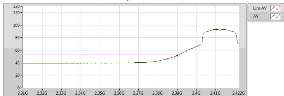
RE above 1GHz;Band:2.4G;11g;BWch:20MHz;Nss:1;Nant:1;Ch:2412MHz;TX
