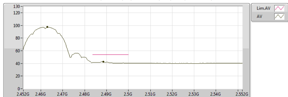
RE above 1GHz;Band:2.4G;11b;BWch:20MHz;Nss:1;Nant:1;Ch:2462MHz;TX
