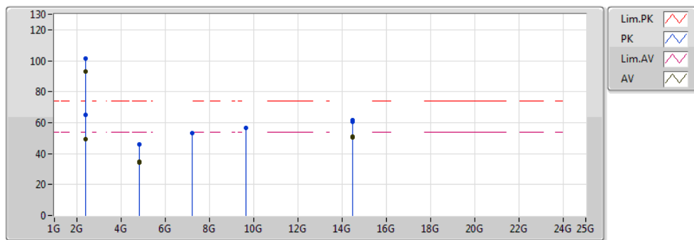
RE above 1GHz;Band:2.4G;HT20;BWch:20MHz;Nss:1,(M0-7);Nant:1;Ch:2412MHz;TX
