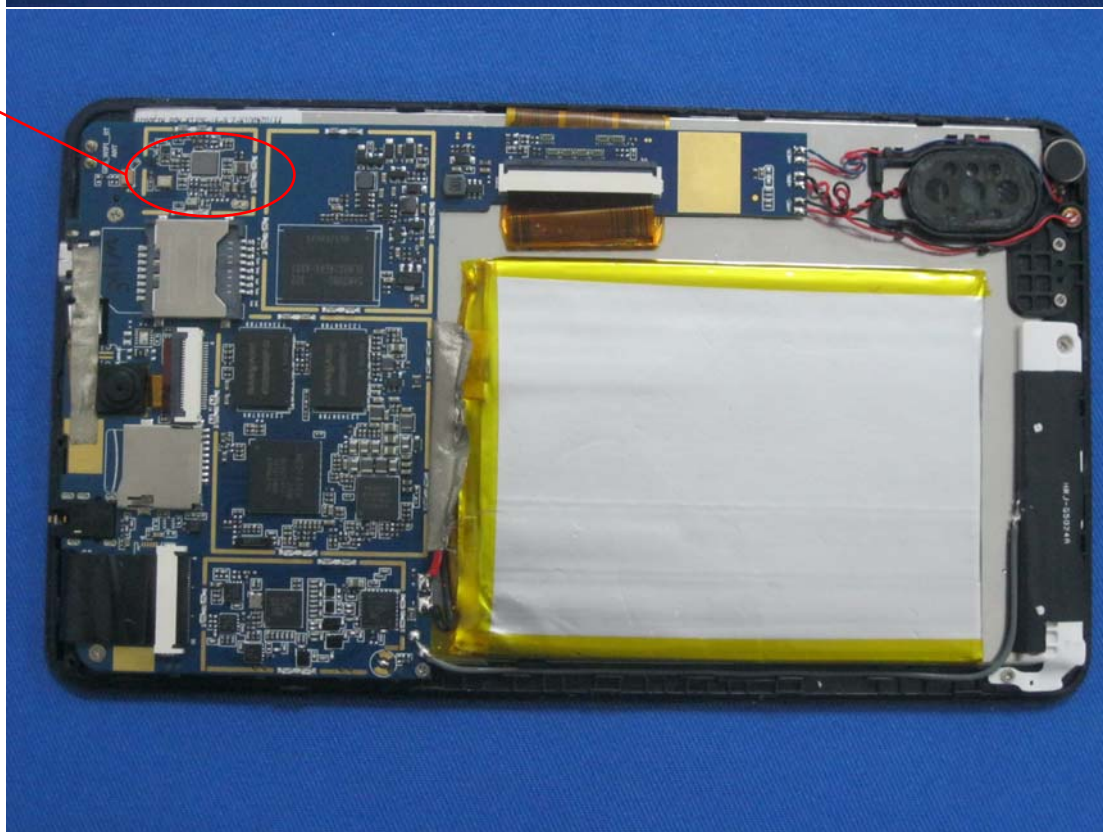
WIFI/BT module OSC: 26 MHz
